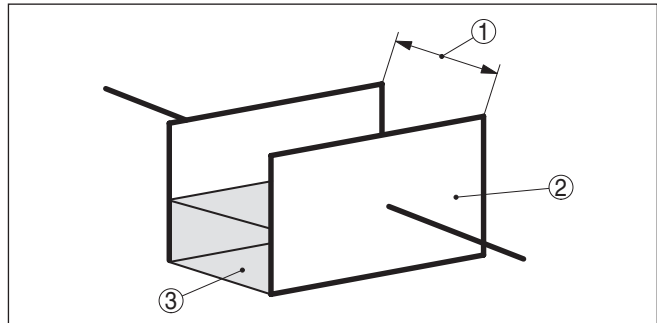
Abb. 2: Funktionsprinzip - Plattenkondensator
