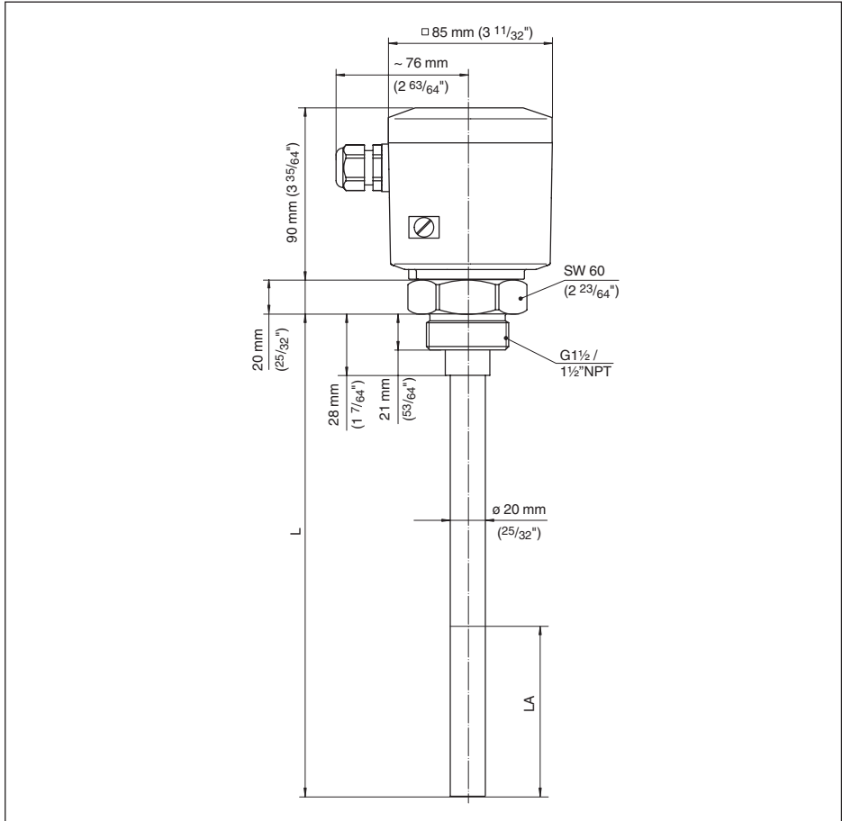
Abb. 10: VEGACAP 27, Gewindeausführung G1½ (ISO 228 T1)
