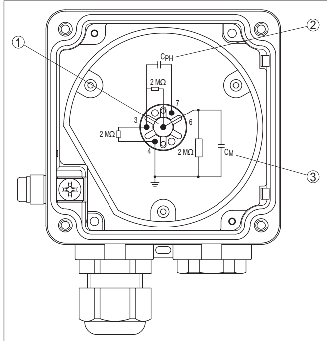
Fig. 21: Weerstand binnen de sensor controleren
