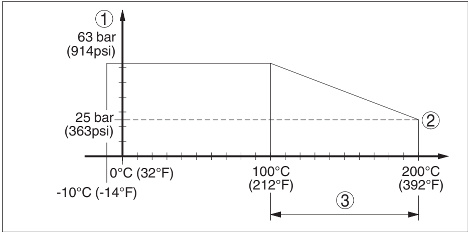
Fig. 22: Procesdruk - procestemperatuur - VEGACAP 27 met procesaansluiting van 316L
