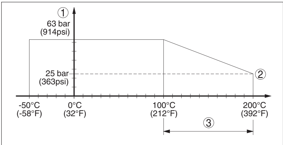
Fig. 23: Procesdruk - procestemperatuur - VEGACAP 27 met procesaansluiting van 316Ti
