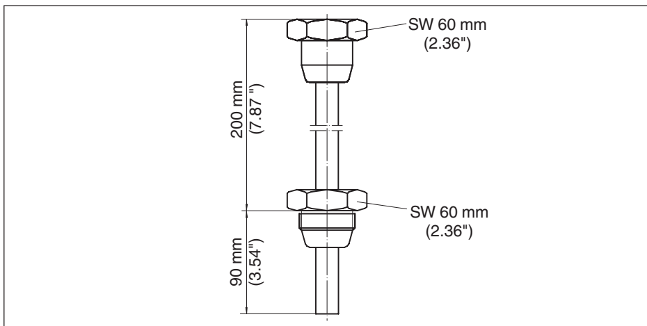
Fig. 25: Temperatuurtussenstuk (optie) 316L, 316Ti
