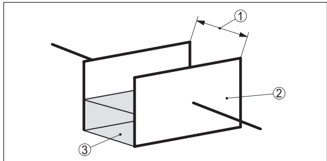
Fig. 2: Werkingsprincipe - plaatcondensator
