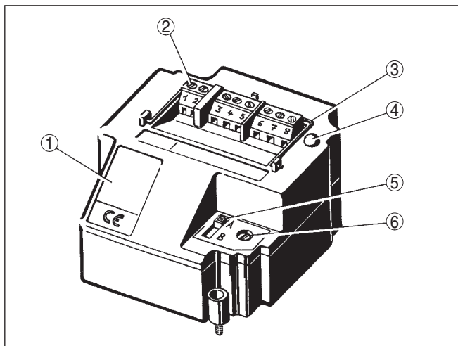
插图. 6: 带继电器输出电子的插件
