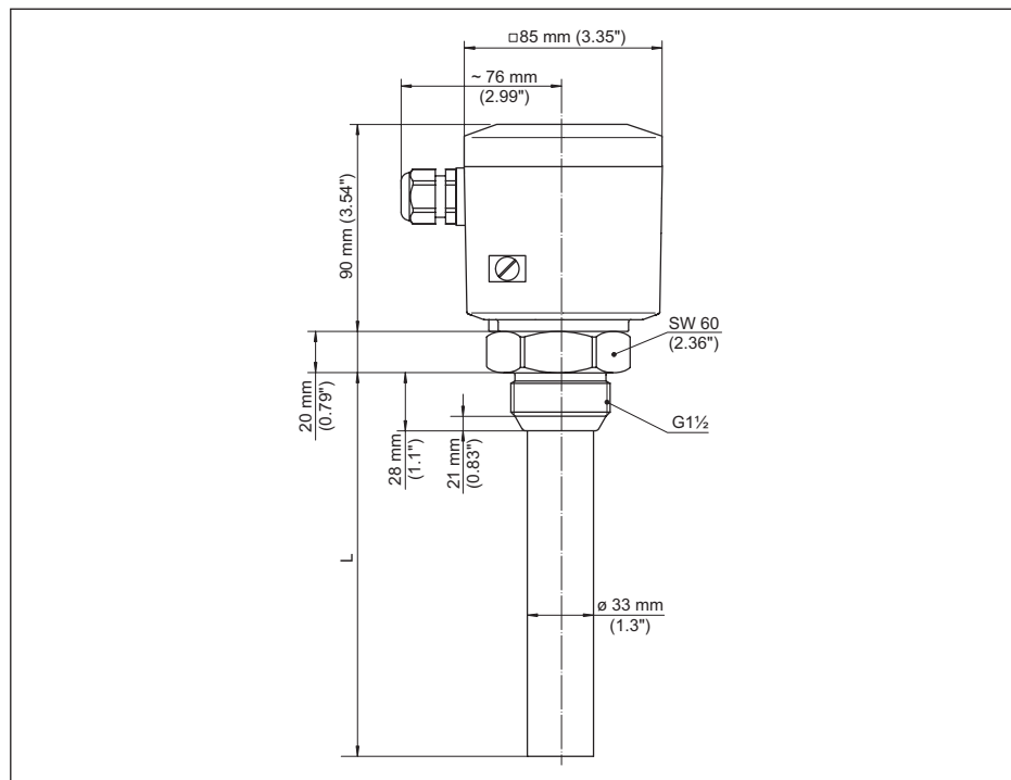
插图 8: VEGACAP 98, G1 A (ISO 228 T1) 螺纹型
