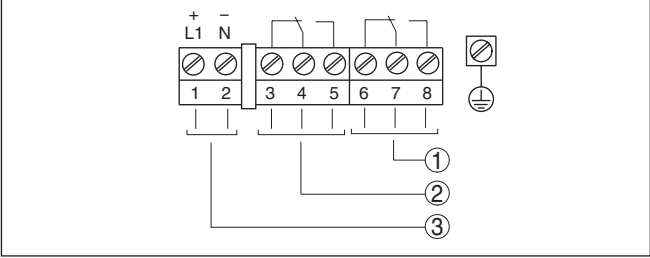
插图 5: 接线图
