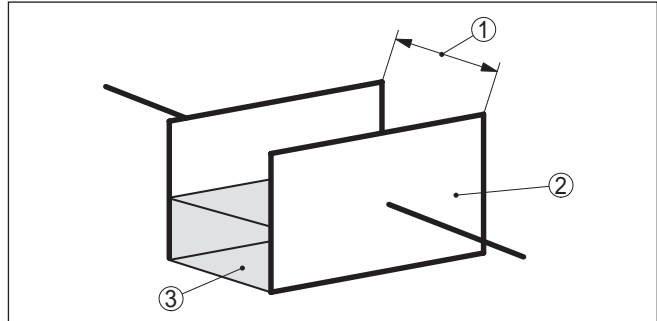
Fig. 2: Werkingsprincipe - plaatcondensator
