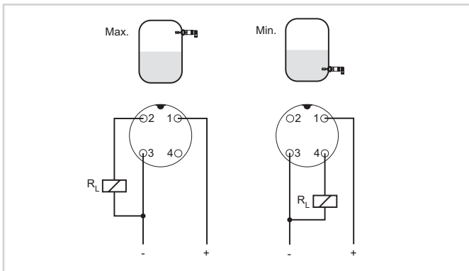
VEGASWING 51 avec connecteur à fiches M12 x 1
