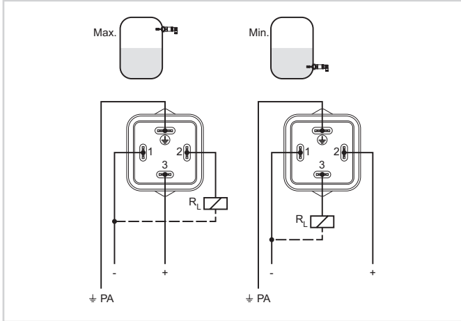
VEGASWING 51 avec connecteur type électrovanne ISO 4400
