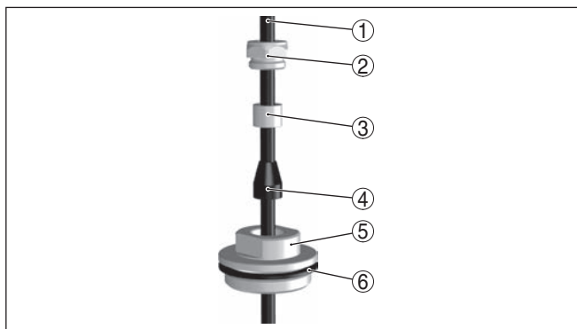
插图. 7: 便携式电缆螺纹连接件的构造
