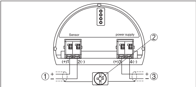
插图. 13: 用于 4 ... 20 mA 传感器的 VEGAWELL 52 的接线图 1 通往传感器 2 用于连接电缆屏蔽的端子 3 用于供电
