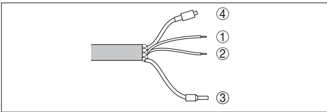
插图. 10: 便携式电缆的芯线分布 1 蓝色 (-): 用于供电或通往分析系统 2 棕色 (+): 用于供电或通往分析系统 3 屏蔽 4 带有过滤元件的压力补偿壳体
