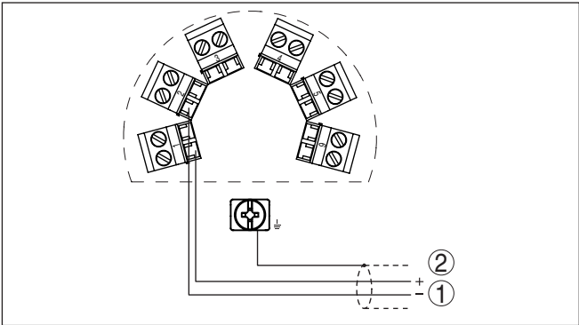
插图. 12: 壳体接线图 1 通往供电装置或通往分析系统
