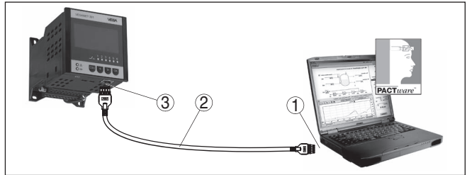
插图. 9: 通过以太网与电脑相连接
