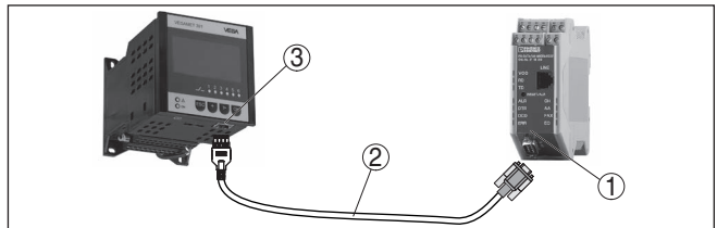
插图. 10: 通过 RS232 连接调制解调器
