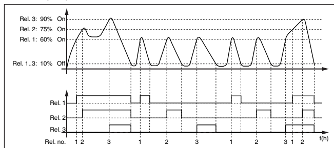
Fig. 17: Ejemplo de control de bomba 4
