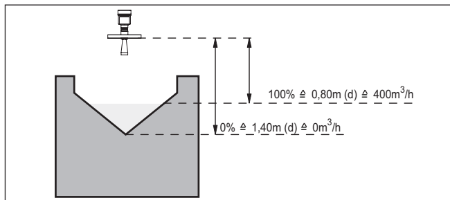
Fig. 21: Ajuste medición de flujo con aliviadero triangular
