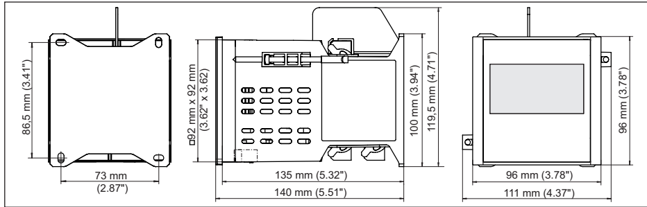
Fig. 23: Medidas VEGAMET 391
