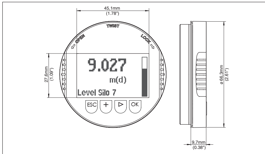
Figura 12: Dimensioni del tastierino di taratura con display
