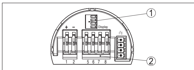
Figura 6: Interfacce per indicazione e calibrazione
