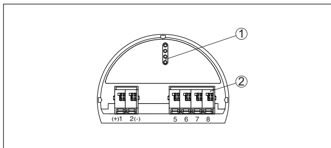
Figura 7: Interfacce per indicazione e calibrazione
