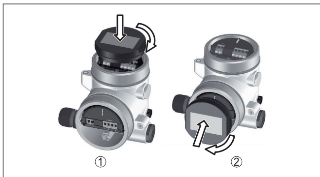
Figura 4: Inserimento del tastierino di taratura con display in caso di custodia a due camere
