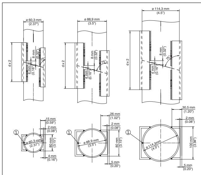
插图. 19: 在用于不同直径的波峰管延长件上进行焊接连接
