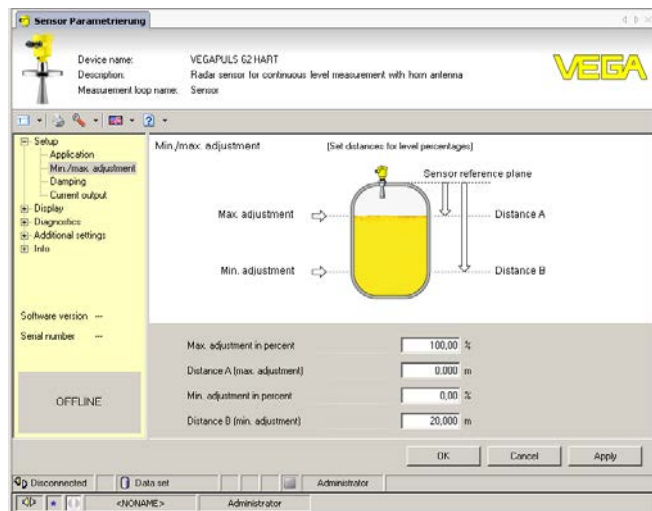
插图. 41: DTM 视图举例
