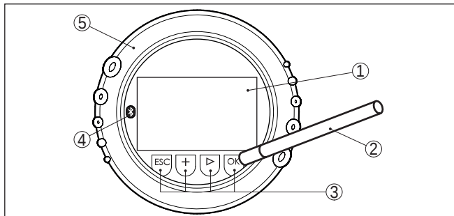
插图. 37: 显示和调整元件 - 拥有磁笔操作功能
