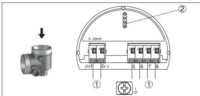
插图. 25: 双腔式壳体的电子部件腔
