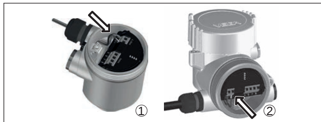
插图. 23: 接线步骤5和6
