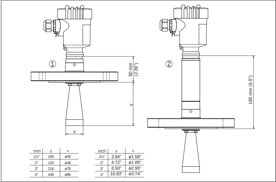
插图. 65: VEGAPULS 62，号角天线，法兰型
