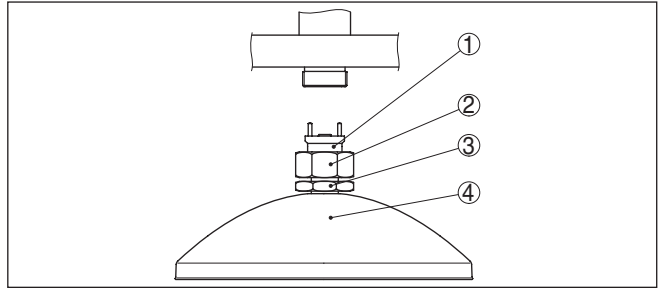
插图. 3: 抛物形天线的拆卸
