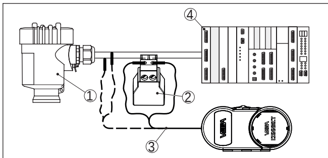
插图. 40: 通过 HART 将电脑与信号线路相连
