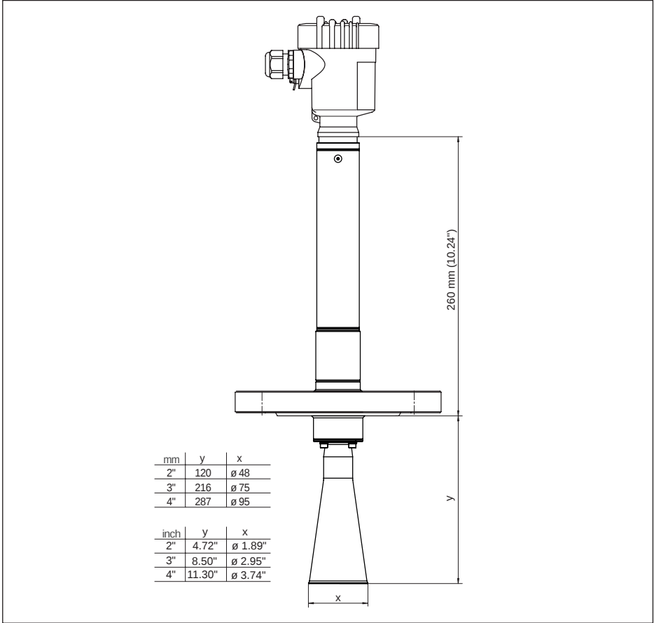
插图. 67: VEGAPULS 62, 法兰型号角天线，带有至 450 °C 的温度连接元件
