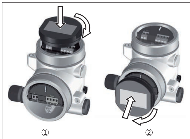
插图. 35: 将显示和调整模块装到双腔式壳体上
