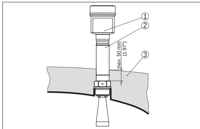
插图. 17: 将仪表安装在绝缘容器上。
