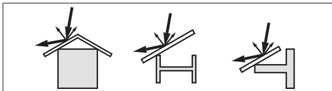
插图. 15: 用散射挡板来覆盖光滑的型材
