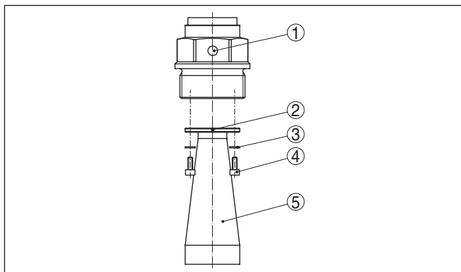
插图. 2: 号角天线的拆卸
