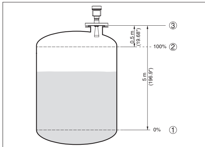
插图. 38: 有关最小/最大调整的参数化举例
