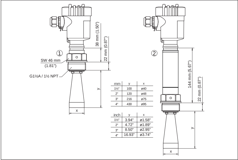
插图. 64: VEGAPULS 62, 号角天线，螺纹型
