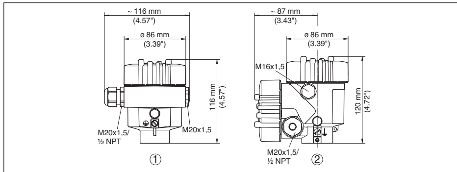
插图. 60: 采用保护等级达 IP 66/IP 68 (0.2 bar) 的壳体型式 (内装显示和调整模块后, 壳体高度增加了 18 mm/0.71 in)
