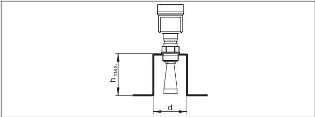
插图. 12: 管接头尺寸有偏差
