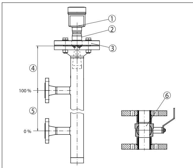
插图. 20: 旁路的构造
