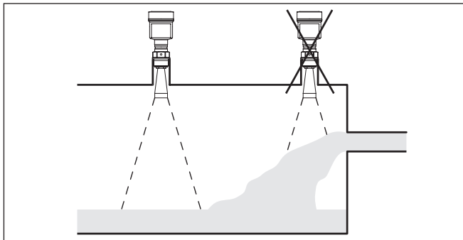
插图. 7: 流入介质时安装雷达传感器
