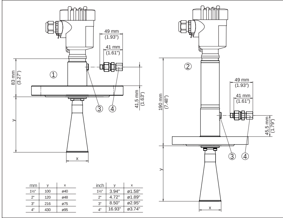
插图. 66: VEGAPULS 62, 带有吹气接口的法兰型号角天线
