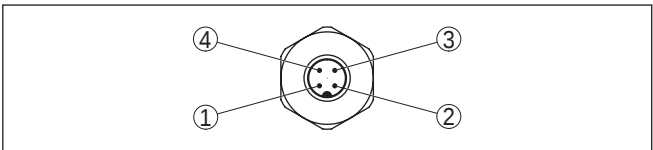
插图. 32: 目检连接插头 M12 x 1
