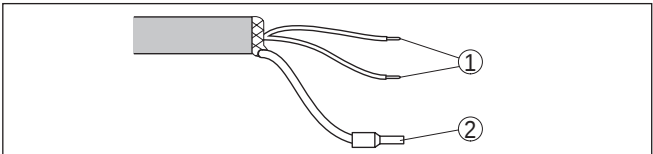
插图. 33: 固定连接的连接电缆的芯线分布
