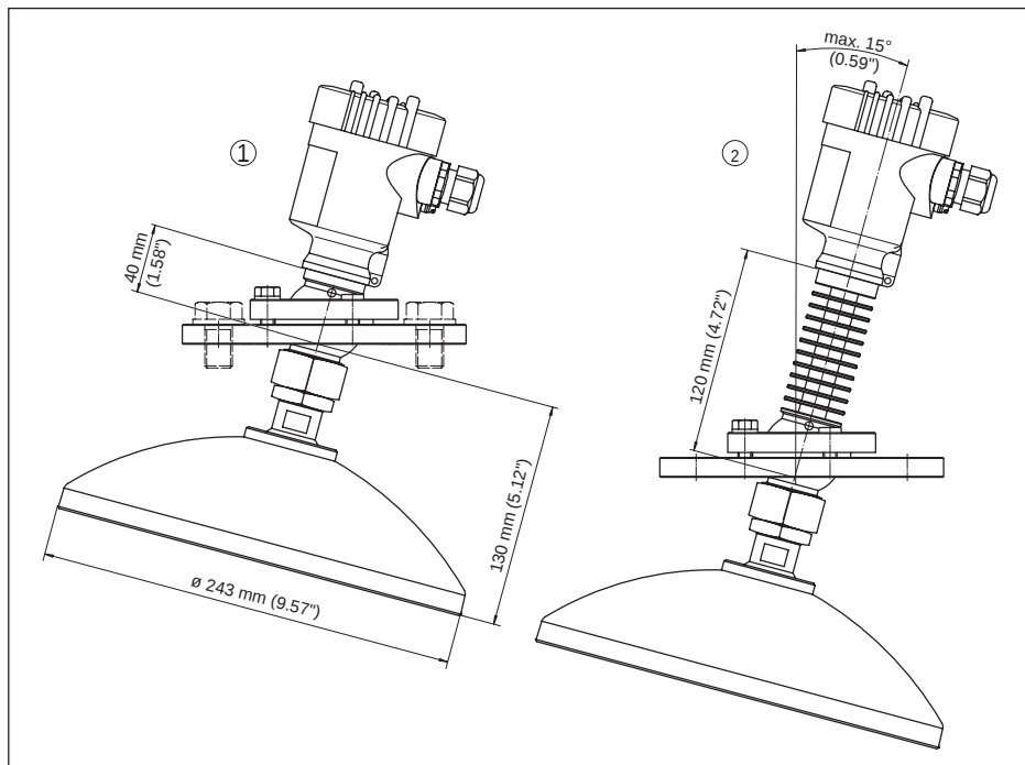
插图. 70: VEGAPULS 62, 抛物形天线和转动支架
