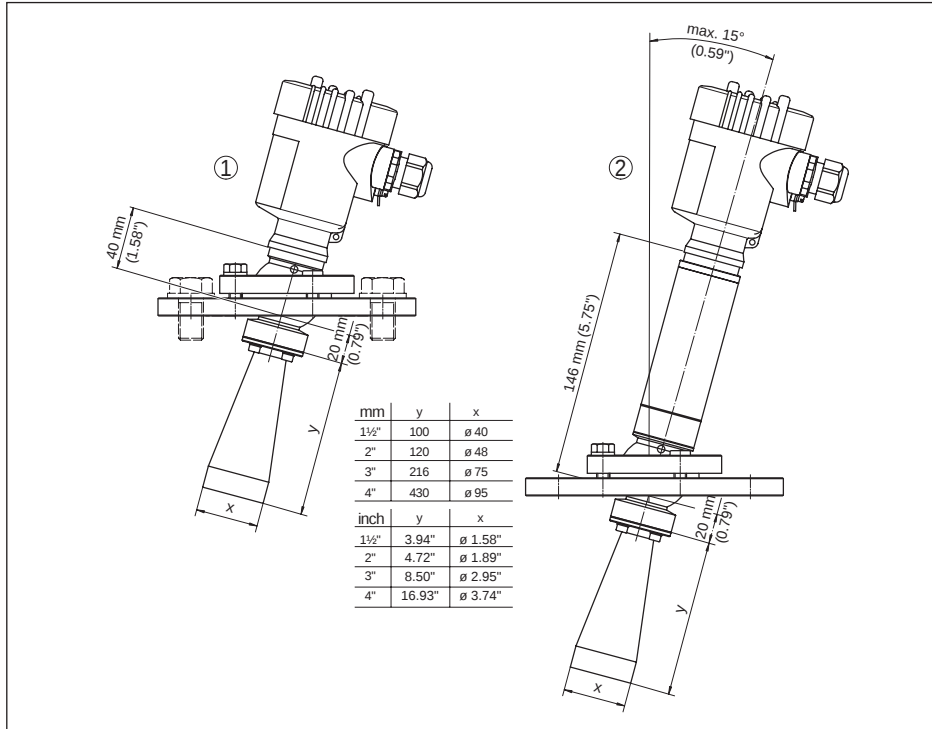
插图. 68: VEGAPULS 62, 号角天线和转动支架
