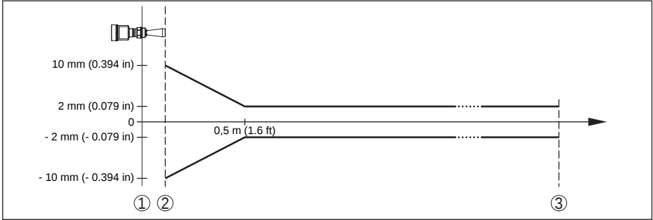
插图: 58: 在基准条件下的测量偏差
