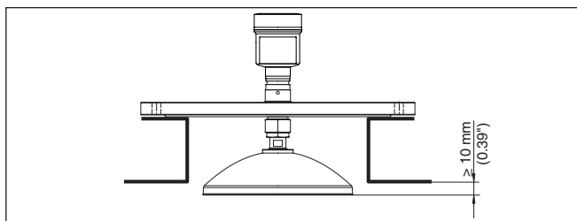
插图. 9: 抛物形天线上推荐的管接头安装方式
