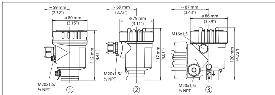
插图. 62: 采用保护等级达 IP 66/IP 68 (0.2 bar) 的壳体型式 (内装显示和调整模块后, 壳体高度增加了18 mm/0.71 in)
