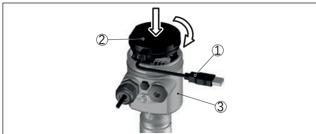
插图. 39: 通过接口适配器将电脑直接与传感器相连
