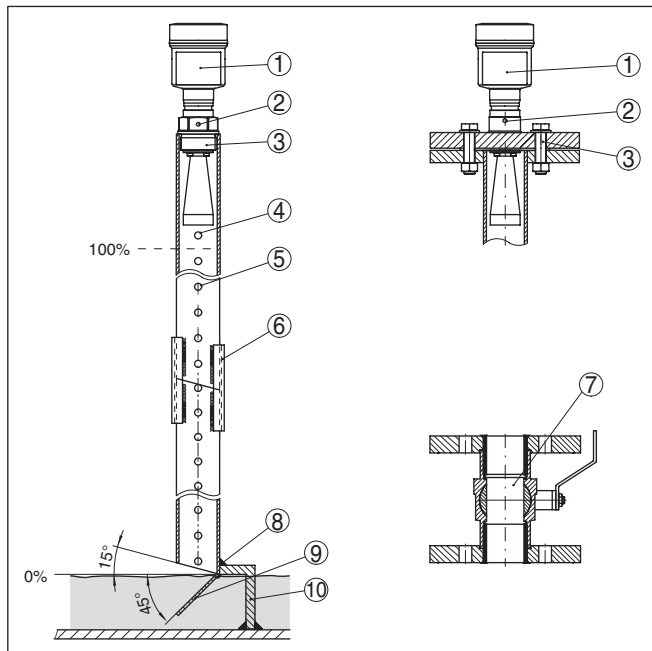
插图. 18: 波峰管的构造 VEGAPULS 62
