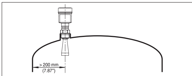
插图. 5: 将雷达传感器安装在圆形容器盖上
