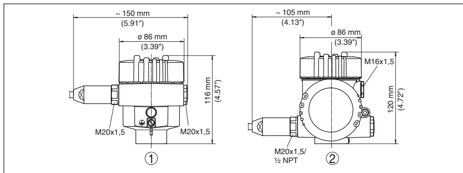
插图. 61: 采用保护等级达 IP 66/IP 68 (1 bar) 的壳体型式 (内装显示和调整模块后, 壳体高度增加了 18 mm/0.71 in)
