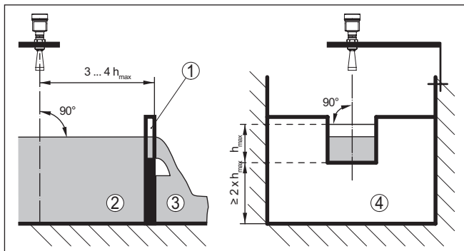
插图. 21: 利用矩形水道来测量流量: d_{\text{最小}} = 传感器的最小间距 (参见“技术参数”一章); h_{\text{最大}} = 矩形水道的最大充填量
