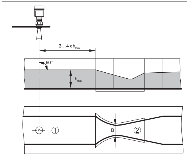
插图. 22: 用卡发基-文丘里水槽来测量流量: h_{max} = 水槽的最大灌装量; B = 水槽的最大收缩率
