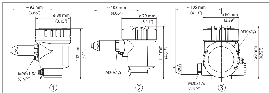
插图. 63: 采用保护等级达 IP 66/IP 68 (1 bar) 的壳体型式 (内装显示和调整模块后, 壳体高度增加了18 mm/0.71 in)
