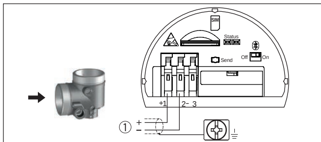
插图. 27: 接线腔 - 无线模块 PLICSMOBILE 81
