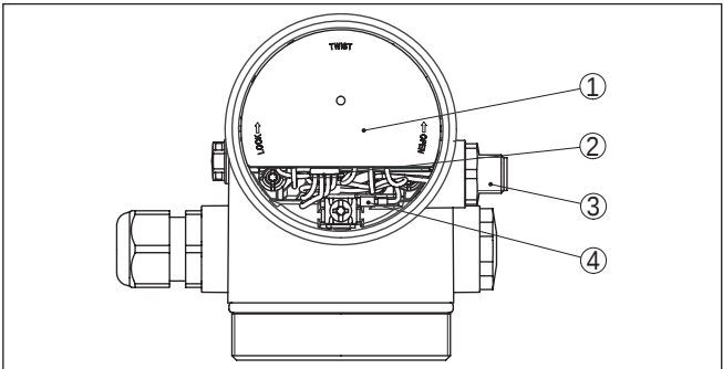
插图. 31: 目检带有与外部显示和调整单元相连接的 VEGADIS-Adapter 的电子部件腔
