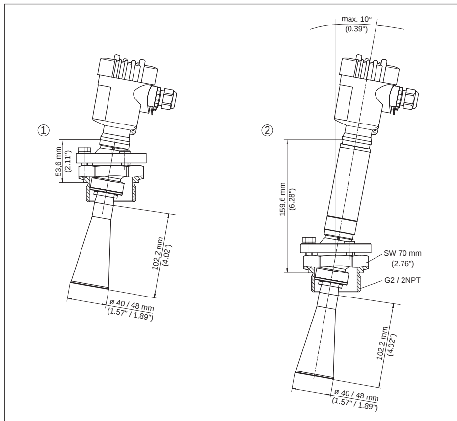
插图. 69: VEGAPULS 62, 号角天线和转动支架, 螺纹接头
