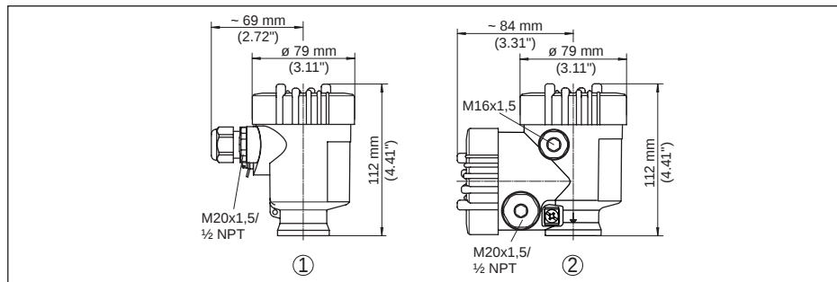
插图. 59: 采用保护方式为 IP 66/IP 67 的外壳型式 (内装显示和调整模块后, 外壳高度增加了 9 mm/0.35 in)
