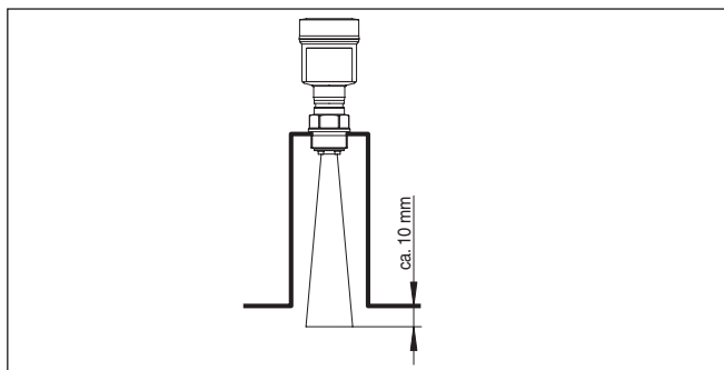
插图. 8: 号角天线上推荐的管接头安装方式
