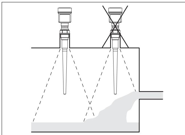
Fig. 6: Montage van de radarsensor bij instromend product
