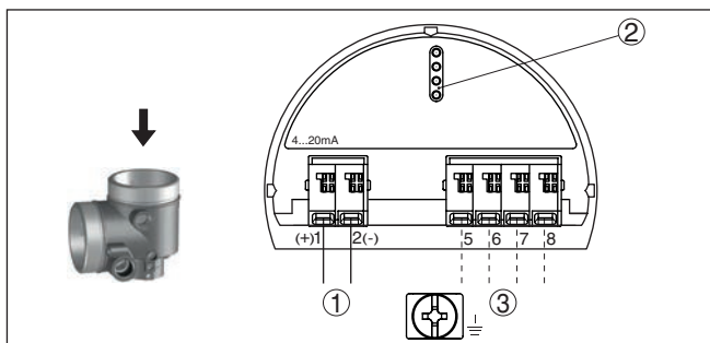
Fig. 16: Elektronicaruimte - Ex-ia-tweekamerbehuizing
