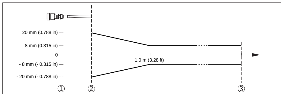
Fig. 46: Meetnauwkeurigheid onder referentiecondities
