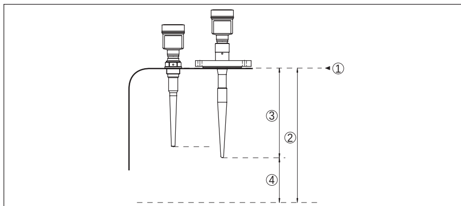
Fig. 45: Data betreffende ingangsgrootte
