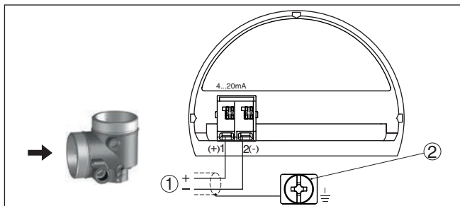
Fig. 17: Aansluitruimte - Ex-d-ia-tweekamerbehuizing
