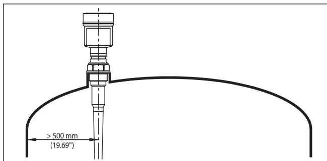
Fig. 4: Montage van de radarsensor op ronde tankdaken
