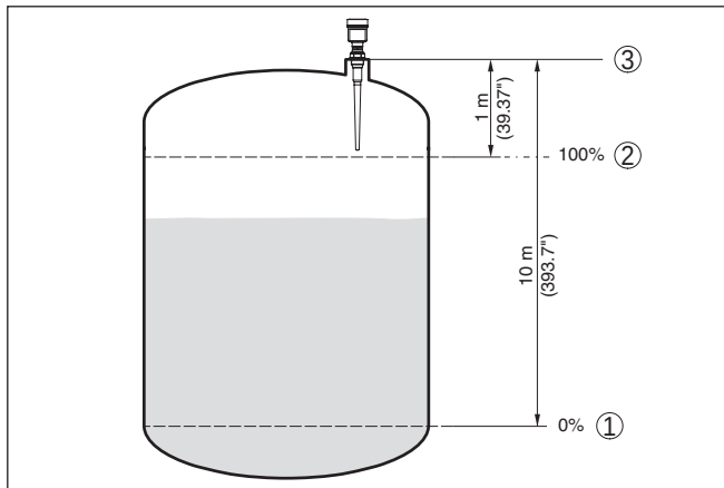
Fig. 26: Parametreervoorbeeld min.-/max.-inregeling
