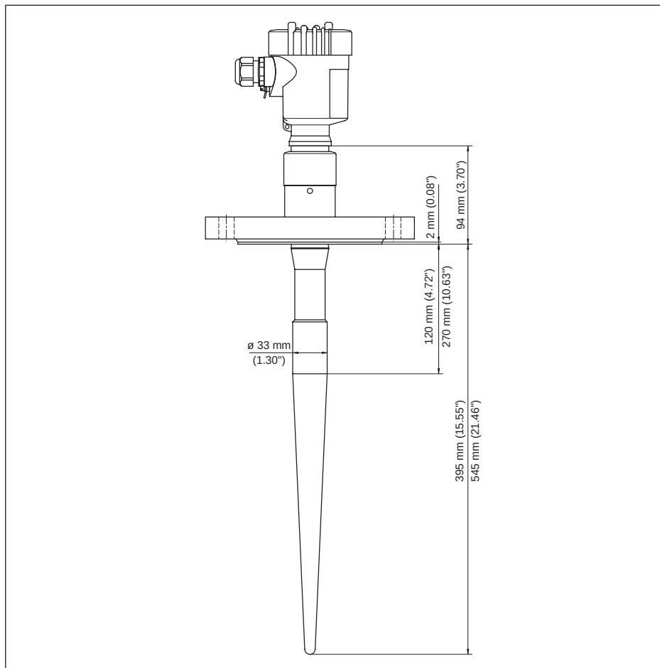
Fig. 51: VEGAPULS 65 - flensuitvoering voor sokken met 100 mm hoogte (inactieve lengte 120 mm, 4 23/32") resp. 250 mm hoogte (inactieve lengte 270 mm, 10 5/8")
