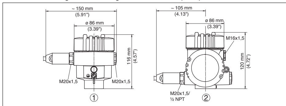
Fig. 49: Huisuitvoeringen in beschermingsklasse IP 66/IP 68, (1 bar), (met ingebouwde display- en bedieningsmodule wordt het huis 18 mm hoger)
