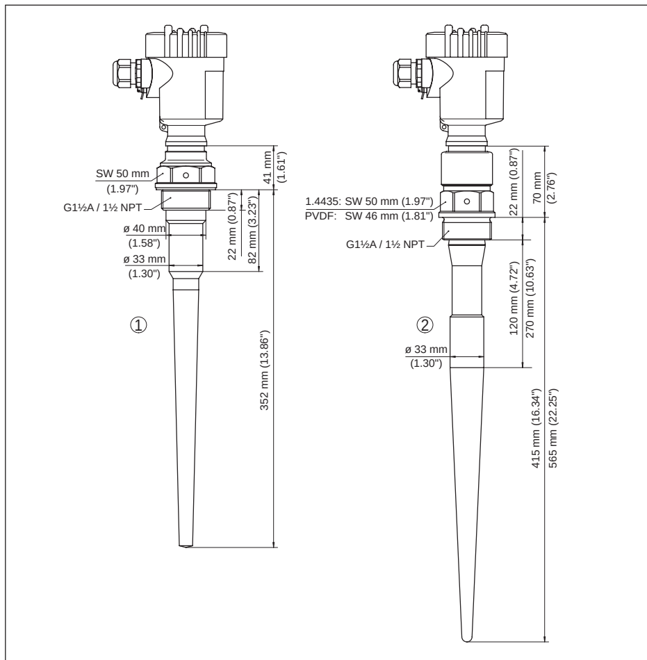
Fig. 50: VEGAPULS 65, schroefdraaduitvoering
