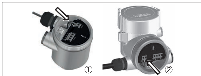
Fig. 11: Aansluitstappen 5 en 6
