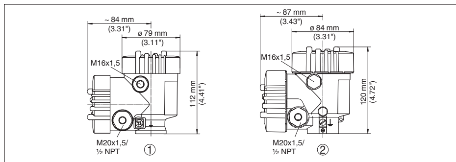
Abb. 42: Maße Gehäuse (mit eingebautem Anzeige- und Bedienmodul vergrößert sich die Gehäusehöhe um 9 mm/0.35 in, bei Metallgehäusen um 18 mm/0.71 in)
