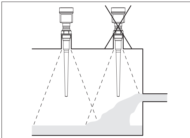
Abb. 6: Montage des Radarsensors bei einströmendem Medium
