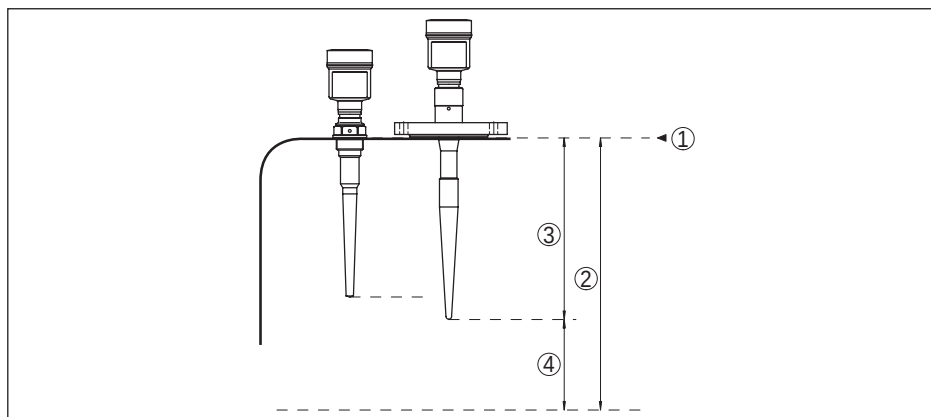
Abb. 40: Daten zur Eingangsgröße
