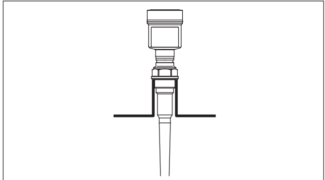
Abb. 7: Empfehlenswerte Rohrstützenmontage
