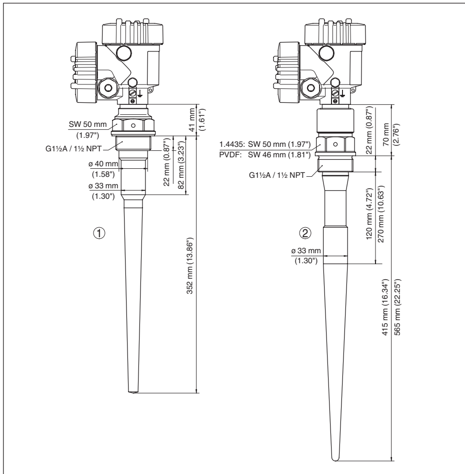
Abb. 43: VEGAPULS 65, Gewindeausführung
