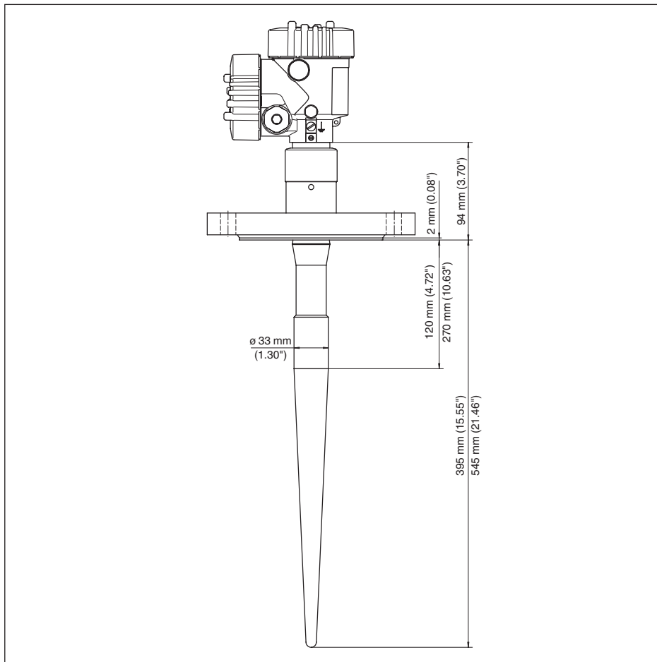
Abb. 44: VEGAPULS 65, Flanschausführung für Stutzen mit 100 mm Höhe (inaktive Länge 120 mm, 4 23/32") bzw. 250 mm Höhe (inaktive Länge 270 mm, 10 5/8")
