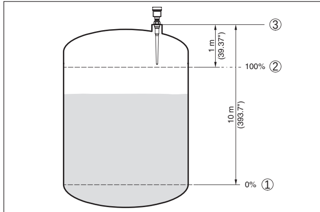
Abb. 21: Parametrierbeispiel Min.-/Max.-Abgleich
