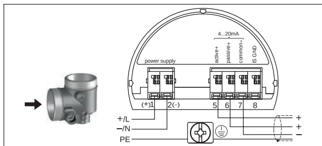
Abb. 13: Anschlussraum Zweikammergehäuse bei Netzspannung
