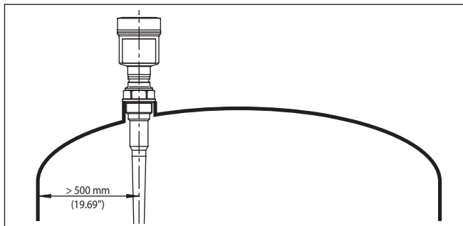
Abb. 4: Montage des Radarsensors an runden Behälterdecken
