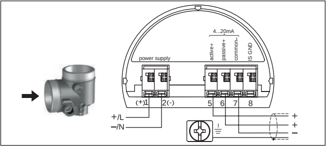
Abb. 14: Anschlussraum Zweikammergehäuse bei Kleinspannung
