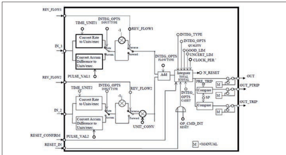
Abb. 37: Schematische Darstellung Funktionsblock Integrator
