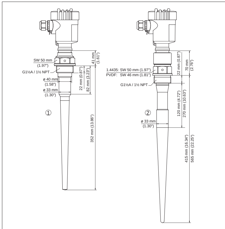
Abb. 43: VEGAPULS 65, Gewindeausführung
