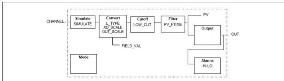
Abb. 32: Schematische Darstellung Funktionsblock Analog Input (AI)
