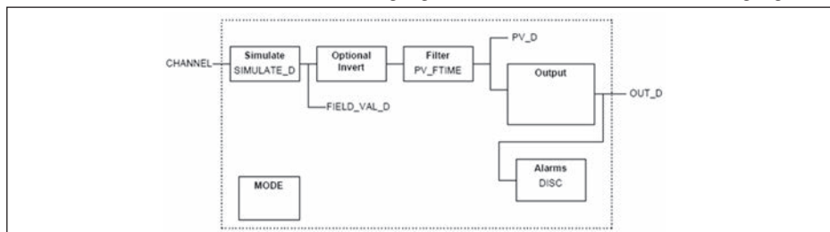
Abb. 33: Schematische Darstellung Funktionsblock Discret Input (DI)
