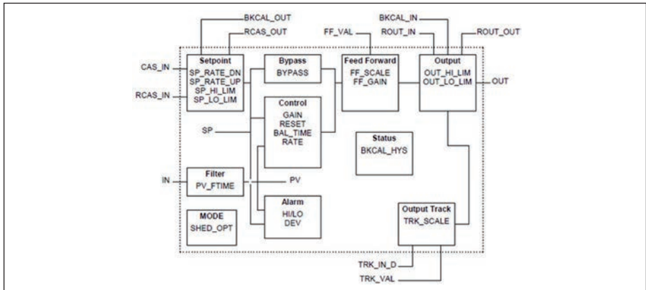
Abb. 34: Schematische Darstellung Funktionsblock PID Control
