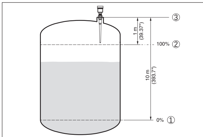
Abb. 25: Parametrierbeispiel Min.-/Max.-Abgleich
