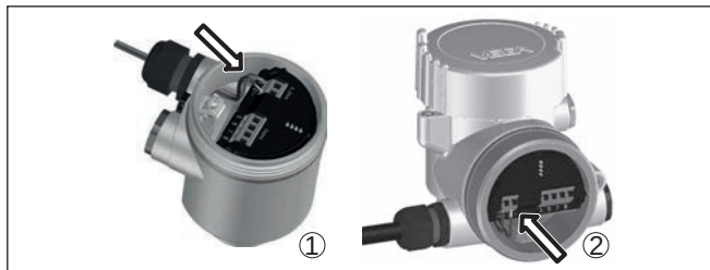
Abb. 11: Anschlusschritte 5 und 6
