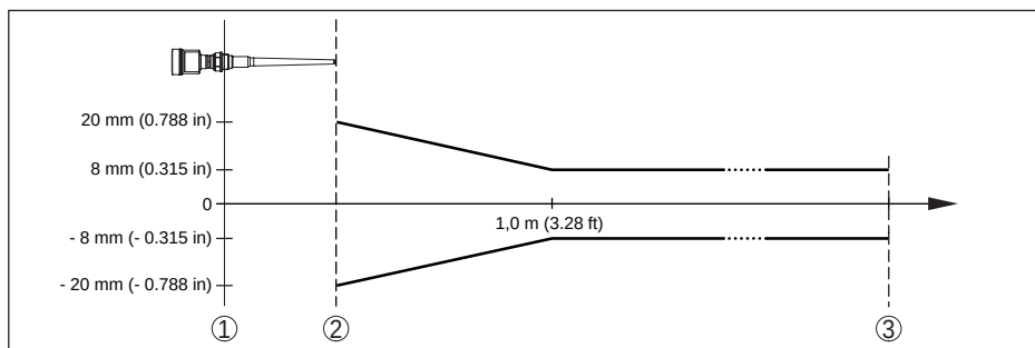
Abb. 30: Messabweichung unter Referenzbedingungen
