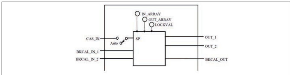
Abb. 35: Schematische Darstellung Funktionsblock Output Splitter
