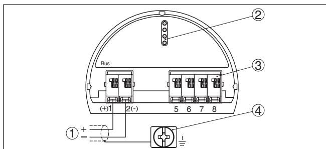
Abb. 14: Anschlussraum - Zweikammergehäuse
