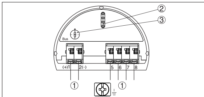
Abb. 13: Elektronikraum - Zweikammergehäuse
