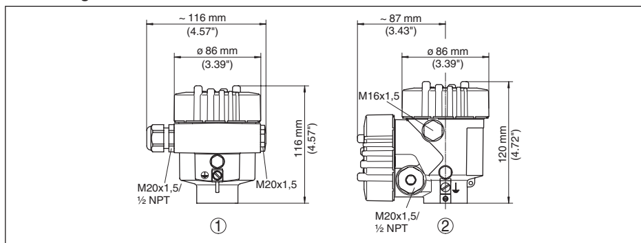
Abb. 41: Gehäuseausführungen in Schutzart IP 66/IP 68 (0,2 bar), (mit eingebautem Anzeige- und Bedienmodul vergrößert sich die Gehäusehöhe um 18 mm/0.71 in)
