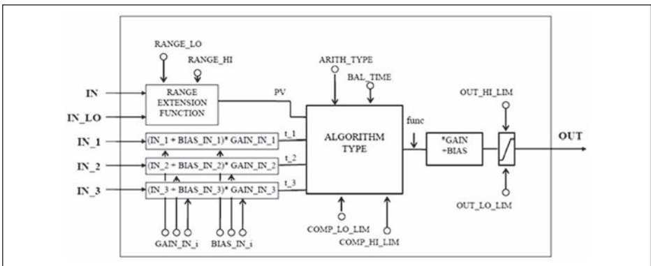
Abb. 39: Schematische Darstellung Funktionsblock Arithmetic
