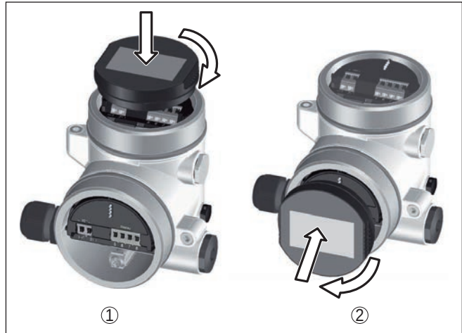
Abb. 22: Einsetzen des Anzeige- und Bedienmoduls beim Zweikammergehäuse
