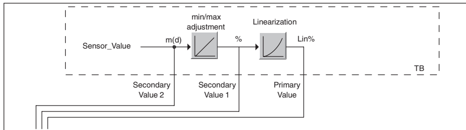
Abb. 31: Schematische Darstellung Transducer Block (TB)
