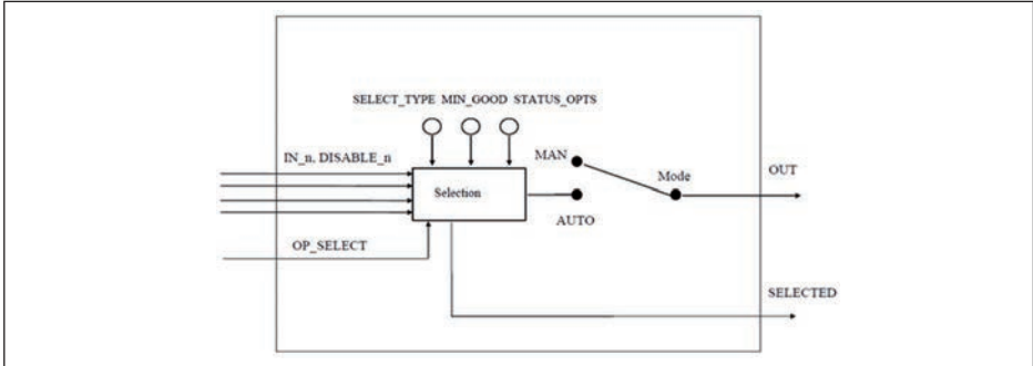
Abb. 38: Schematische Darstellung Funktionsblock Input Selector
