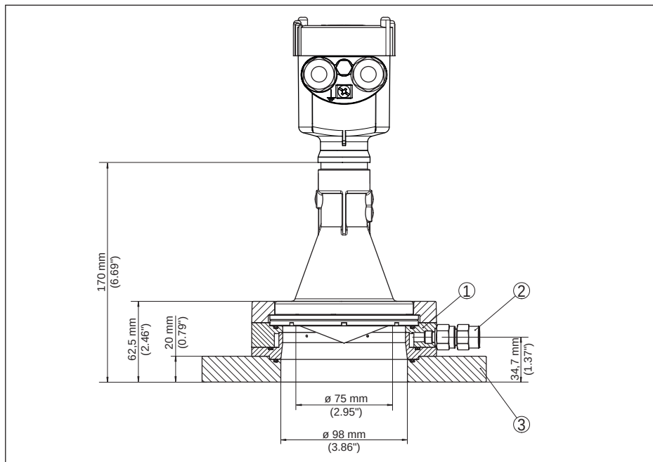
Fig. 63: VEGAPULS 67, adapterflens met luchtspoeling
