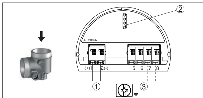
Fig. 28: Elektronicaruimte - Ex-ia-tweekamerbehuizing
