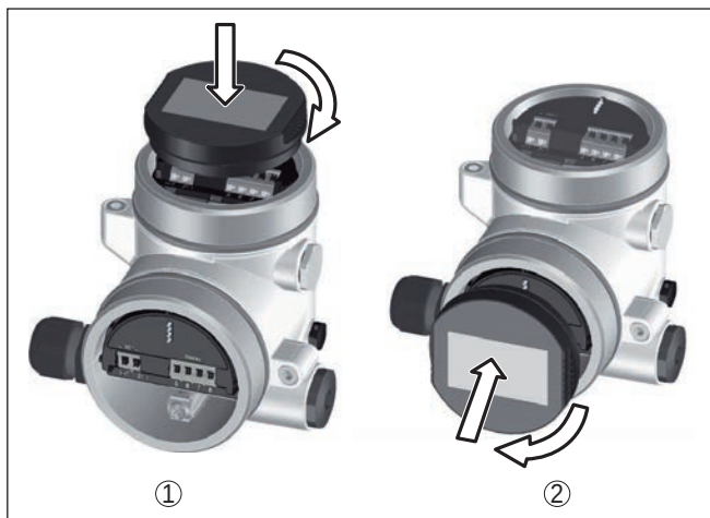
Fig. 35: Plaatsen van de display- en bedieningsmodule bij de tweekamerbehuizing
