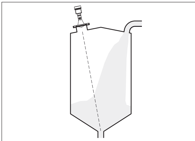
Fig. 8: Montage van de radarsensor bij instromend product met vullen van bovenaf.
