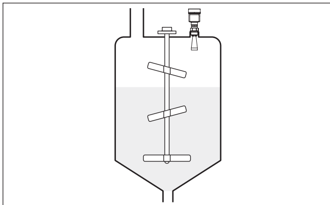
Fig. 18: Roerwerken
