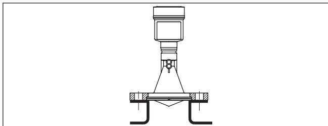
Fig. 10: Aanbevolen montage sok
