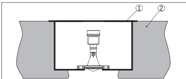
Fig. 19: Montage van het instrument in een ondervloerdoos
