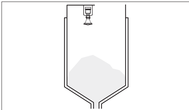
Fig. 3: Radarsensor met montagebeugel
