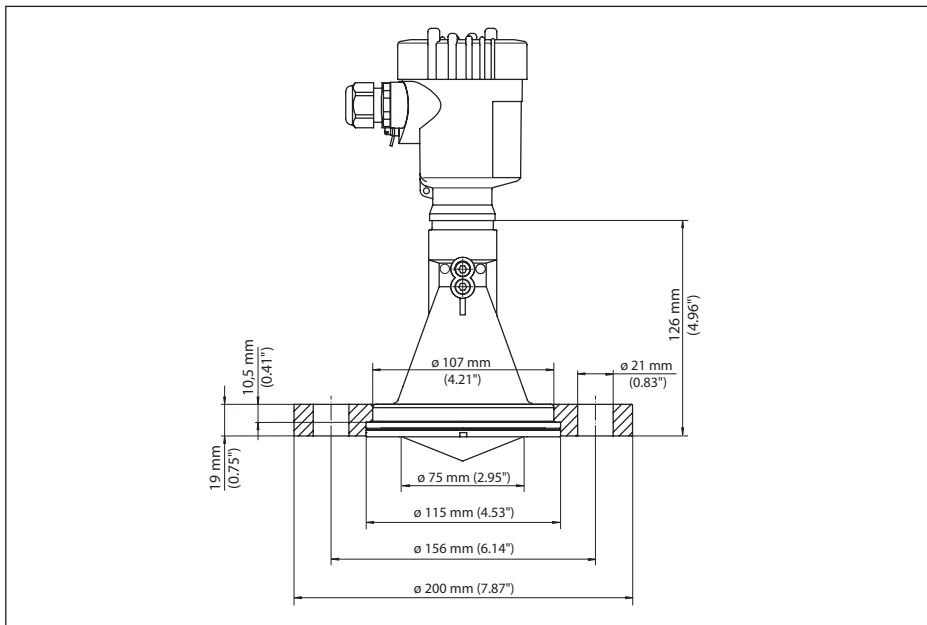
Fig. 60: VEGAPULS 67, overschuifflens passend voor DN 80 PN 16, ASME 3" 150lbs, JIS80 10K
