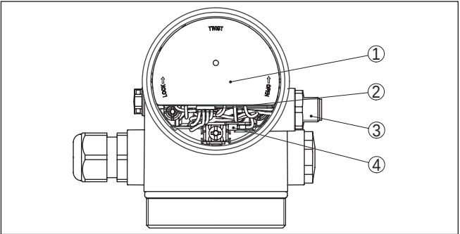
Fig. 31: Een blik op de elektronicaruimte met VEGADIS-adapter voor aansluiting van de externe display- en bedieningseenheid
