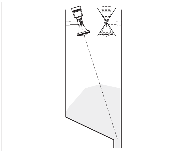
Fig. 21: Inbouw en uitrichting in meerkamersilo's
