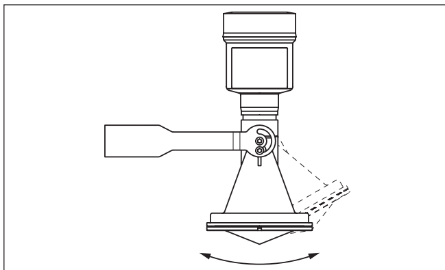
Fig. 4: Verstelling van de hellingshoek
