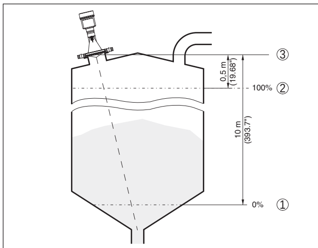
Fig. 38: Parametrevoorbeeld min.-/max.-inregeling
