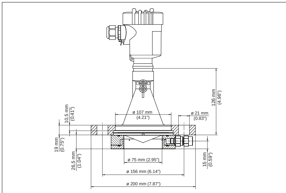
Fig. 61: VEGAPULS 67, overschuifflens met spoelaansluiting, passend voor DN 80 PN 16, ASME 3" 150lbs, JIS80 10K
