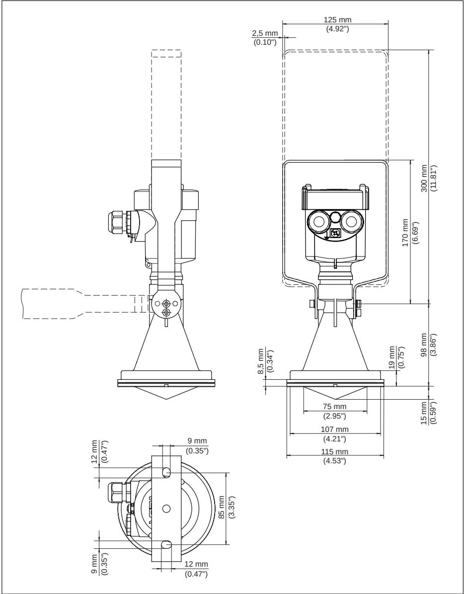
Fig. 59: VEGAPULS 67, montagebeugel in 170 of 300 mm lengte
