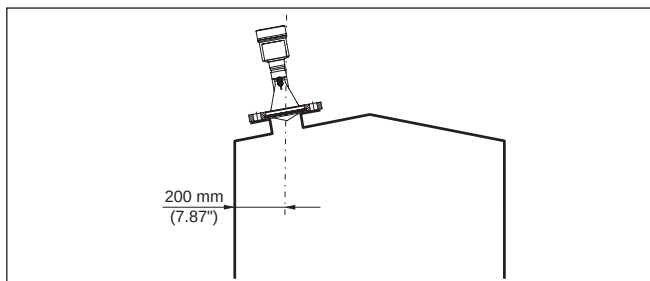
Fig. 7: Montage van de radarsensor op het tankdak
