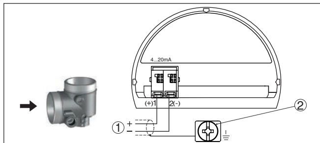
Fig. 29: Aansluitruimte - Ex-d-ia-tweekamerbehuizing
