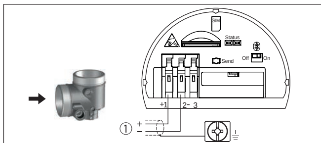
Fig. 27: Aansluitruimte - radiografische PLICSMOBILE 81
