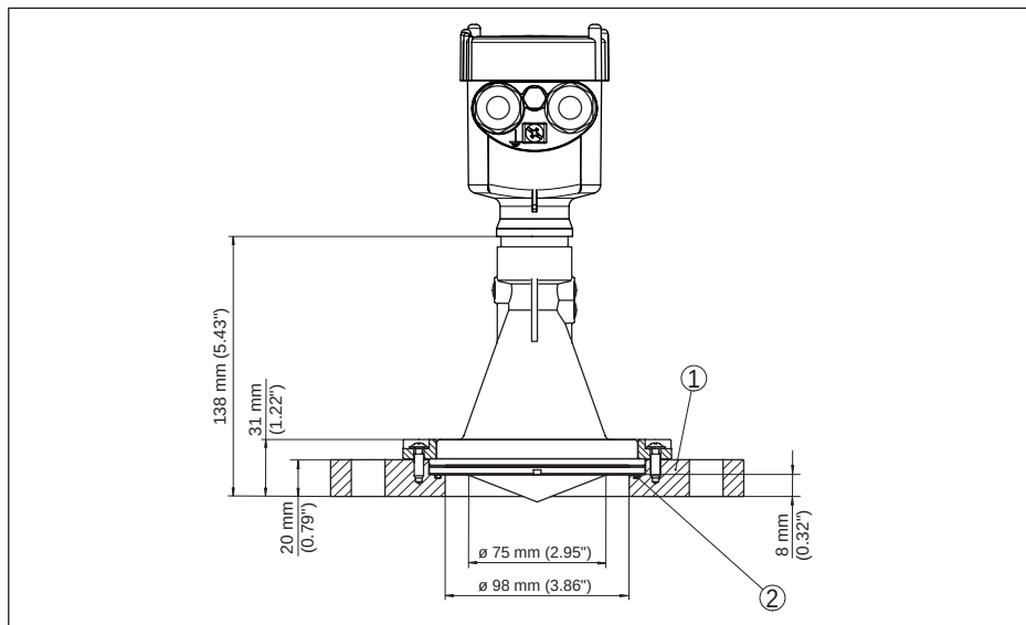
Fig. 62: VEGAPULS 67, adapterflens
