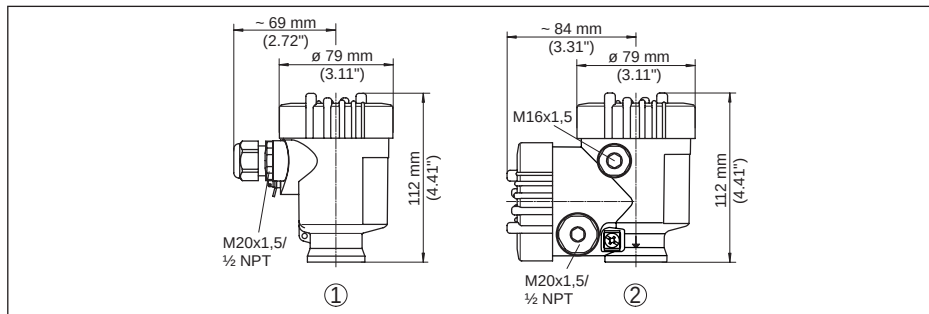
Fig. 54: Huisuitvoeringen in beschermingsklasse IP 66/IP 67 (met ingebouwde aanwijs- en bedieningsmodule wordt het huis 9 mm hoger)
