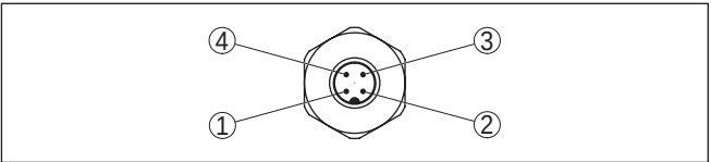
Fig. 32: Zicht op de connector M12 x 1
