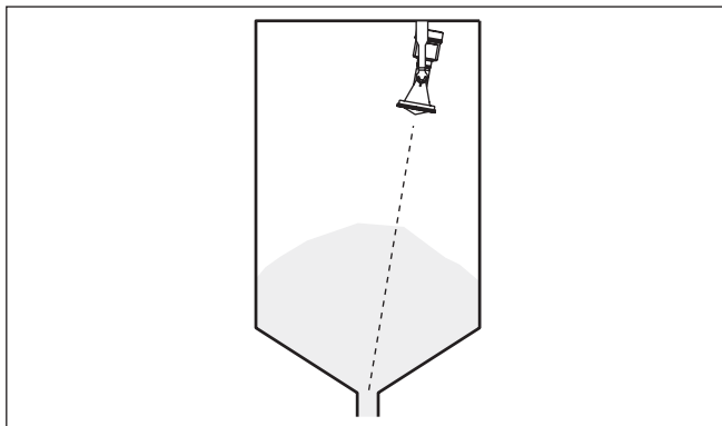
Fig. 14: Montage op tankdak
