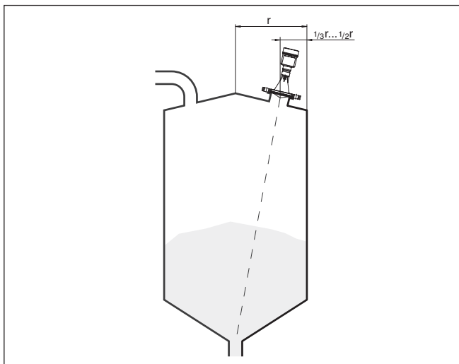
Fig. 15: Montagepositie en uitlijning
