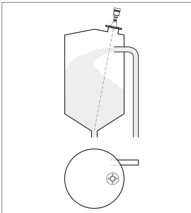
Fig. 9: Montage van de radarsensor bij instromend product vanaf de zijkant.
