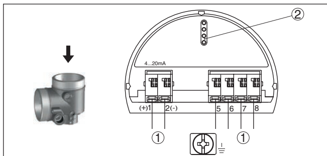
Fig. 25: Elektronicaruimte - tweekamerbehuizing
