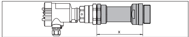
插图. 4: VEGAMIP 61 带安装适配件 "高温型" -40 ... +450 °C (-40 ... +842 °F)
