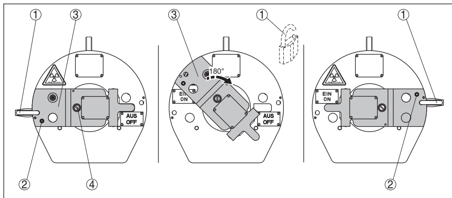
Fig. 33: Mise en marche du rayonnement - VEGASOURCE 31 Version D
