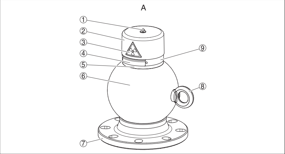
Fig. 38: Matériaux VEGASOURCE 31 - version A
