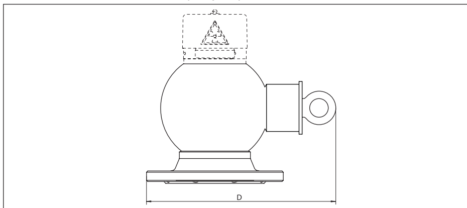
Fig. 54: Conteneur blindé VEGASOURCE 31 - version anti-feu (en option)
