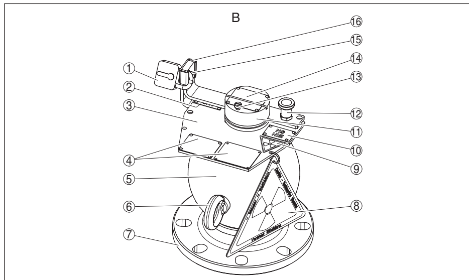
Fig. 39: Matériaux VEGASOURCE 31 - version B
