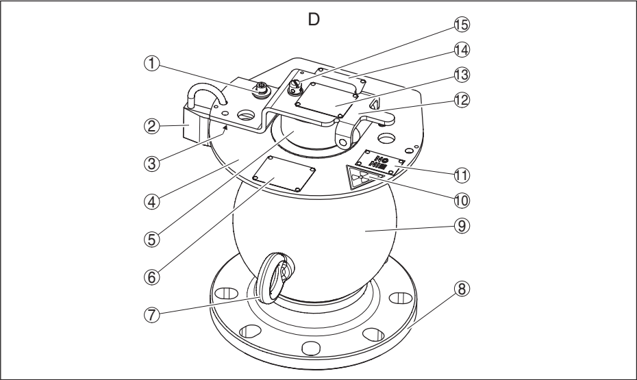
Fig. 41: Matériaux VEGASOURCE 31 - version D
