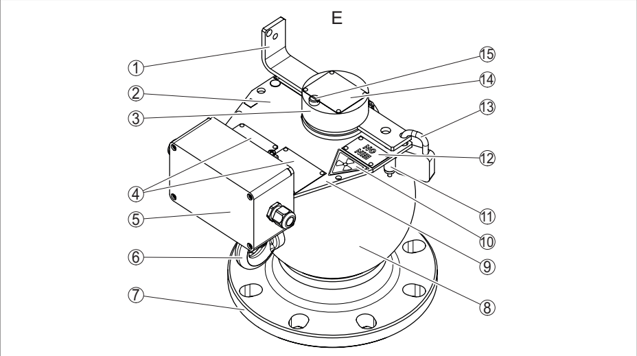
Fig. 42: Matériaux VEGASOURCE 31 - version E
