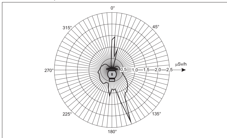
Fig. 45: Courbe iso-distance (distance : 1 m) - Exemple : conteneur blindé VEGASOURCE 31 avec Cs-137, 100 mCi (3,7 GBq)
