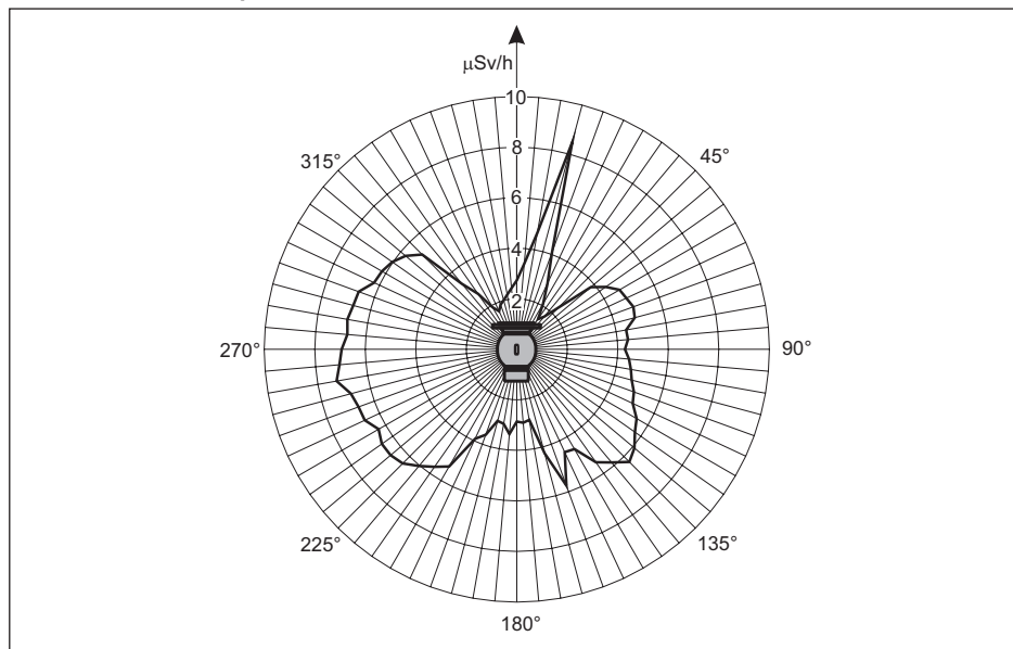
Fig. 44: Courbe iso-distance (distance : 1 m) - Exemple : conteneur blindé VEGASOURCE 31 avec Co-60, 20 mCi (0,74 GBq)
