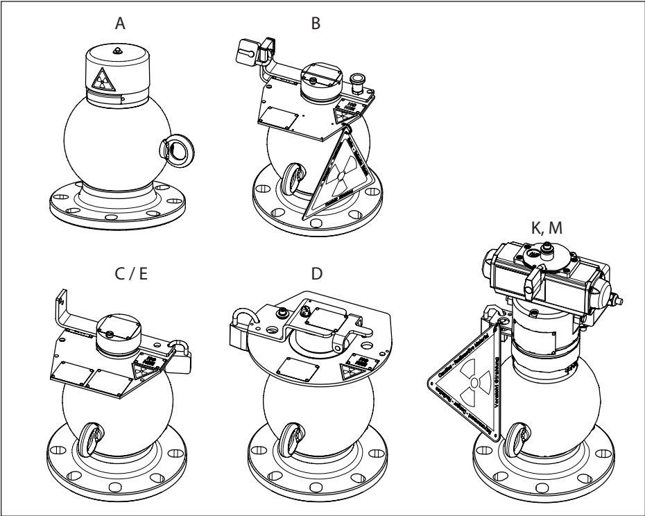
Fig. 2: Versions VEGASOURCE 31 (Aperçu)
