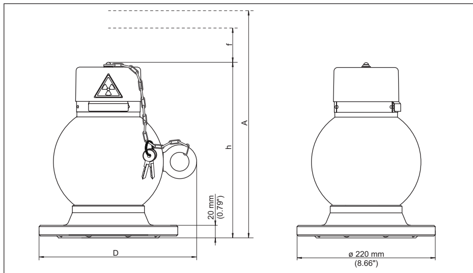
Fig. 46: Conteneur blindé VEGASOURCE 31 - Version A (insert de l'émetteur pour la commutation MARCHE/ARRÊT manuelle, serrure à insertion pour la sécurité de la commutation MARCHE ou ARRÊT, capot de protection)
