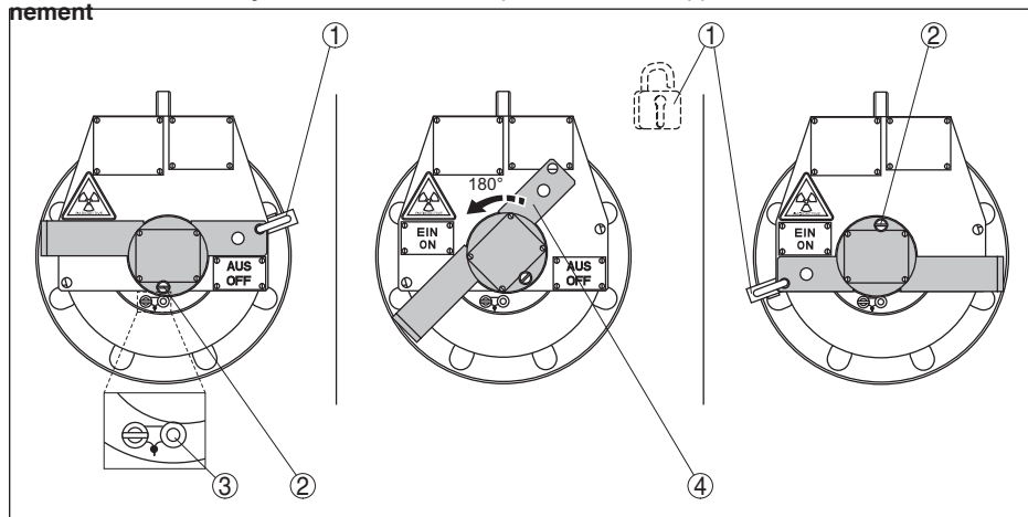
Fig. 32: Mise en marche du rayonnement - VEGASOURCE 31 Version C, E
