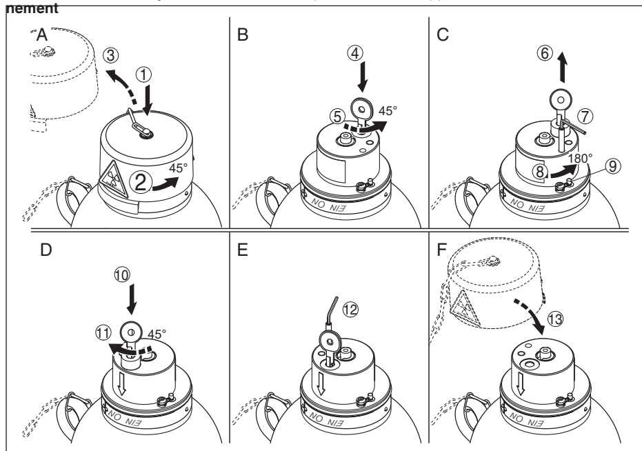
Fig. 30: Mise en marche du rayonnement - VEGASOURCE 31 Version A
