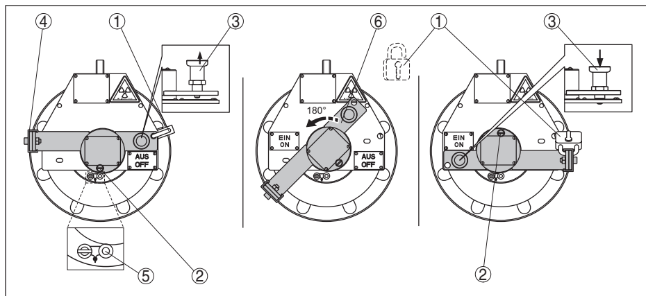
Fig. 31: Mise en marche du rayonnement - VEGASOURCE 31 Version B
