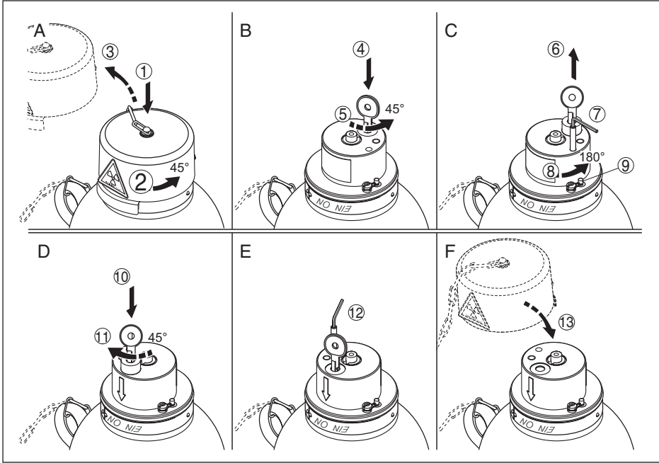
Res. 30: Işınlamanın açık konuma getirilmesi - VEGASOURCE 35 A modeli
