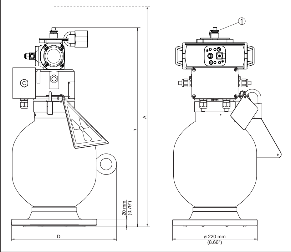
Res. 52: VEGASOURCE 35 ışından koruyucu hazne, M, N modeli
