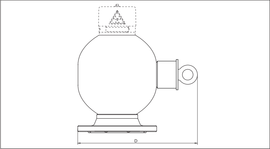
Res. 54: VEGASOURCE 35 ışıktan koruyucu hazne, ateşe dayanıklı model (Opsiyonel)
