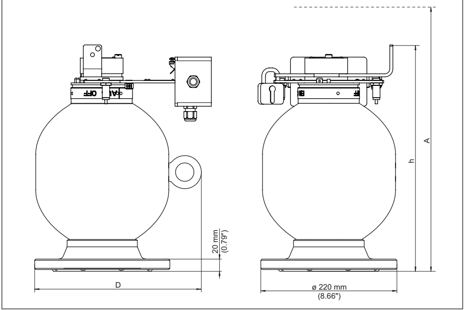
Res. 50: Işıktan koruyucu hazne VEGASOURCE 35, E modeli, (manüel açma/kapama anahtarı için döner bilezik, anahtarlama konumunun AÇIK veya KAPALI'da kilitlenebilmesi için asma kilit), konum alarmları da dahil
