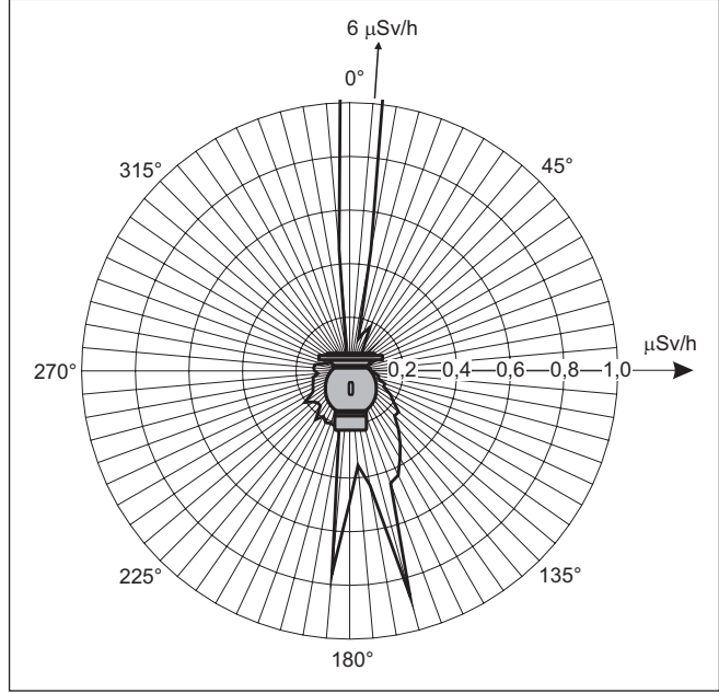
Res. 45: Eşit uzaklık eğimi (Mesafe: 1 m) - Örnek: Cs-137'li VEGASOURCE 35 ışından koruyucu hazne, 1000 mCi (37 GBq)
