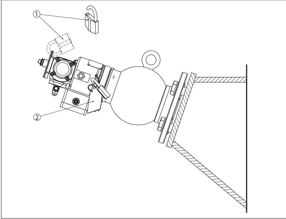
Res. 34: Pnömatik açma/kapama teçhizatlı ışınlananın açık konuma getirilmesi - VEGASOURCE 35 K, M modeli
