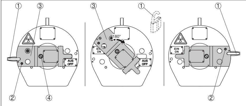
Res. 33: Işınlamanın açık konuma getirilmesi - VEGASOURCE 35 D modeli
