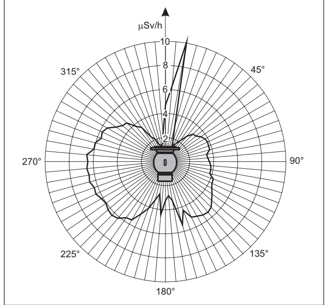
Res. 44: Eşit uzaklık eğimi (Mesafe: 1 m) - Örnek: Co-60'lu VEGASOURCE 35 ışıktan koruyucu hazne, 100 mCi (3,7 GBq)
