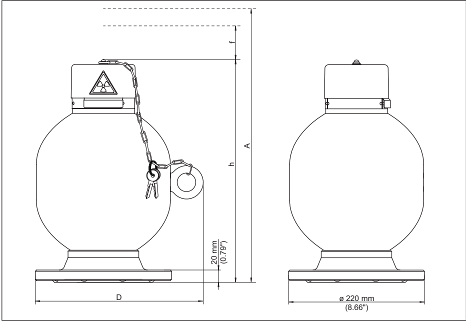
Res. 46: VEGASOURCE 35 ışıktan koruyucu hazne, A modeli (Elle AÇMA/KAPAMA ayarı için preparat modülü, AÇMA/KAPAMA ayarlarının kilitlenmesi için geçme kilit, koruyucu kapak)
