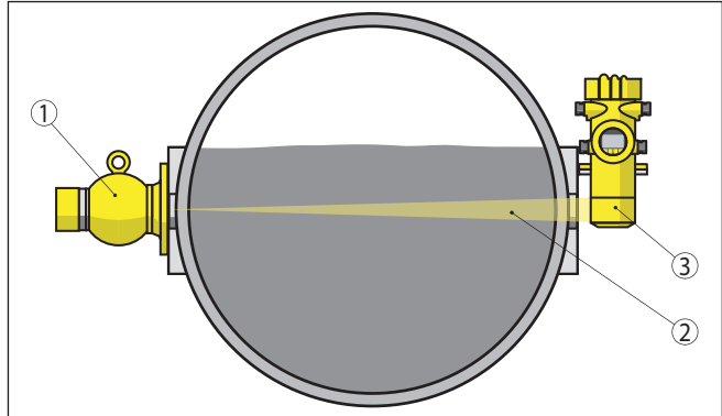
Res. 21: Yatay pozisyondaki bir boru hatında ölçüm düzeni
