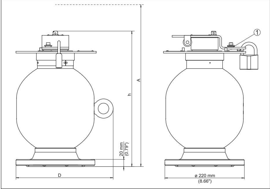
Res. 49: VEGASOURCE 35 ışıktan koruyucu hazne, D modeli
