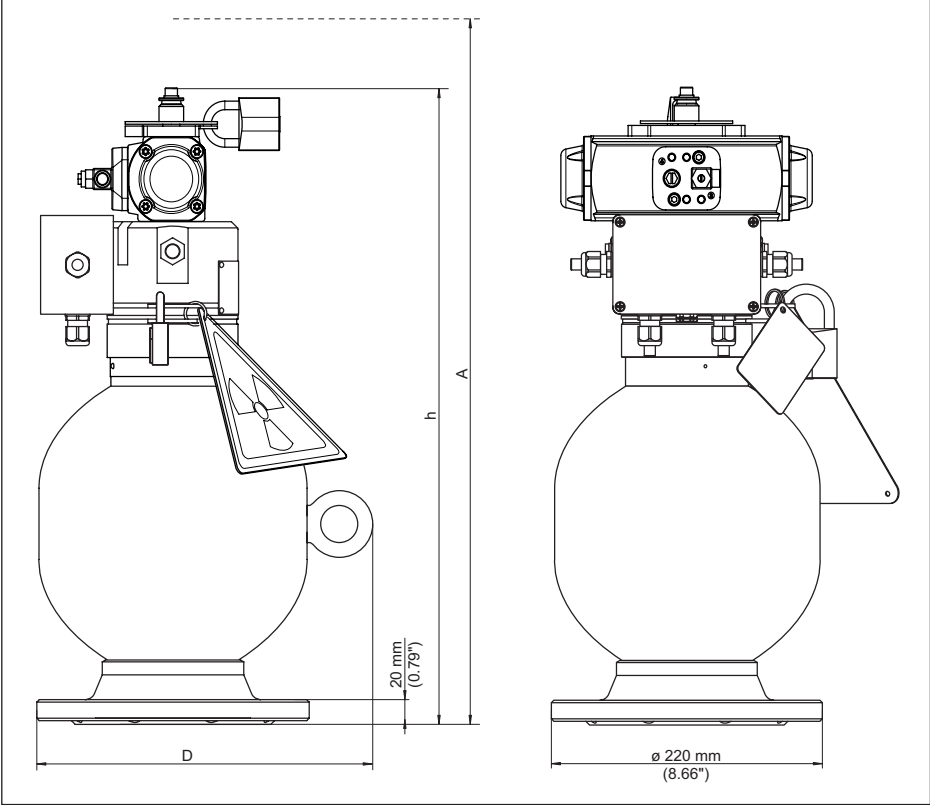
Res. 51: VEGASOURCE 35 ışından koruyucu hazne, K, L modeli
