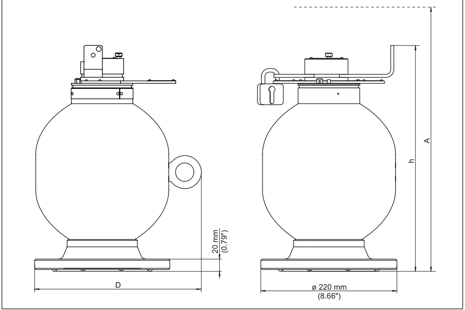
Res. 48: VEGASOURCE 35 ışından koruyucu hazne, C modeli (Elle AÇMA/KAPAMA ayarı için döner ibre, AÇMA/KAPAMA ayarlarının kilitlemesi için asma kilit)
