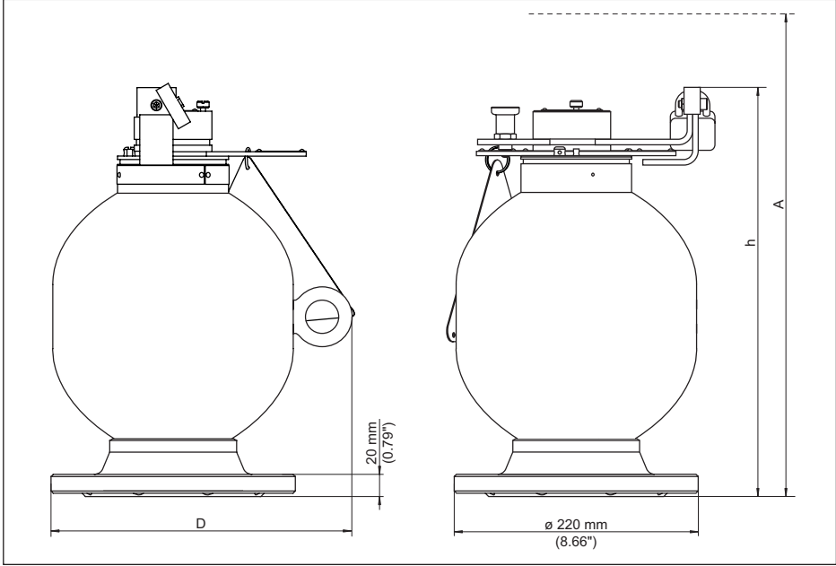
Res. 47: VEGASOURCE 35 ışından koruyucu hazne, B modeli (Elle AÇMA/KAPAMA ayarı için döner ibre, AÇMA ayarlarının kilitlemesi için sabitleme pimi, KAPAMA ayarının kilitlemesi için asma kilit)
