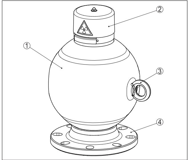
Res. 9: Işından koruyucu hazne VEGASOURCE 35
