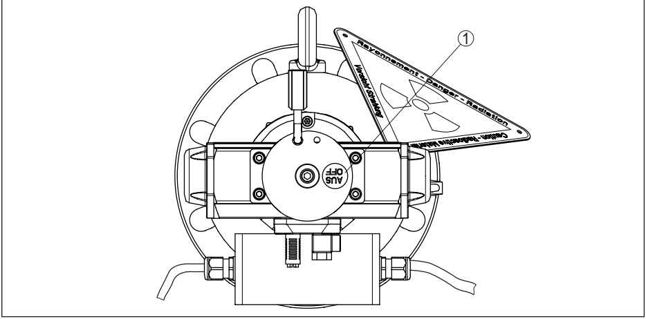
Res. 35: VEGASOURCE 35'de anahtarlama durumunun görüntülenmesi - K, M modeli
