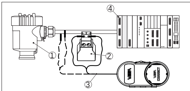
Fig. 42: Aansluiting van de PC via HART op de signaalkabel
