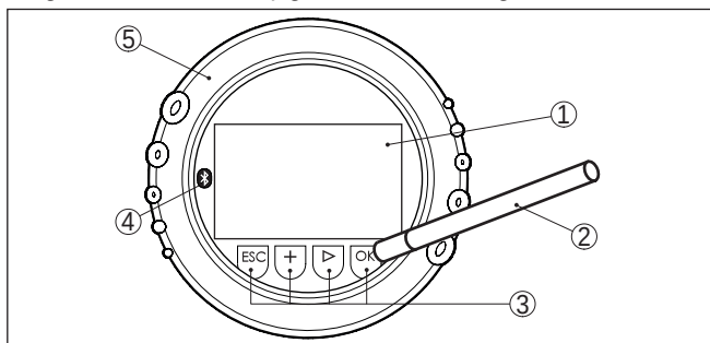
Fig. 39: Display- en bedieningselement - met bediening via magneetpen
