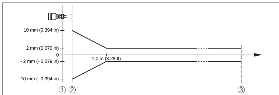
Fig. 55: Meetnauwkeurigheid onder referentiecondities
