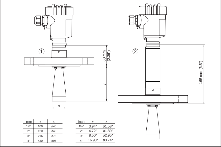
Fig. 62: VEGAPULS SR 68, hoornantenne in flensuitvoering
