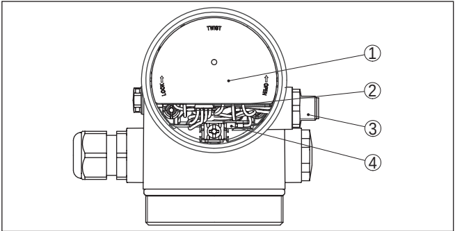
Fig. 33: Een blik op de elektronicaruimte met VEGADIS-adapter voor aansluiting van de externe display- en bedieningseenheid
