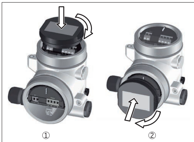
Fig. 37: Plaatsen van de display- en bedieningsmodule bij de tweekamerbehuizing
