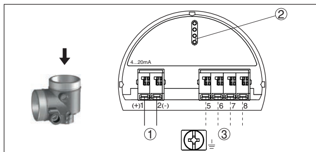
Fig. 30: Elektronicaruimte - Ex-ia-tweekamerbehuizing
