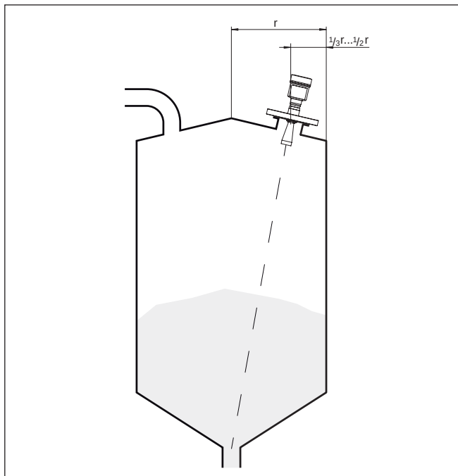
Fig. 13: Uitrichting
