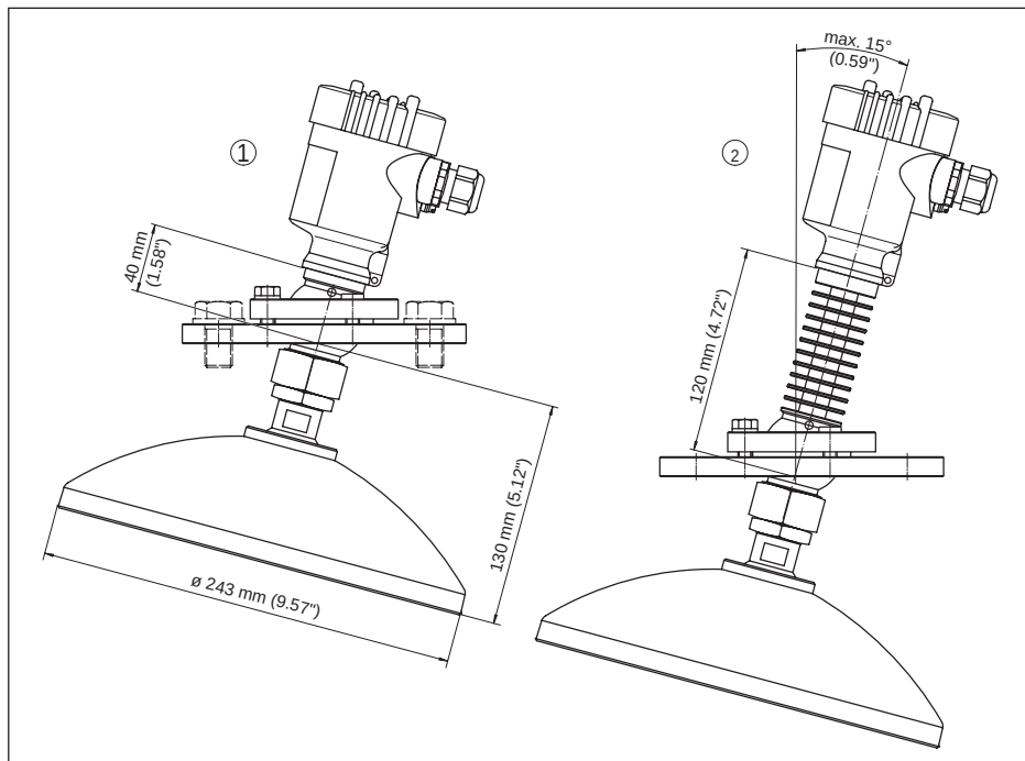
Fig. 64: VEGAPULS SR 68, paraboolantenne en zwenkflens
