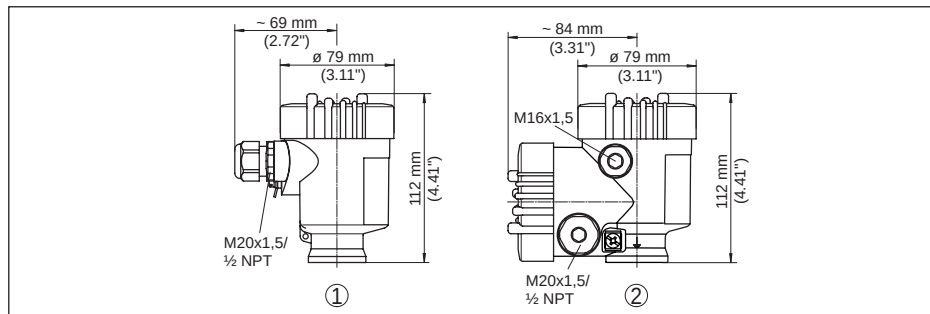
Fig. 56: Huisuitvoeringen in beschermingsklasse IP 66/IP 67 (met ingebouwde aanwijs- en bedieningsmodule wordt het huis 9 mm hoger)
