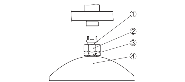
Fig. 3: Demontage paraboolantenne.
