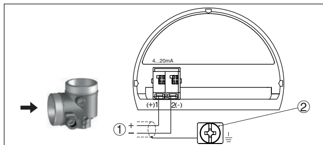
Fig. 31: Aansluitruimte - Ex-d-ia-tweekamerbehuizing
