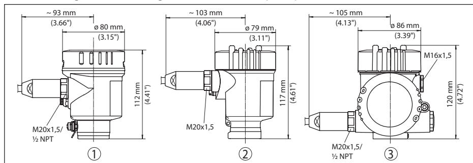
Fig. 60: Huisuitvoeringen in beschermingsklasse IP 66/IP 68, (1 bar), (met ingebouwde display- en bedieningsmodule wordt het huis 18 mm hoger)
