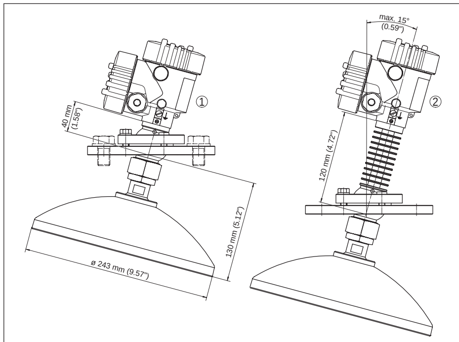
Fig. 56: VEGAPULS SR 68, paraboolantenne en zwenkflens
