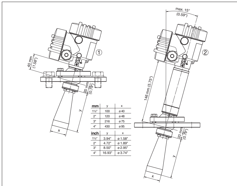
Fig. 55: VEGAPULS SR 68, hoornantenne en zwenkflens
