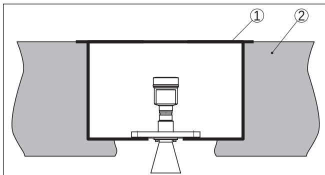
Fig. 21: Montage van het instrument in een ondervloerdoos
