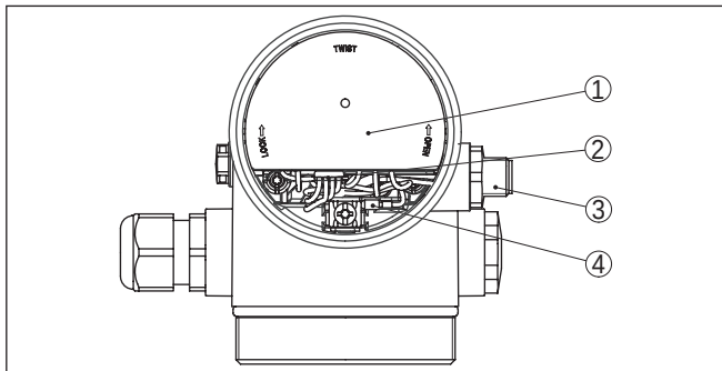
Fig. 30: Een blik op de elektronicarimte met VEGADIS-adapter voor aansluiting van de externe display- en bedieningseenheid
