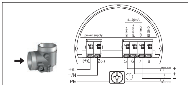
Fig. 28: Aansluitruimte tweekamerbehuizing bij netspanning
