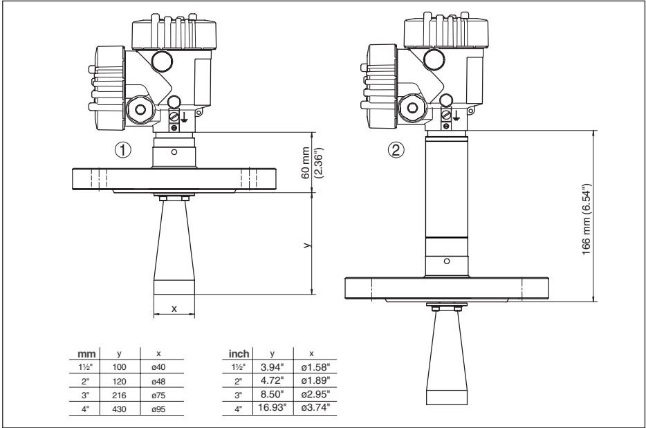
Fig. 54: VEGAPULS SR 68, hoornantenne in flensuitvoering
