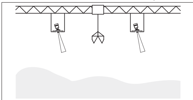
Fig. 19: Radarsensoren aan een bovenloopkraan
