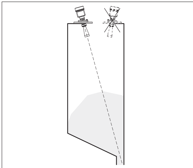
Fig. 23: Uitrichting van de VEGAPULS SR 68 op het aftappunt in het midden van de silo
