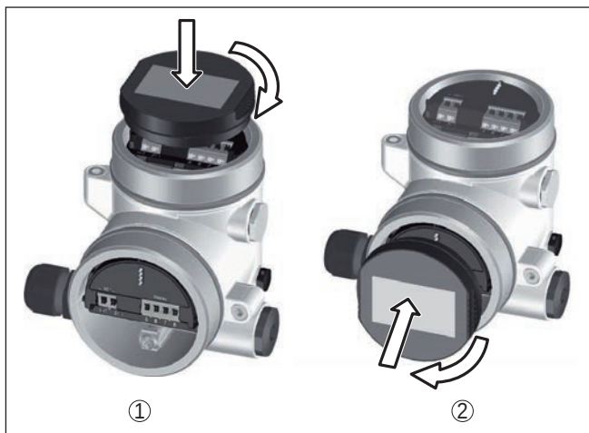
Fig. 33: Plaatsen van de display- en bedieningsmodule bij de tweekamerbehuizing
