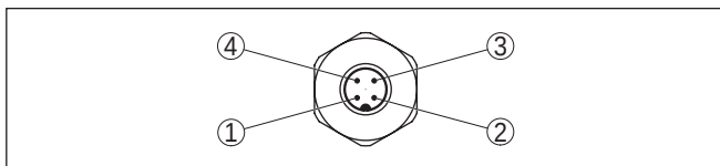
Fig. 31: Zicht op de connector M12 x 1
