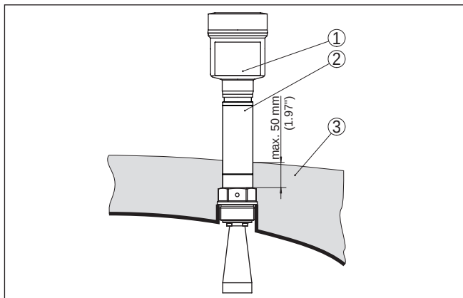
Fig. 20: Montage van het instrument in geïsoleerde tanks.
