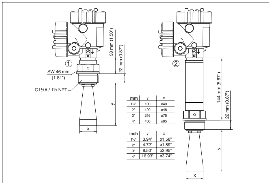
Fig. 53: VEGAPULS SR 68, hoornantenne in schroefdraaduitvoering
