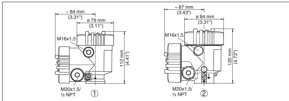
Fig. 52: Afmetingen behuizing (met ingebouwde display- en bedieningsmodule wordt de hoogte van de behuizing 9 mm groter, bij metalen behuizingen 18 mm)
