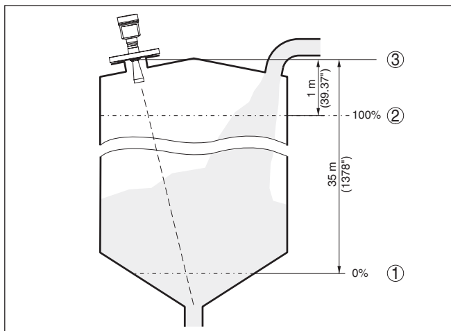
Fig. 36: Parametreervoorbeeld min.-/max.-inregeling
