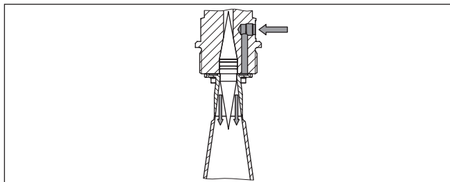
Fig. 24: Spoelluchtaansluiting bij hoornantenne
