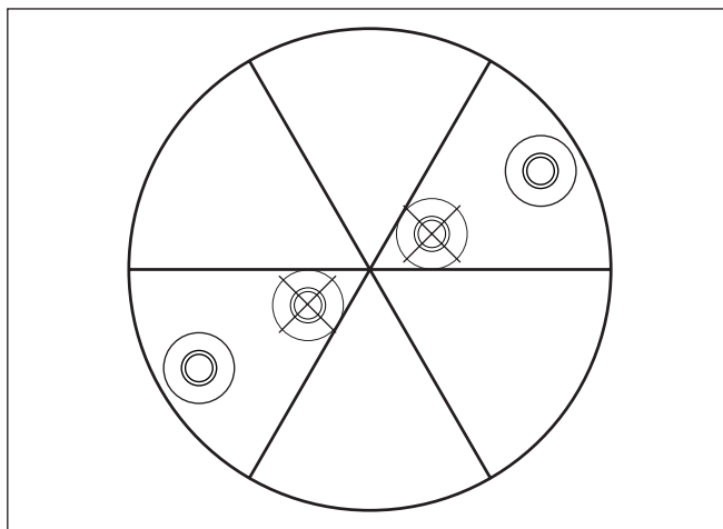
Fig. 22: Montage van de VEGAPULS SR 68 in meerkamersilo's
