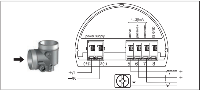
Fig. 29: Aansluitruimte tweekamerbehuizing bij laagspanning
