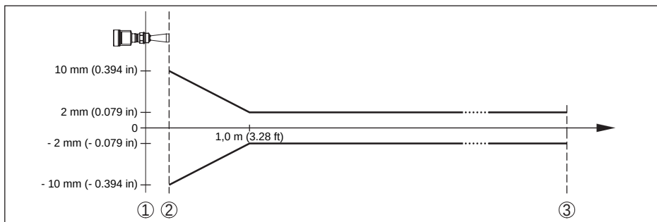
Fig. 51: Meetnauwkeurigheid onder referentiecondities
