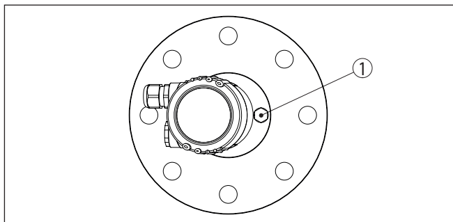
Fig. 16: VEGAPULS SR 68 met zwenkflens
