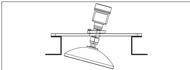
Fig. 12: Afstand tussen antenne en aansluiting bij paraboolantenne
