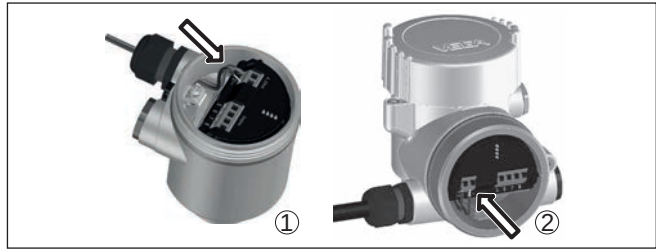
Fig. 25: Aansluitstappen 5 en 6
