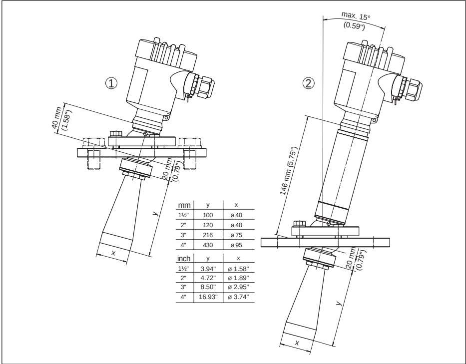
Fig. 64: VEGAPULS SR 68, hoornantenne en zwenkflens
