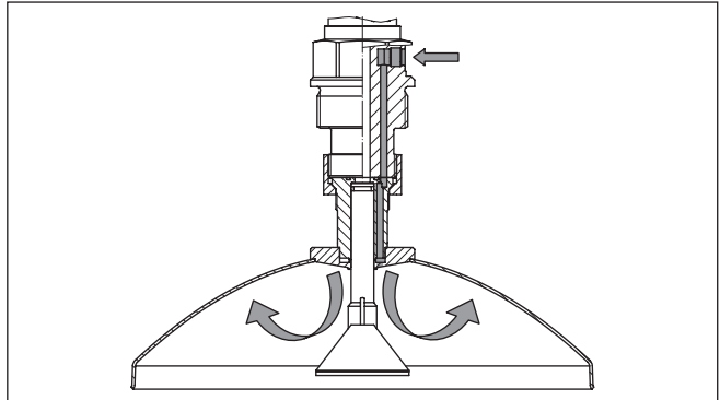
Fig. 24: Spoelluchtaansluiting bij parabolantenne
