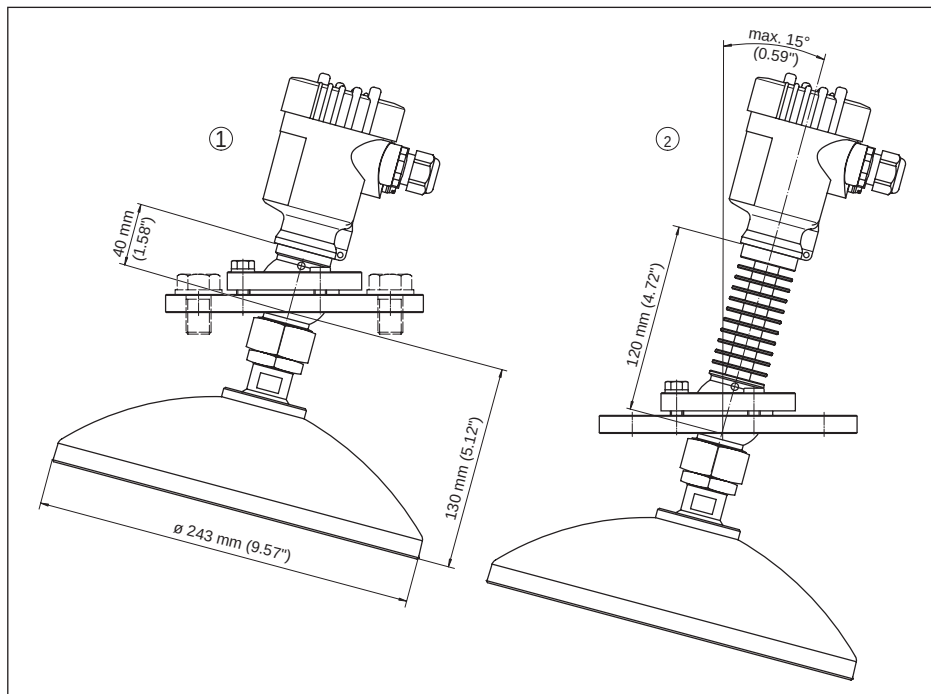
Fig. 65: VEGAPULS SR 68, paraboolantenne en zwenkflens
