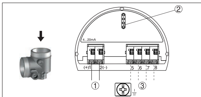
Fig. 29: Elektronicaruimte - Ex-ia-tweekamerbehuizing
