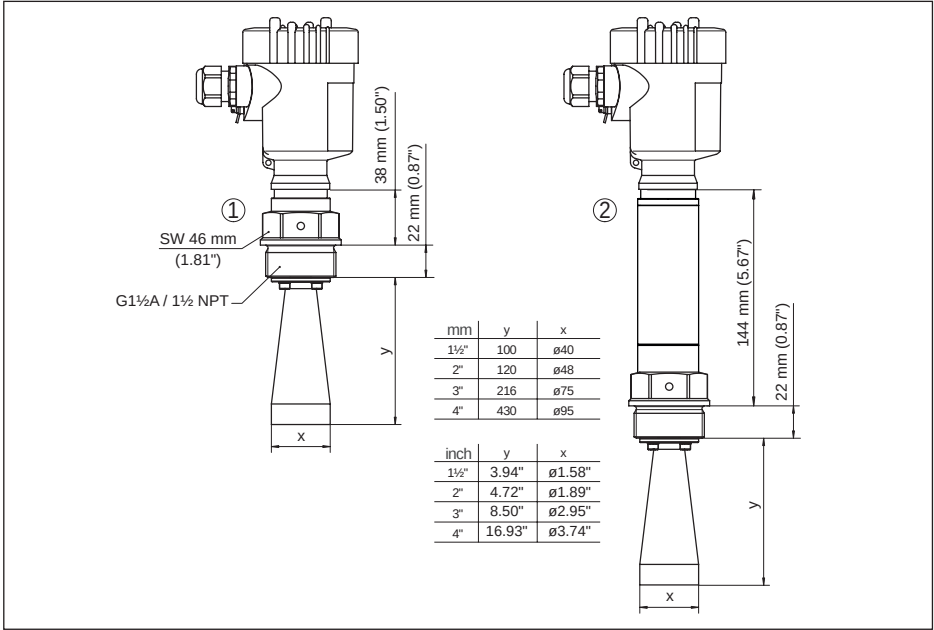
Fig. 62: VEGAPULS SR 68, hoornantenne in schroefdraaduitvoering
