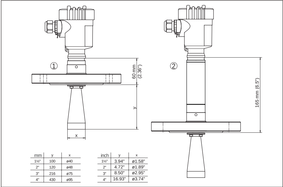
Fig. 63: VEGAPULS SR 68, hoornantenne in flensuitvoering
