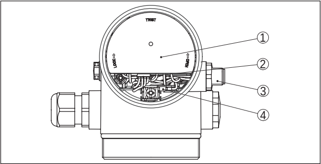
Fig. 32: Een blik op de elektronicaruimte met VEGADIS-adapter voor aansluiting van de externe display- en bedieningseenheid
