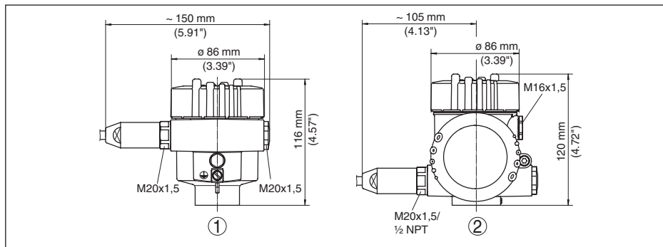
Fig. 59: Huisuitvoeringen in beschermingsklasse IP 66/IP 68, (1 bar), (met ingebouwde display- en bedieningsmodule wordt het huis 18 mm hoger)
