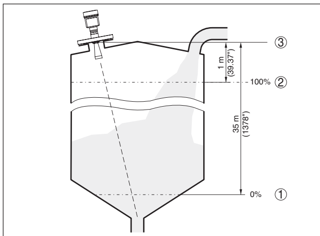
Fig. 39: Parametrevoorbeeld min.-/max.-inregeling
