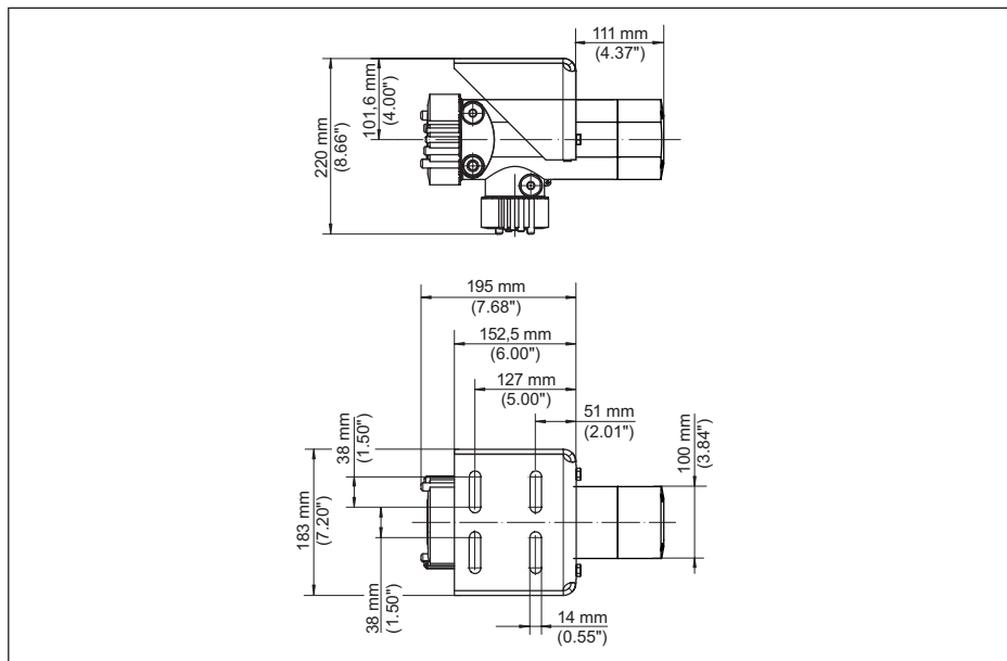
Fig. 26: POINTRAC 31 zonder detectorbuis, 46 mm (1,8 in) - met meegeleverde montagetoebehoren
