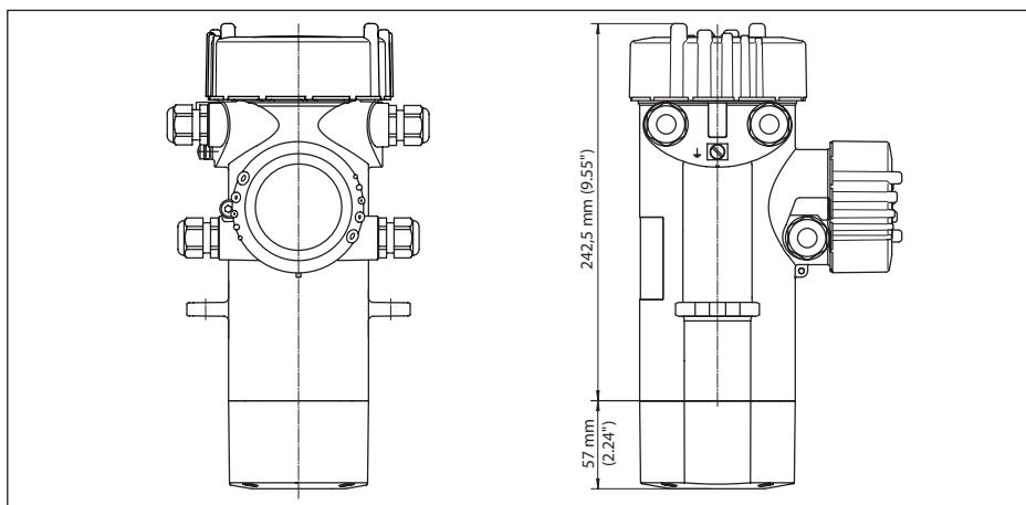
Fig. 25: POINTRAC 31 zonder detectorbuis - meetbereik = bestellengte 46 mm (1,8 in)
