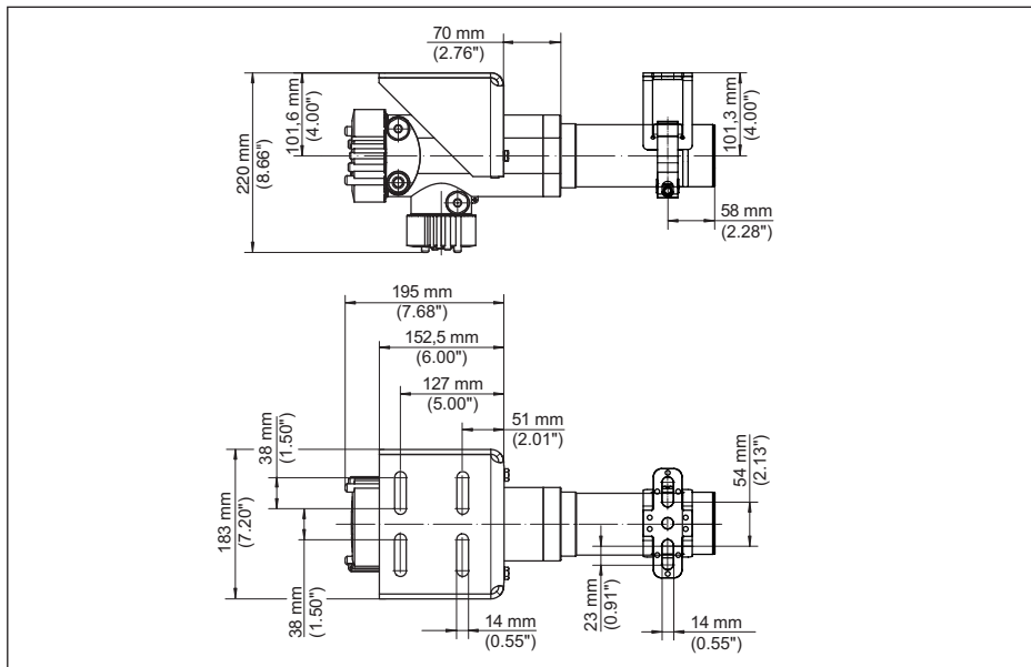
Fig. 24: POINTRAC 31 met detectorbuis, 152 mm of 304 mm (6 in/12 in) - met meegeleverde montage toebehoren
