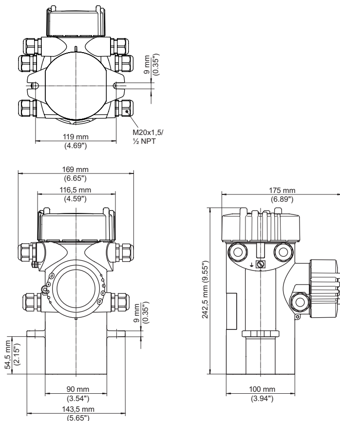
Fig. 22: Aluminium behuizing resp. rvs-behuizing (fijnjetwerk)
