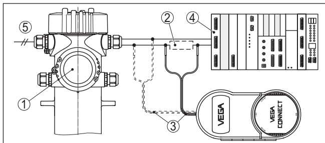
Fig. 18: Aansluiting van de PC via HART op de signaalkabel
