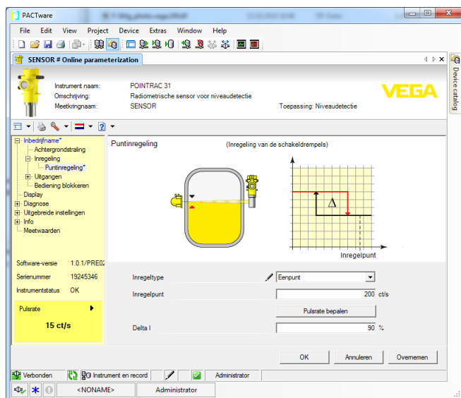
Fig. 19: Voorbeeld van een DTM-aanzicht
