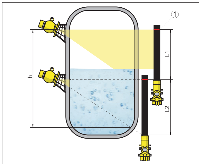
Fig. 7: Position de montage - Agencement en cascade
