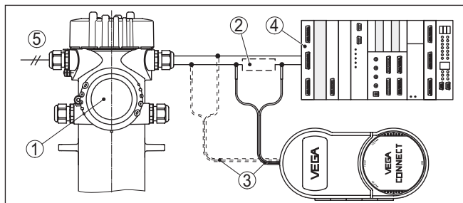
Fig. 24: Raccordement du PC à la ligne signal via HART
