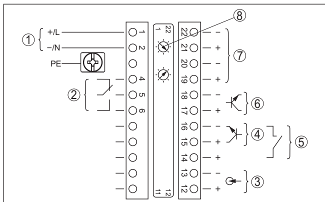
Fig. 12: Compartiment électronique et de raccordement (Ex d) des appareils avec sortie courant à sécurité intrinsèque
