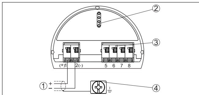
Fig. 13: Compartiment de réglage et de raccordement (Ex ia) des appareils avec sortie courant à sécurité intrinsèque
