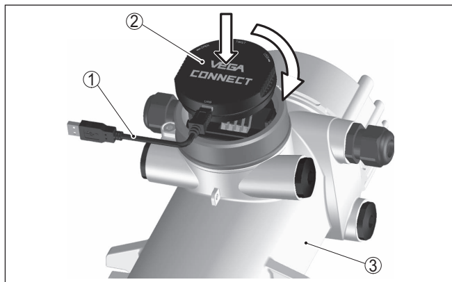
Fig. 23: Raccordement du PC directement au capteur via l'adaptateur d'inter- faces
