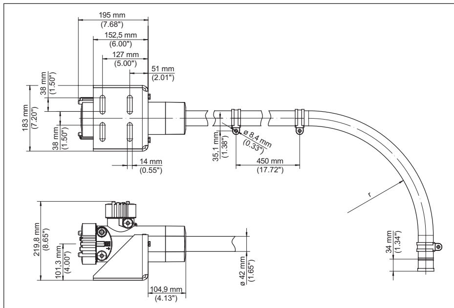
Fig. 31: FIBERTRAC 31 avec des accessoires de montage compris à la livraison
