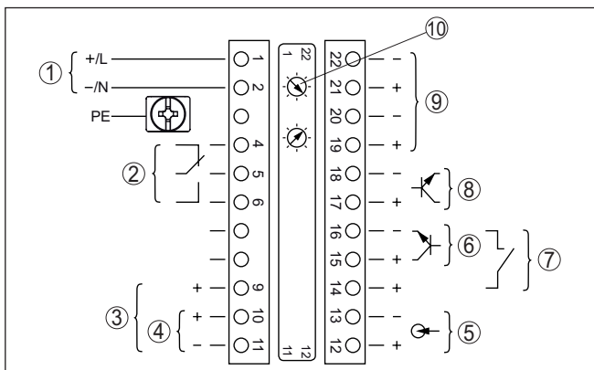
Fig. 14: Compartiment électronique et de raccordement des appareils non Ex et appareils avec sortie courant non à sécurité intrinsèque
