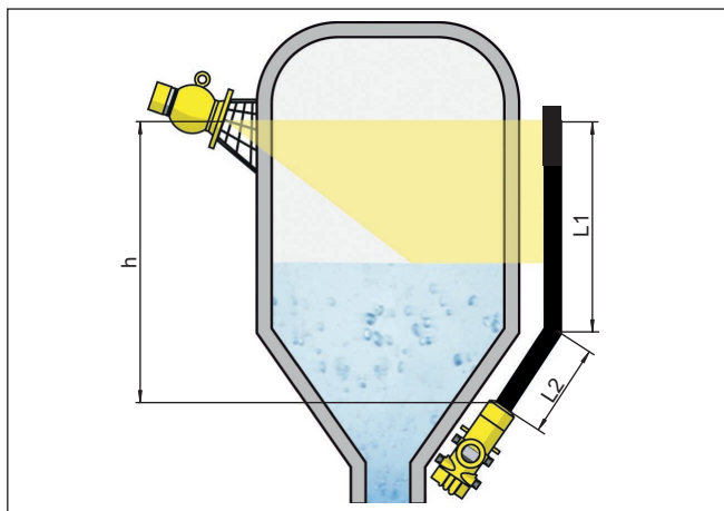
Fig. 5: Mesure de niveau dans une cuve de stockage
