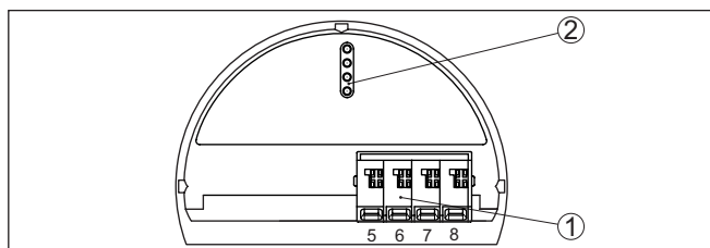
Fig. 15: Bedienings- en aansluitruimte bij niet-Ex instrumenten en instrumenten met niet-intrinsiekveilige stroomuitgang
