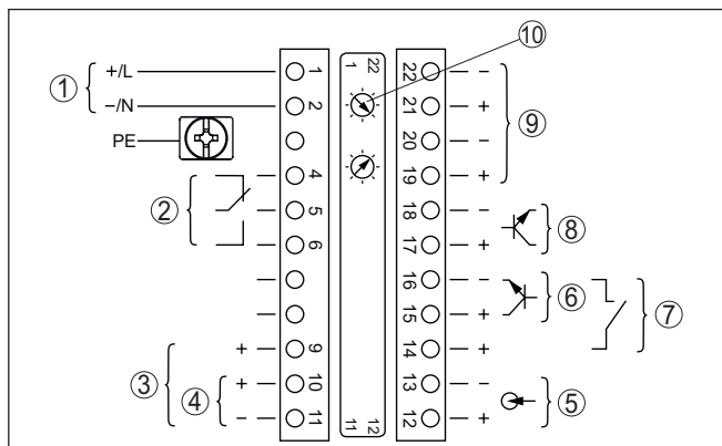
Fig. 14: Elektronica- en aansluitruimte bij niet-Ex instrumenten en instrumenten met niet-intrinsiekveilige stroomuitgang
