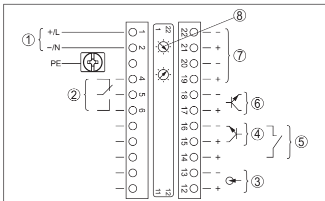
Fig. 16: Elektronica- en aansluitruimte (Ex d) bij instrumenten met intrinsiekveilige stroomuitgang
