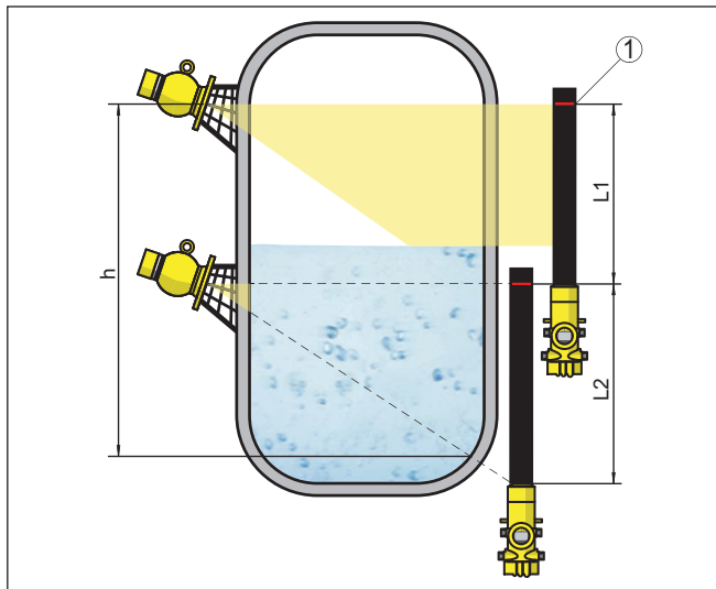
Fig. 7: Inbouwpositie - cascade opstelling
