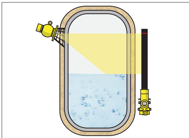
Fig. 8: Niveaumeting aan een verwarmde tank met warmte-isolatie
