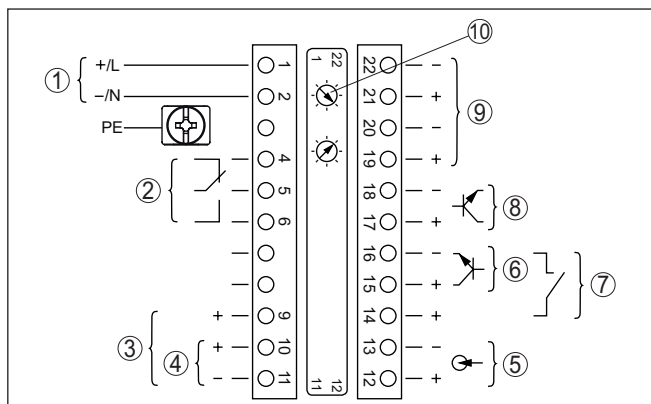
插图. 11: 非防爆仪表和带有非自安全电流输出出口的仪表上的电子部件和接线腔
