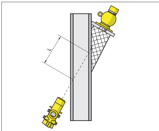
插图. 21: 斜向安装时适用管件的辐照长度
