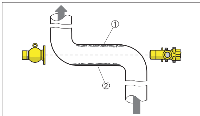
插图. 5: 安装在一根水平管道上
