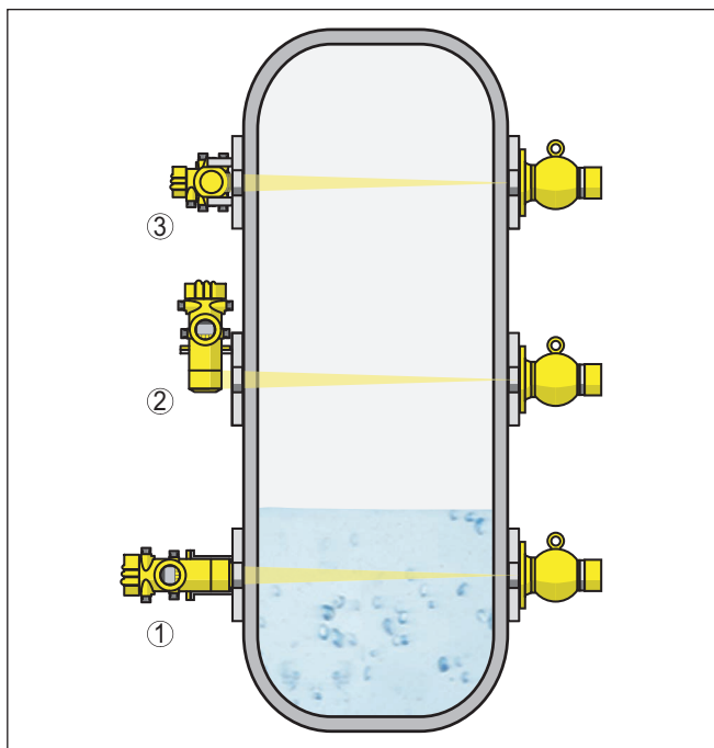
插图. 8: 安装位置 - 极限液位测量
