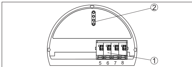
插图. 12: 非防爆仪表和带有非安全电流输出出口的仪表上的操作和接线腔
