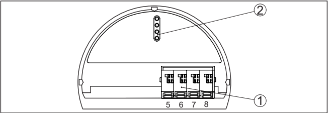
插图. 16: 非防爆仪表和带有非安全电流输出出口的仪表上的操作和接线腔
