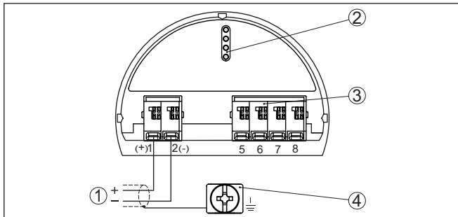
插图. 14: 在带有自安全电流输出出口的仪表上的操作和接线腔 (防爆 ia)
