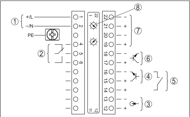
插图. 17: 在带有自安全电流输出出口的仪表上的电子部件和接线腔 (防爆 (d))
