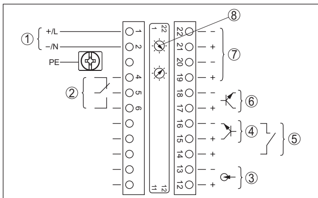
插图. 13: 在带有安全电流输出出口的仪表上的电子部件和接线腔 (防爆 (d))
