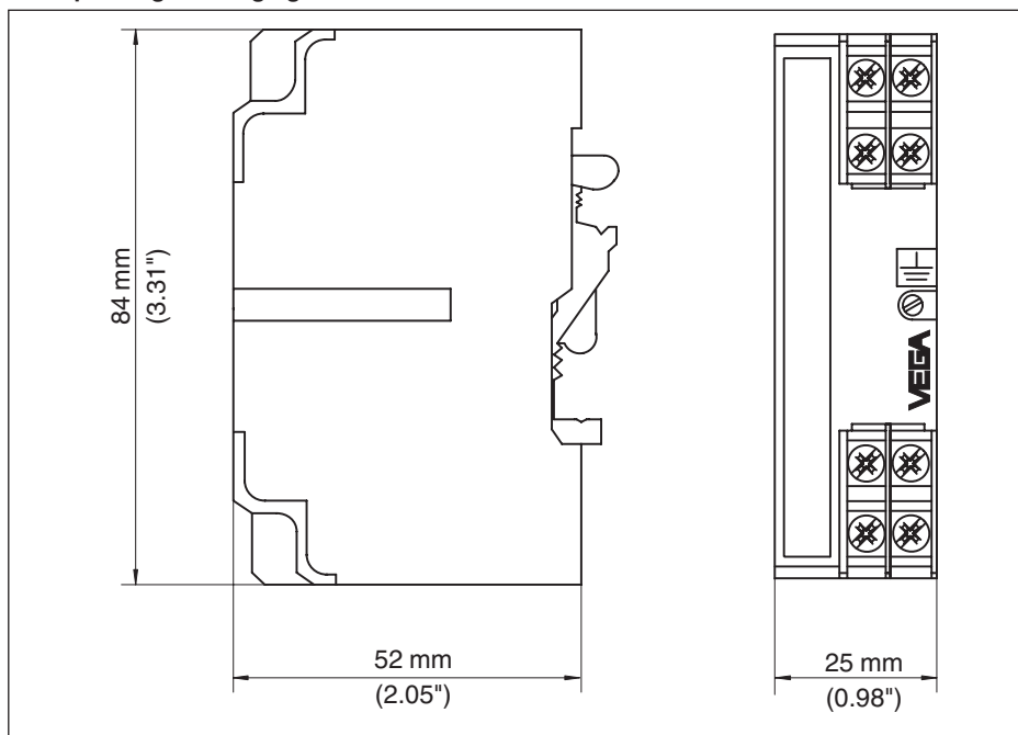
Fig. 10: Afmetingen B53-19
