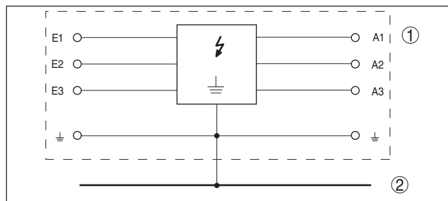
Fig. 7: Principeschakelschema B53-19
