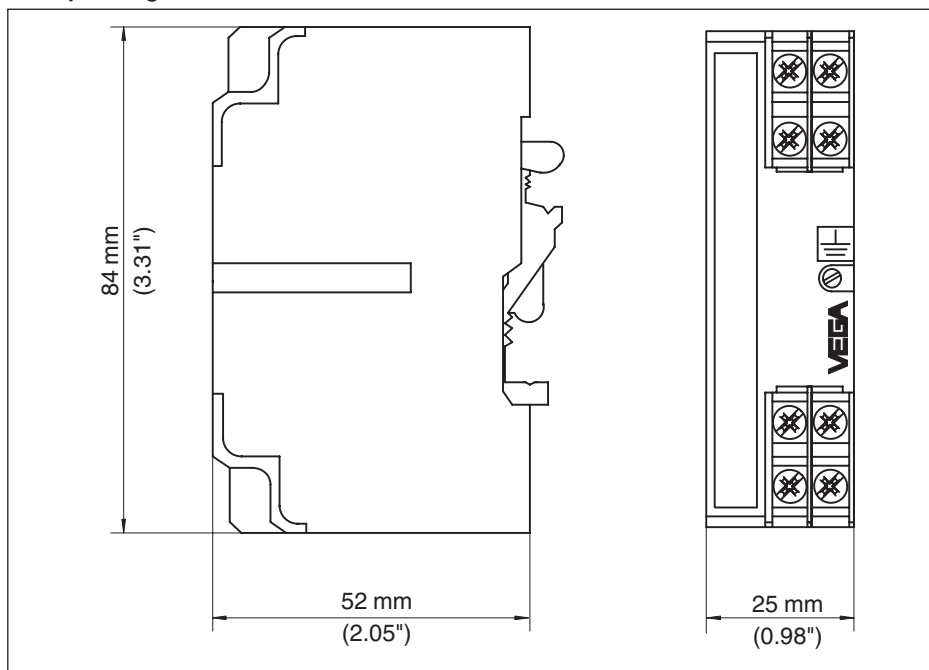
Abb. 10: Maße B62-36G
