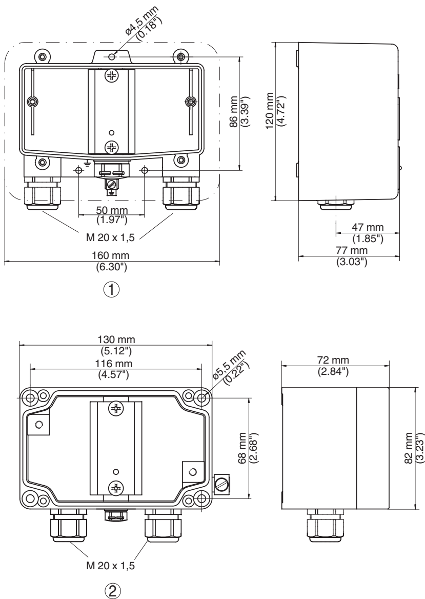
Abb. 11: Maße B62-36G
