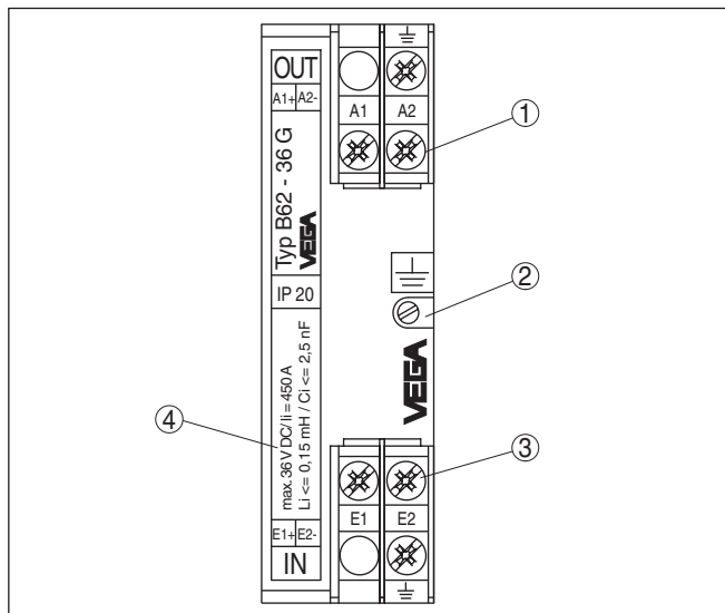
Abb. 1: Aufbau des B62-36G
