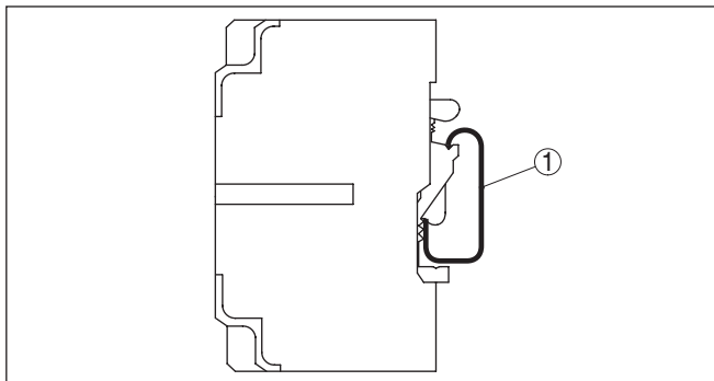
Abb. 3: Montage auf Tragschiene nach EN 50 035 (C-Schiene) 35 \times 7,5 \text{ mm} 1 Tragschiene
