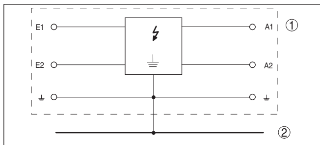
Abb. 7: Prinzipschaltbild B62-36G
