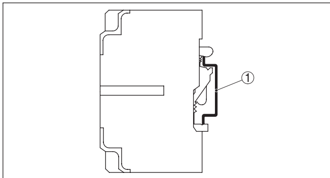
Abb. 2: Montage auf Tragschiene nach EN 50 022 (Hutschiene) 35 \times 7,5 \text{ mm} 1 Tragschiene
