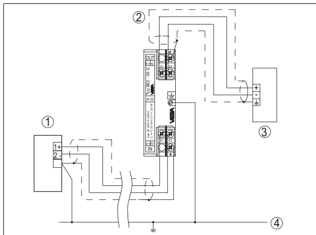
Abb. 9: Anschlussplan B62-36G - Steuergeräteschutz (Nicht-Ex-Anwendungen)
