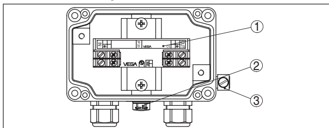
Abb. 5: Montage im Aluminium-Gehäuse
