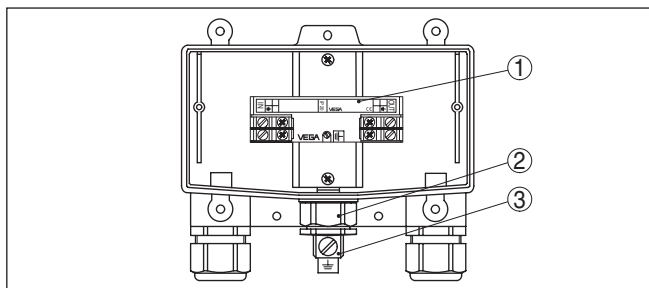
Abb. 6: Montage im Kunststoffgehäuse
