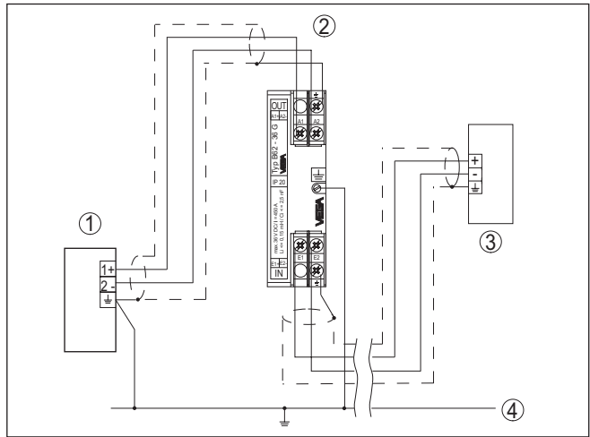
Abb. 8: Anschlussplan B62-36G - Sensorschutz (Nicht-Ex-Anwendungen)
