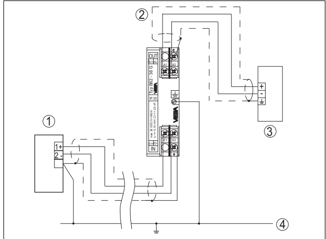
Abb. 9: Anschlussplan B62-36G - Steuergeräteschutz (Nicht-Ex-Anwendungen)
