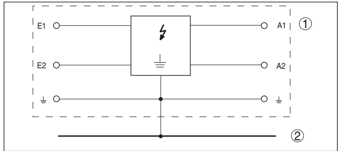
Abb. 7: Prinzipschaltbild B62-36G
