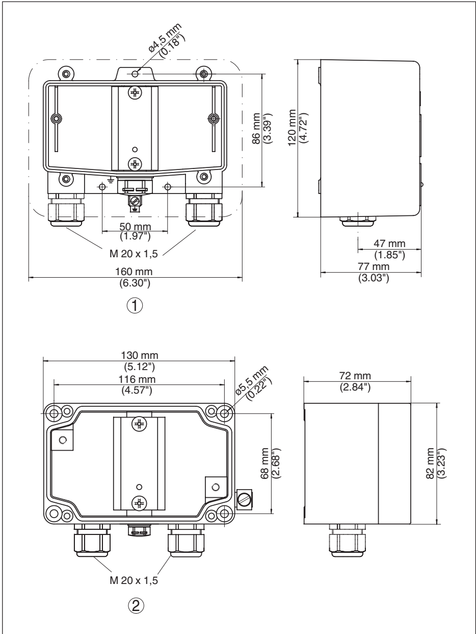
Abb. 11: Maße B62-36G
