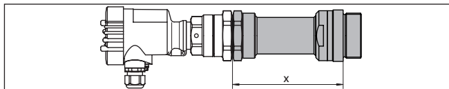
Abb. 4: VEGAMIP 61 mit Montageadapter "Hochtemperatur" -40 ... +450 °C (-40 ... +842 °F)
