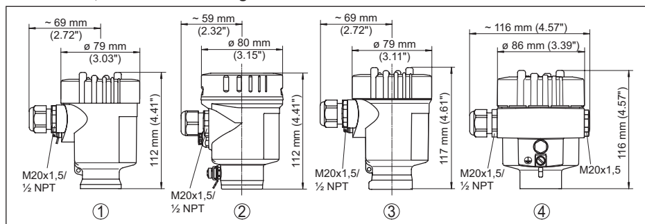
Abb. 29: Gehäuseausführungen
