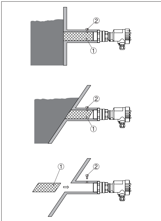
Abb. 12: Frontbündige Montage
