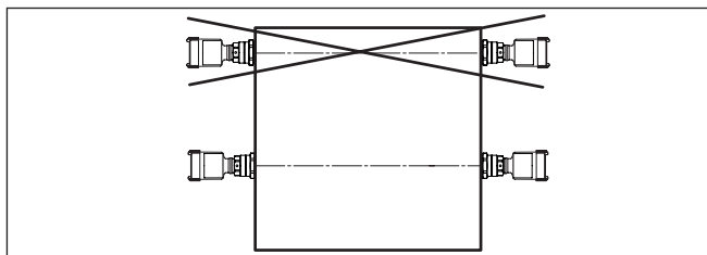
Abb. 6: Einbauposition (Draufsicht)
