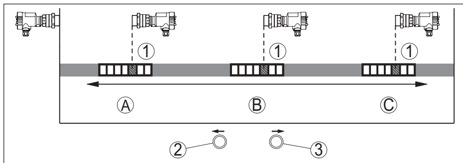
Abb. 25: Anzeigeleiste
