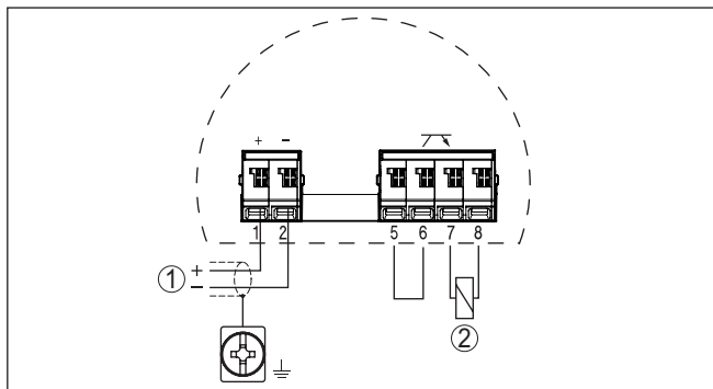
Abb. 21: Anschlussplan Empfängereinheit - VEGAMIP 61 (Receiver) - PNP-Verhalten
