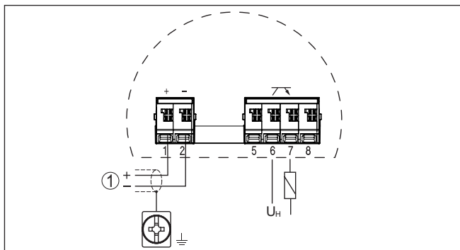
Abb. 23: Anschlussplan Empfängereinheit - VEGAMIP 61 (Receiver) - Potenzialfrei
