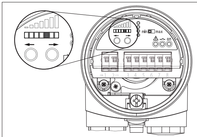
Abb. 27: LED-Anzeigeleiste - Einstellung für Füllgüter mit geringer Signaldämpfung
