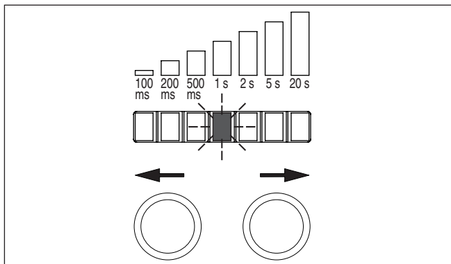
Abb. 28: Schaltverzögerung einstellen - LED-Anzeige blinkt
