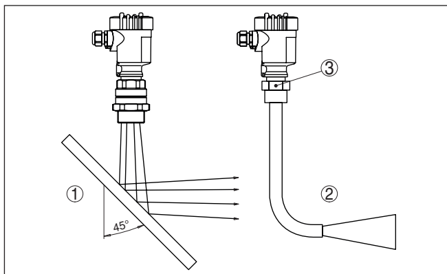
Abb. 19: Möglichkeiten zur Signalumlenkung
