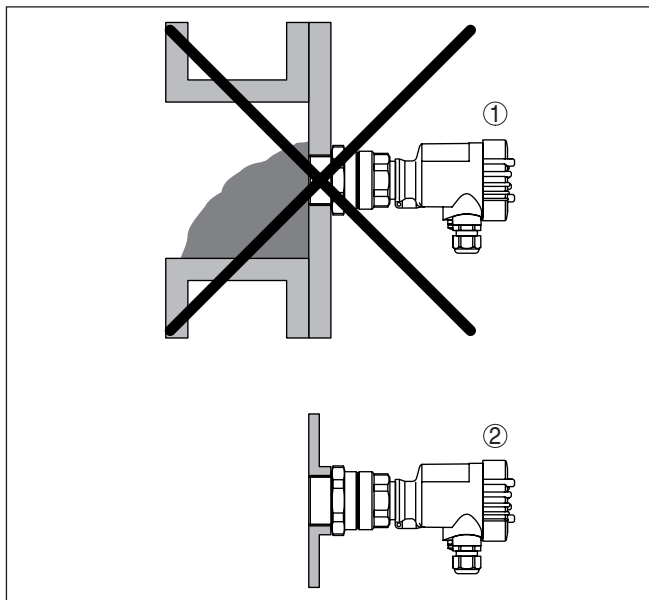
Abb. 11: Frontbündige Montage
