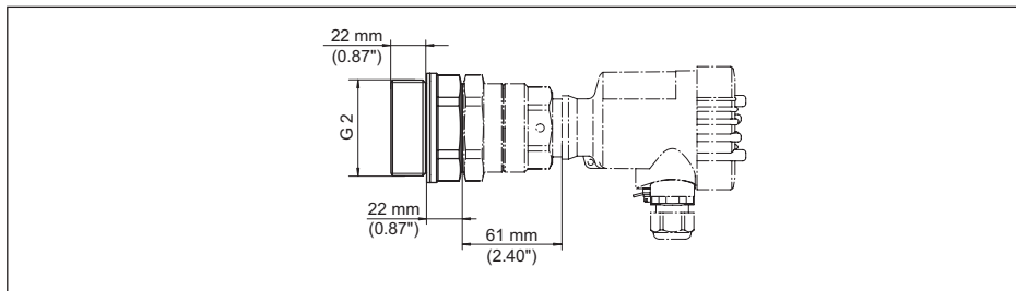
Abb. 33: Montageadapter mit Keramikabdeckung (optional) für VEGAMIP 61 mit innenliegender Hornantenne, Gewindeausführung G1½ mit PTFE-Abdeckung (auch mit 1½ NPT-Gewinde)
