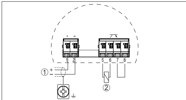
Abb. 22: Anschlussplan Empfängereinheit - VEGAMIP 61 (Receiver) - NPN-Verhalten
