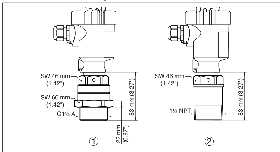
Abb. 30: VEGAMIP 61, innenliegende Hornantenne (Gewindeausführung)
