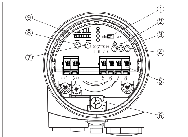
Abb. 24: Elektronikeinsatz MP6X S (Empfängereinheit) - Transistorausgang
