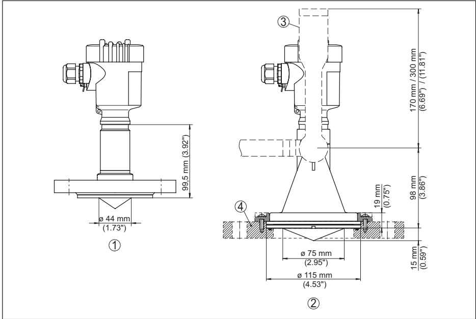
Abb. 31: VEGAMIP 61, gekapselte Antennen
