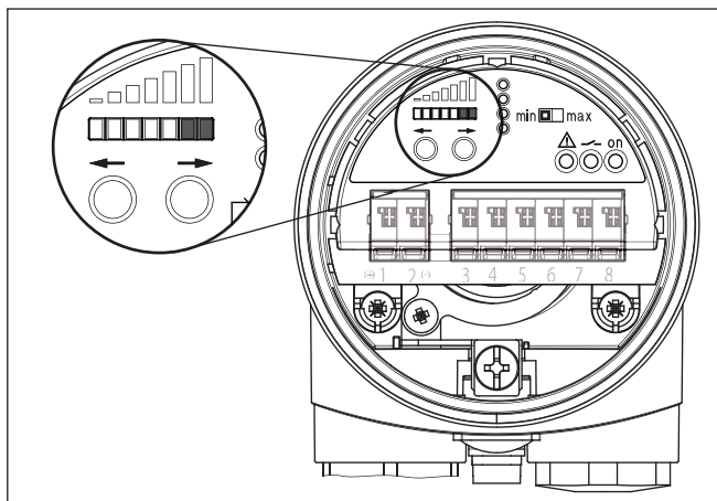
Abb. 26: LED-Anzeigeleiste - Einstellung für Füllgüter mit guter Signaldämpfung
