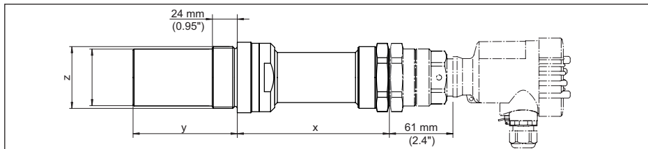
Abb. 35: Montageadapter mit Tubus (optional) für frontbündige Montage, für VEGAMIP 61 mit innenliegender Hornantenne, Gewindeausführung G1½ mit PTFE-Abdeckung (auch mit 1½ NPT-Gewinde)
