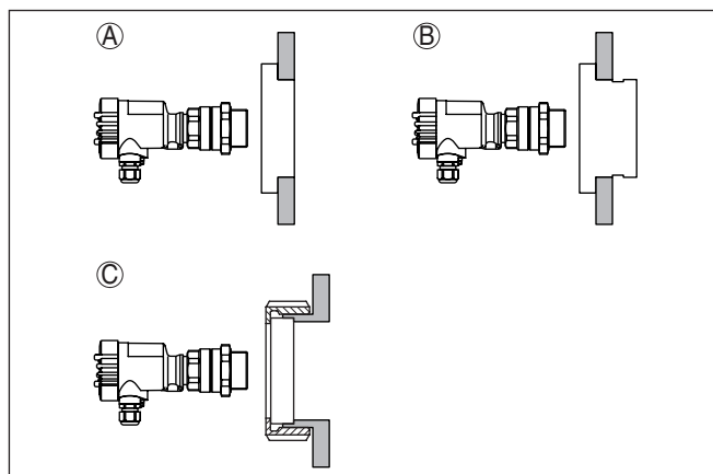
Abb. 8: Einbau vor einem Behälterfenster
