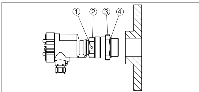
Abb. 10: VEGAMIP 61, Gewindeausführung G1½
