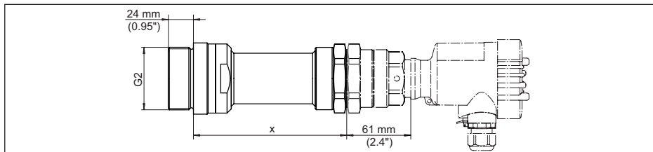
Abb. 34: Montageadapter mit Keramikabdeckung (optional) für VEGAMIP 61 mit innenliegender Hornantenne, Gewindeausführung G1½ mit PTFE-Abdeckung (auch mit 1½ NPT-Gewinde)
