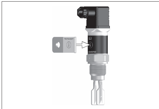
Fig. 13: Simulation du signal de sortie
