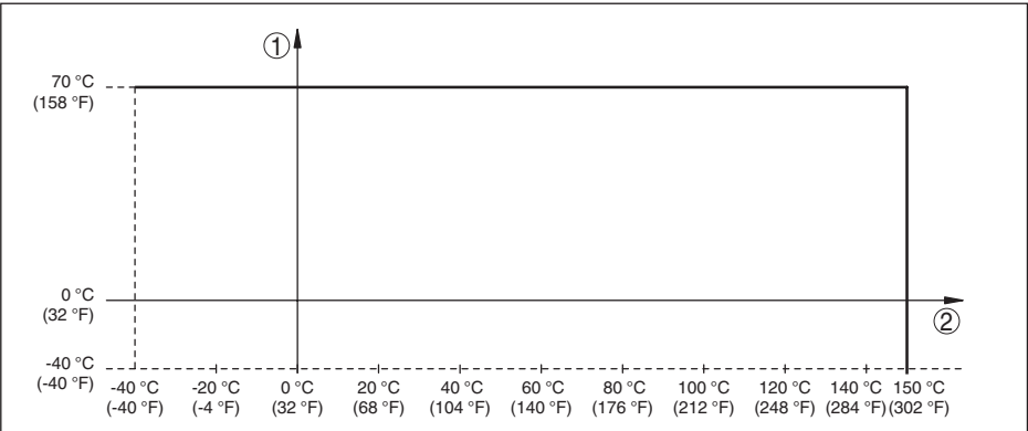
Fig. 15: Dépendance entre température ambiante et température du process
