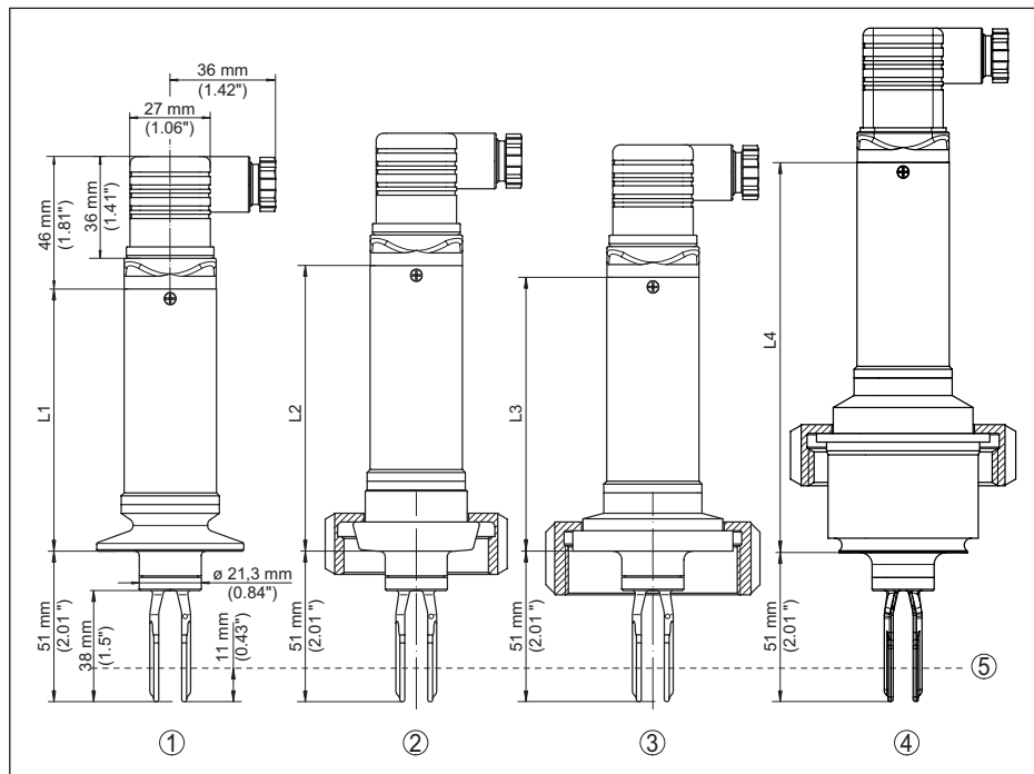
Fig. 18: VEGASWING 51, version alimentaire - raccords hygiéniques
