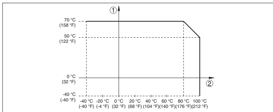
Fig. 14: Dépendance entre température ambiante et température du process
