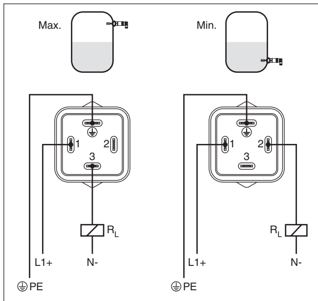
Fig. 12: Schéma de raccordement, sortie statique pour connecteur type électrovanne ISO 4400
