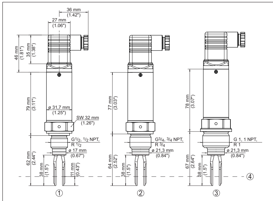
Fig. 17: VEGASWING 51, version haute température - raccords filetés
