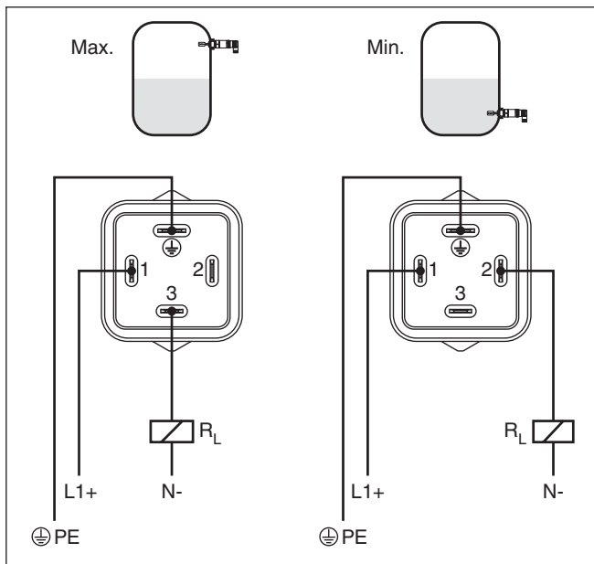
Fig. 12: Aansluitschema, contactloze schakelaar bij ventielconnector ISO 4400
