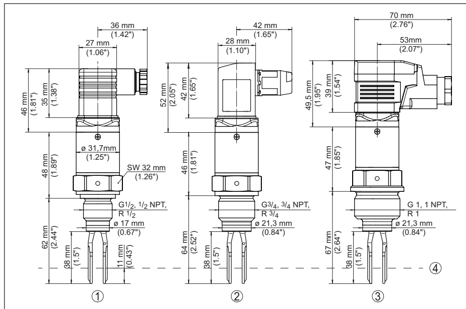
Fig. 16: VEGASWING 51, standaard uitvoering - schroefdraadaansluiting
