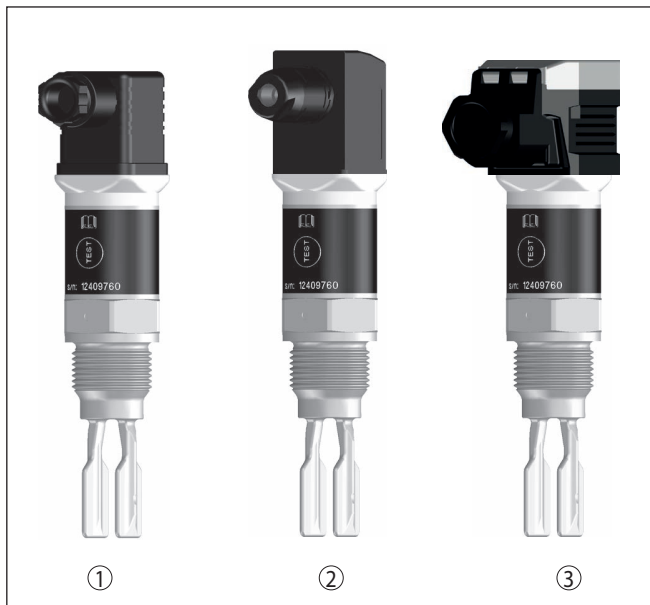
Fig. 7: Overzicht aansluitvarianten
