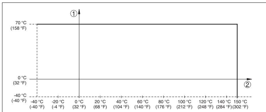
Fig. 15: Afhangelijkheid omgevingstemperatuur van procestemperatuur
