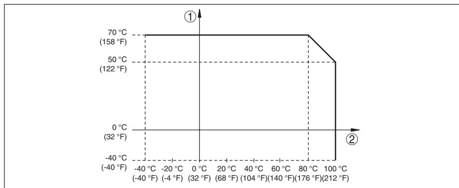
Fig. 14: Afhangelijkheid omgevingstemperatuur van processtemperatuur
