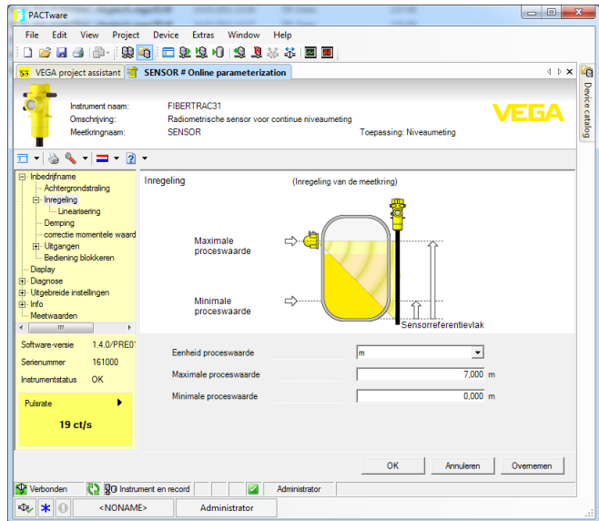
Fig. 22: Voorbeeld van een DTM-aanzicht
