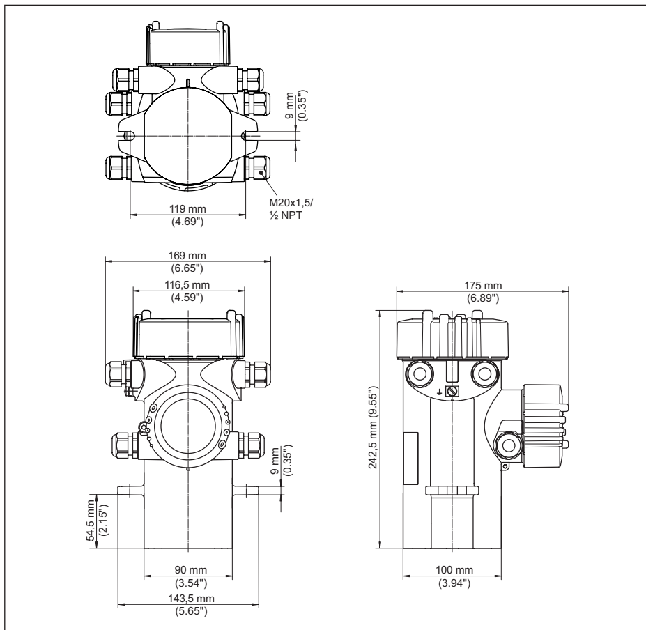
Fig. 26: Aluminium behuizing resp. rvs-behuizing (fijnnetwerk)
