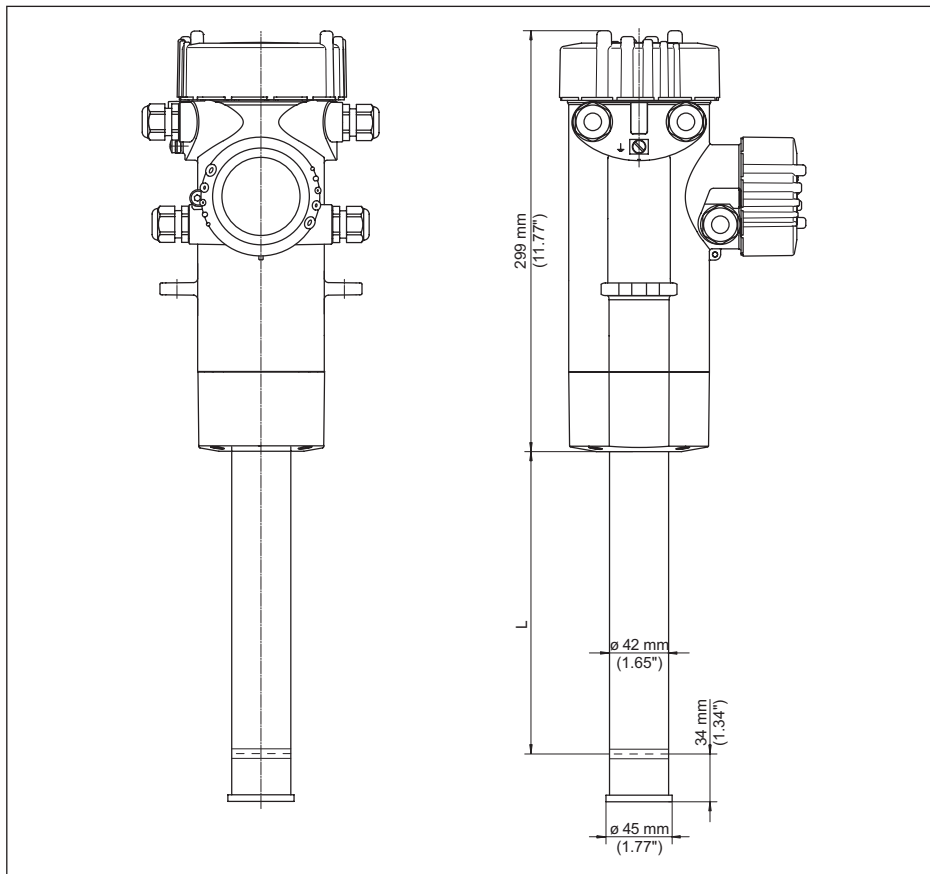
Fig. 27: FIBERTRAC 31
