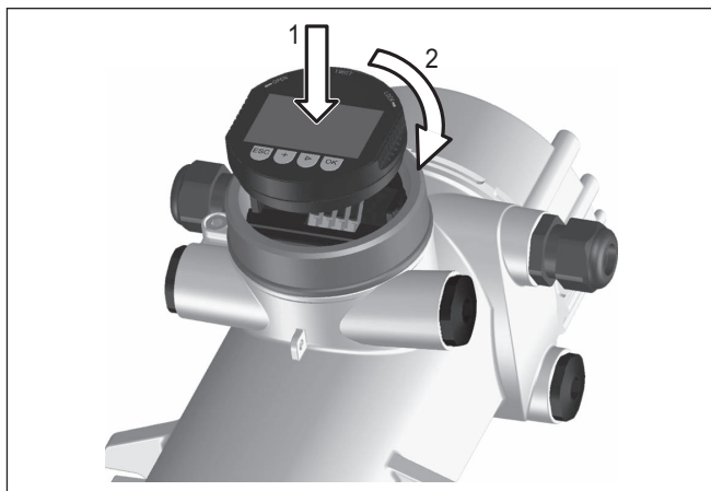
Fig. 19: Insertion du module de réglage et d'affichage
