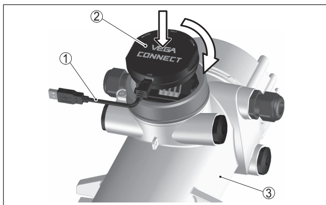
Fig. 22: Raccordement du PC directement au capteur via l'adaptateur d'interfaces
