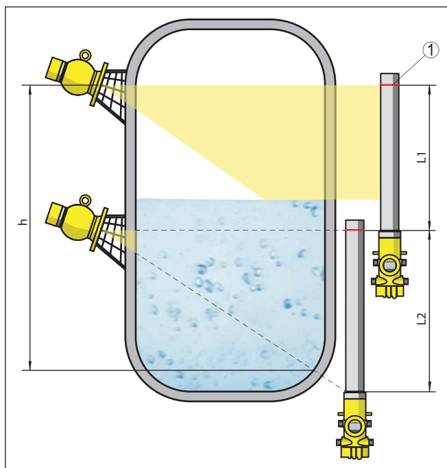
Fig. 7: Position de montage - Agencement en cascade
