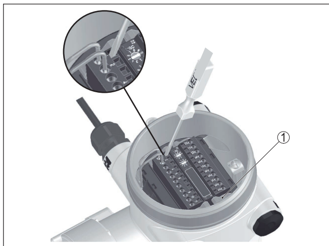
Fig. 9: Étapes de raccordement 4 et 5
