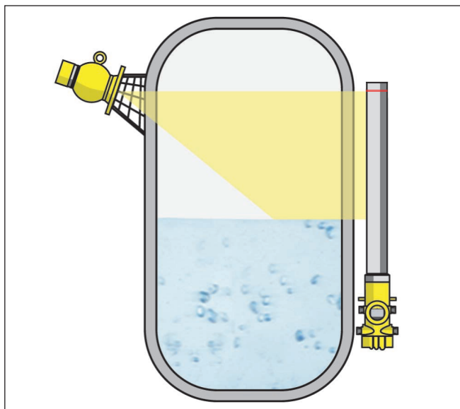
Fig. 5: Mesure de niveau dans une cuve de stockage
