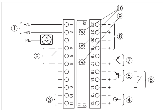
Fig. 10: Compartiment électronique et de raccordement des appareils non Ex et appareils avec sortie signal pas à sécurité intrinsèque
