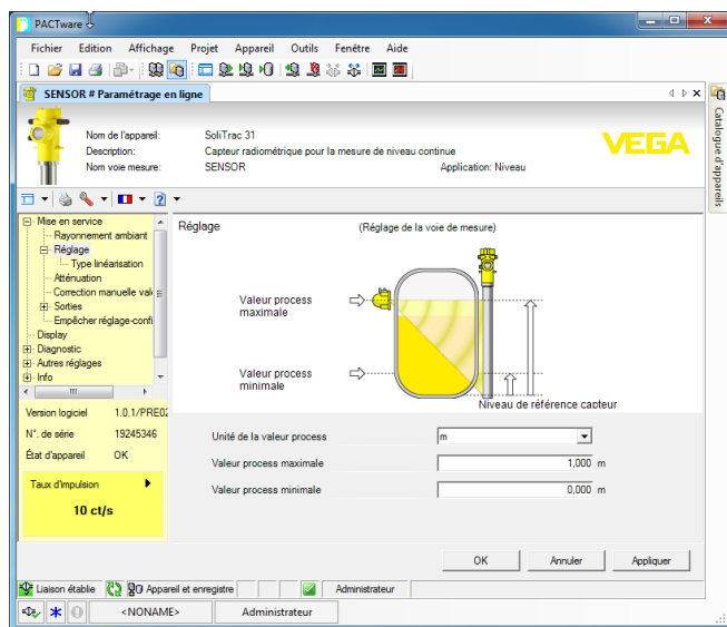
Fig. 23: Exemple de masque DTM
