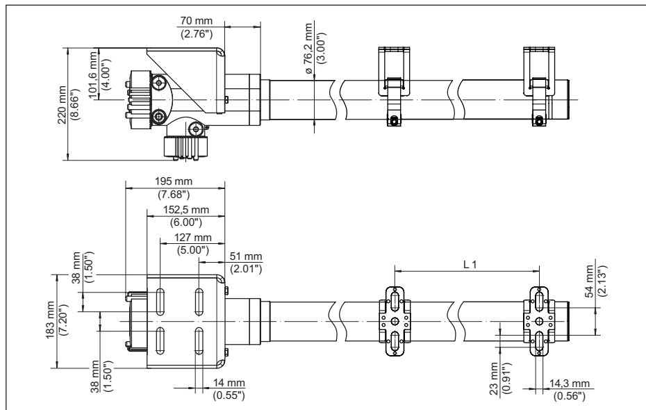
Fig. 28: SOLITRAC 31 avec des accessoires de montage compris à la livraison
