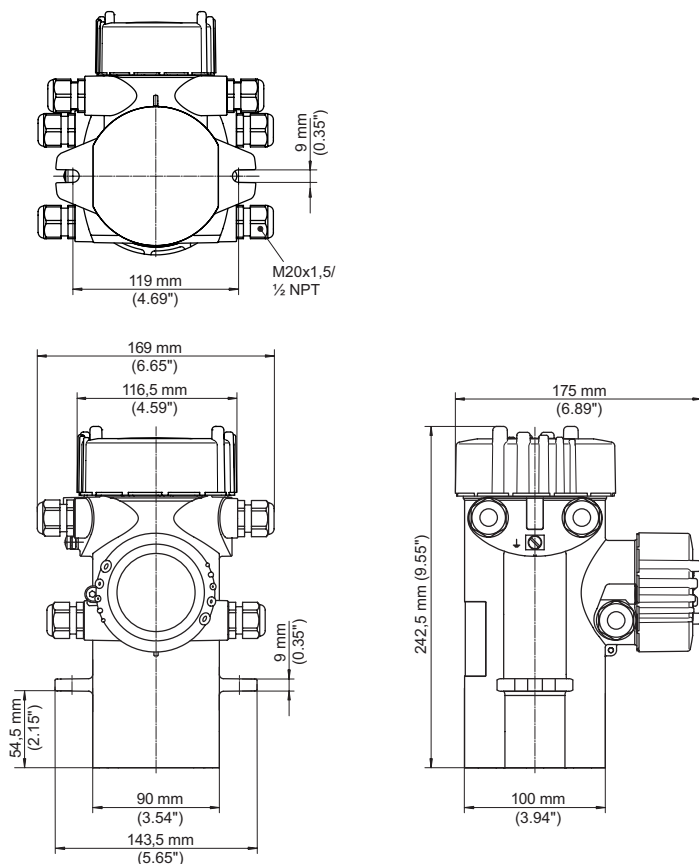
Fig. 26: Boîtier en aluminium ou boîtier en acier inox (moulage cire-perdue)
