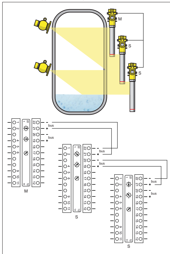
Fig. 18: Compartiment électronique et de raccordement pour le montage en cascade de plusieurs appareils.
