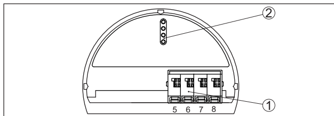
Fig. 11: Compartiment de réglage et de raccordement des appareils non Ex et appareils avec sortie signal pas à sécurité intrinsèque
