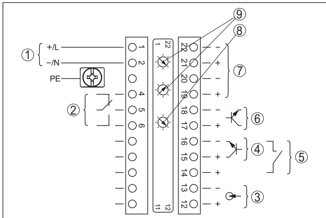
Fig. 12: Compartiment électronique et de raccordement (Ex d) des appareils avec sortie signal à sécurité intrinsèque
