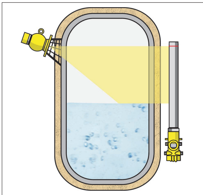
Fig. 8: Mesure de niveau dans un réservoir chauffé avec isolation thermique
