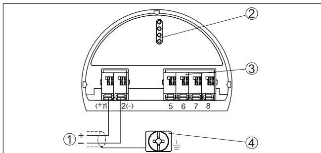
Fig. 13: Compartiment de réglage et de raccordement (Ex ia) des appareils avec sortie signal à sécurité intrinsèque
