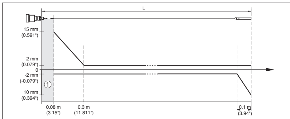
插图. 39: 绳型 VEGAFLEX 81 在介质“水”中的测量偏差
