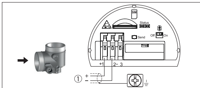
插图. 17: 接线腔 - 无线模块 PLICSMOBILE 81
