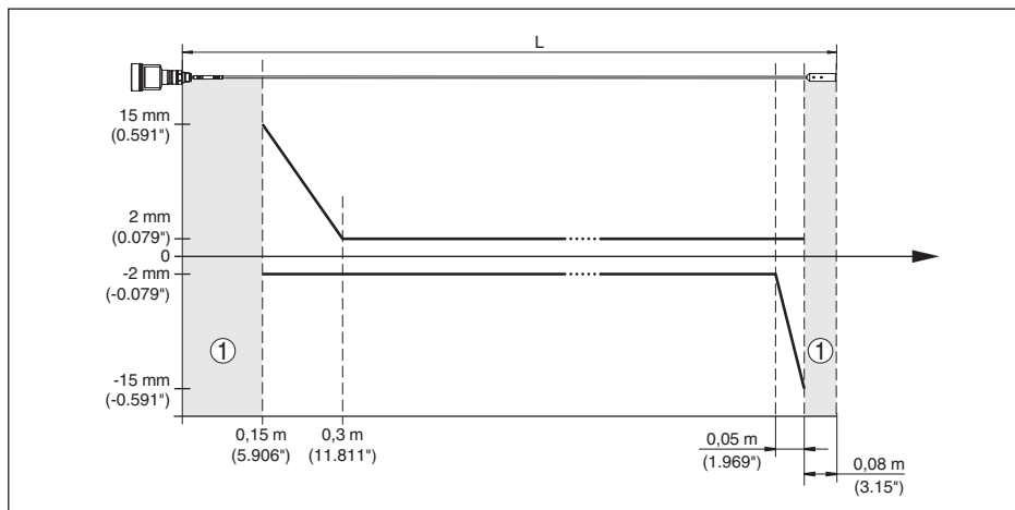
插图. 40: 绳型 (ø 2 mm/0.079 in) VEGAFLEX 81 在介质“油”中的测量偏差
