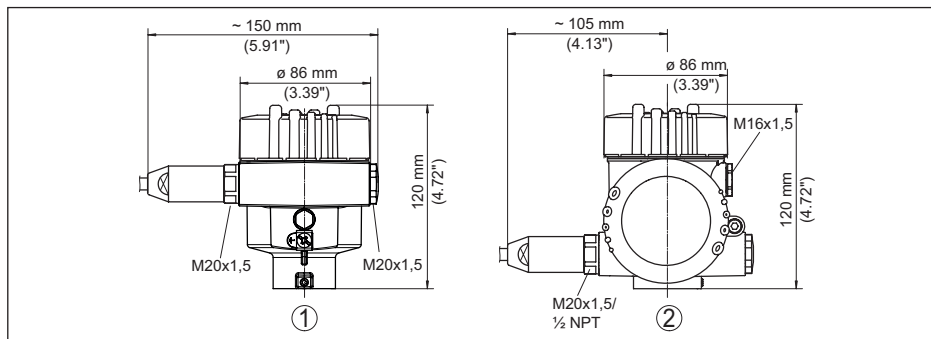
插图. 48: 采用保护等级达 IP66/IP68 (1 bar) 的壳体型式, (内装显示和调整模块后, 壳体高度增加了 9 mm/0.35 in)
