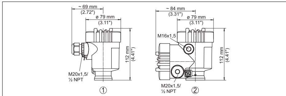
插图. 46: 采用防护等级为 IP66/IP67 的外壳版本 (内装显示和调整模块后, 外壳高度增加了 9 mm/0.35 in)
