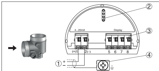
插图. 16: 双腔式外壳的接线腔
