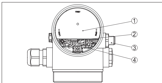
插图. 20: 目检带有与外部显示和调整单元相连接的 VEGADIS-Adapter 的电子部件腔
