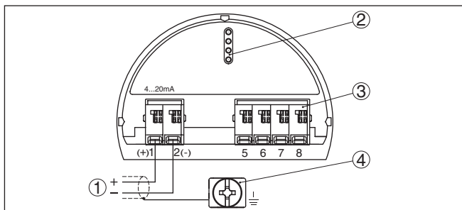
插图. 14: 单腔式外壳的电子部件和接线腔
