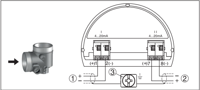
插图. 23: 双腔式外壳的接线腔，附加电子部件 " 额外的电流输出"
