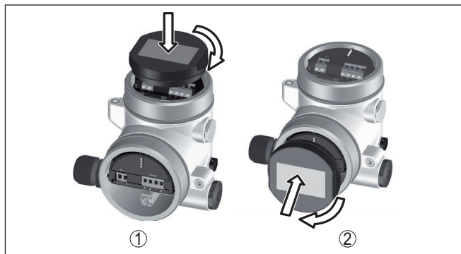
插图. 25: 将显示和调整模块装到双腔式壳体上
