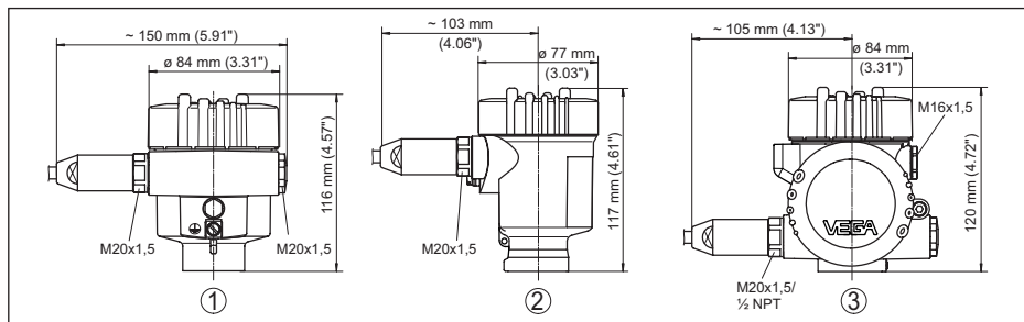
插图. 50: 采用保护等级达 IP66/IP68 (1 bar) 的壳体型式. (内装显示和调整模块后, 壳体高度增加了 9 mm/0.35 in)
