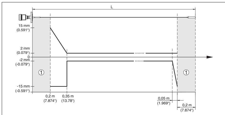
插图. 43: 在介质油中, 绳型 VEGAFLEX 81 (ø 4 mm/0.157 in, 经 PFA 涂层) 的测量偏差
