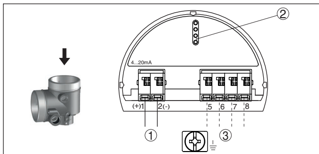
插图. 18: 防爆 (d-ia) 型双腔式外壳的电子部件腔
