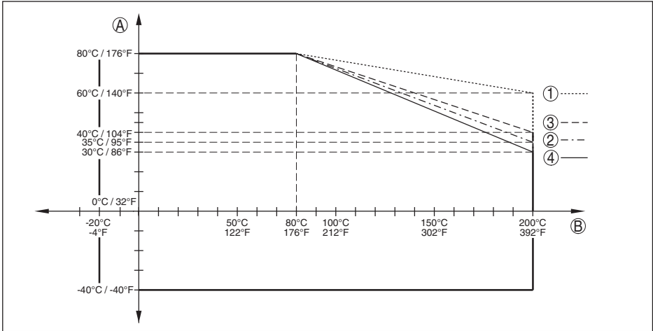
插图. 45: 环境温度 - 过程温度、带有温度连接元件的选型
