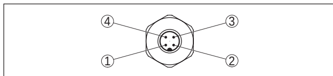
插图. 21: 察看 M12 x 1-连接器
