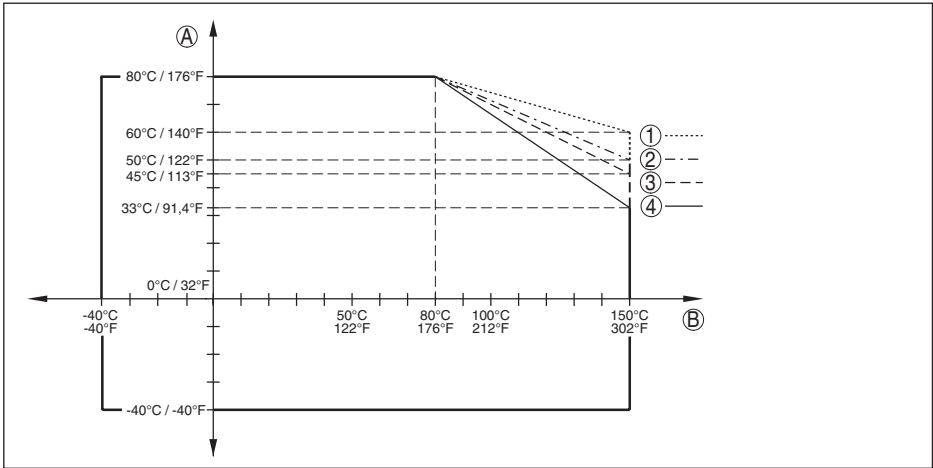
插图. 44: 环境温度 - 过程温度, 标准型
