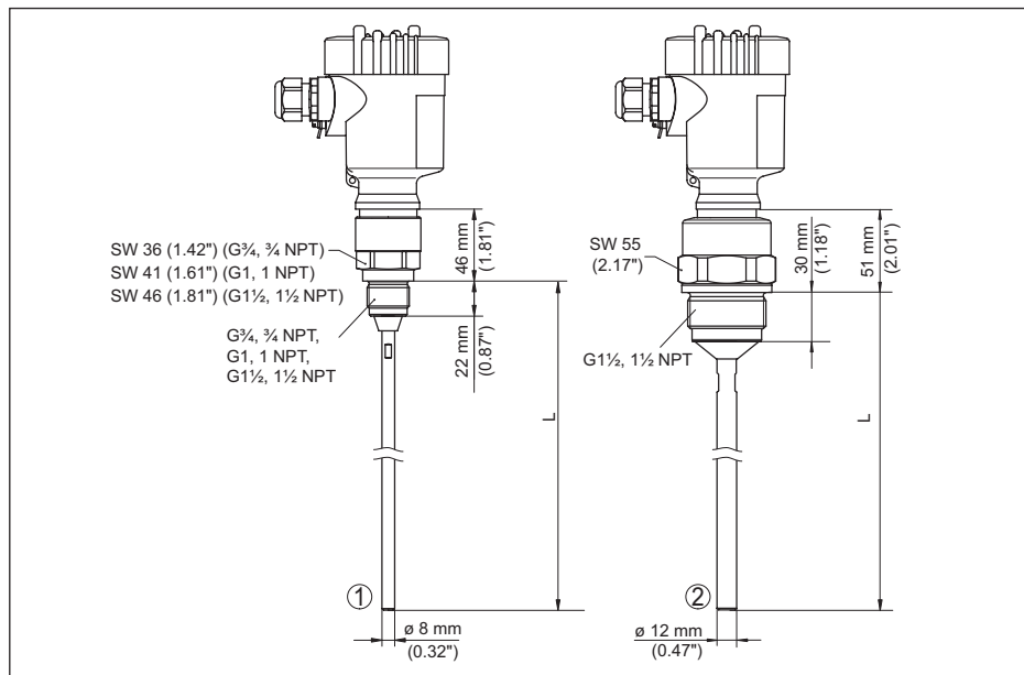
插图. 53: VEGAFLEX 81, 螺纹型
