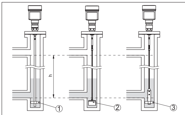
插图. 9: 安装在一根旁路管中 - 星形对中垫片或定心锤的位置
