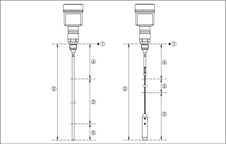
插图. 36: VEGAFLEX 81 的量程
