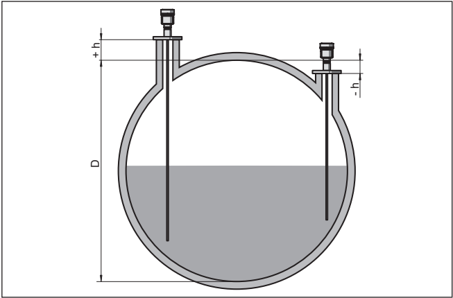
插图. 27: 容器高度和管接头修正值
