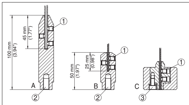
插图. 35: 截短绳型测量探头
