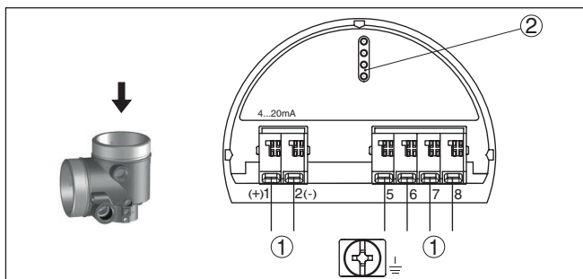
插图. 15: 双腔式外壳的电子部件腔
