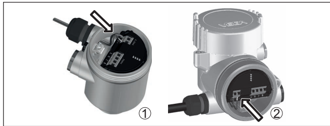
插图. 13: 接线步骤5和6
