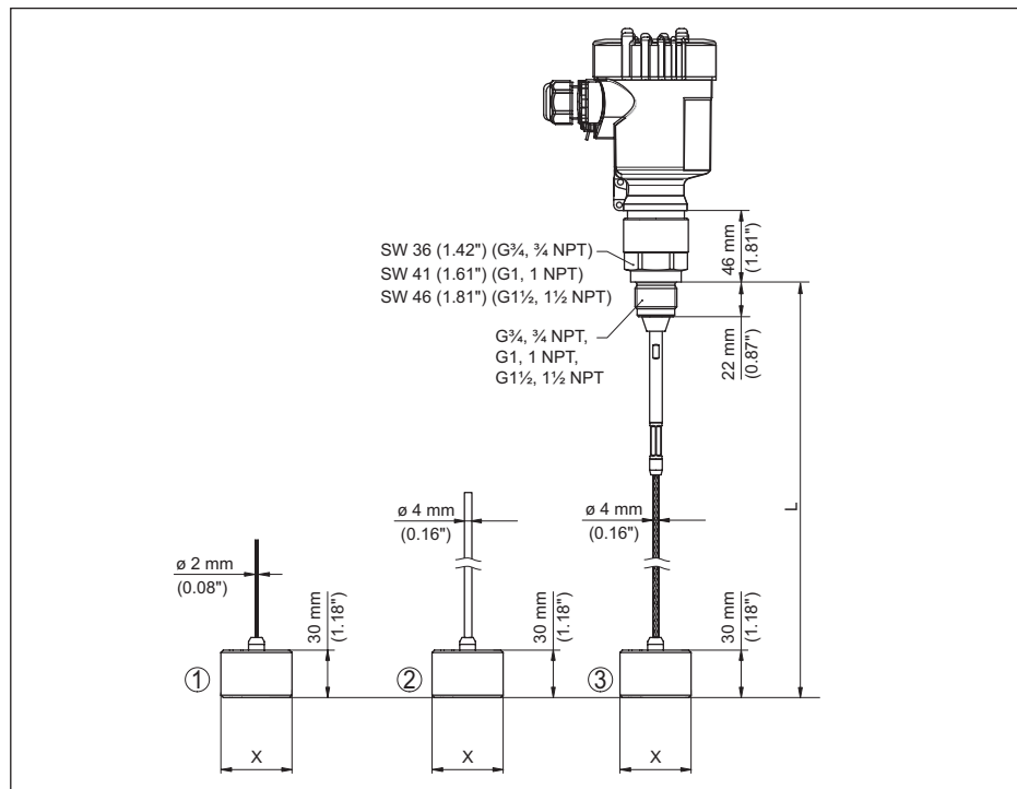
插图. 52: VEGAFLEX 81, 螺纹型
