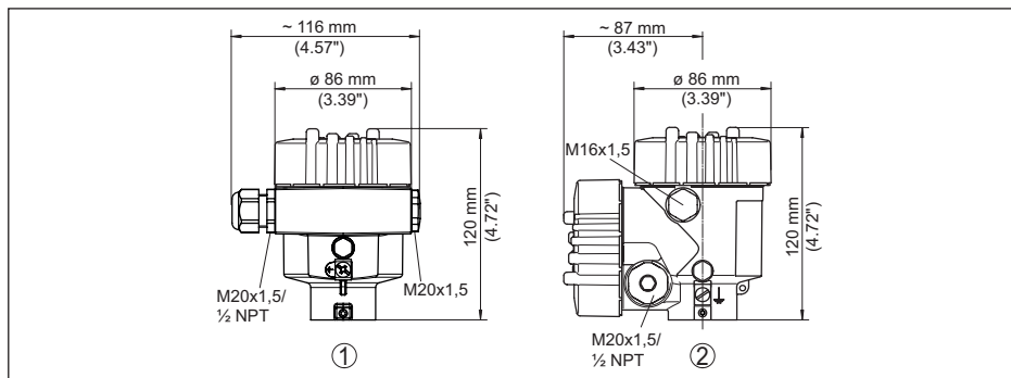
插图. 47: 采用防护等级达 IP66/IP68 (0.2 bar) 的壳体版本, (内装显示和调整模块后, 壳体高度增加了 9 mm/0.35 in)
