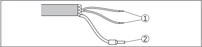
插图. 22: 固定连接的连接电缆的芯线分布
