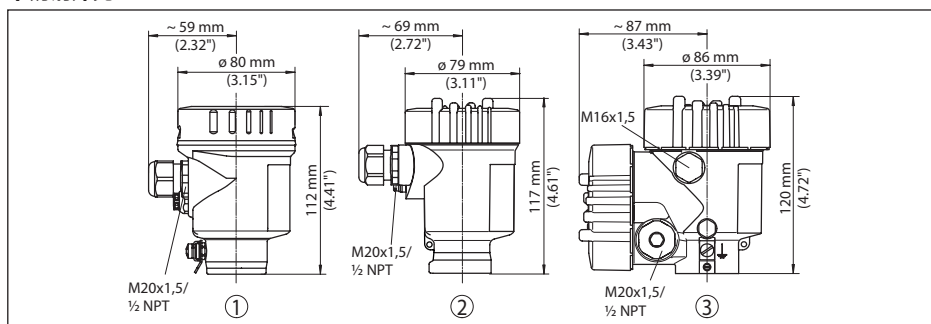
插图. 49: 采用防护等级达 IP66/IP68 (0.2 bar) 的壳体版本, (内装显示和调整模块后, 壳体高度增加了 9 mm/0.35 in)
