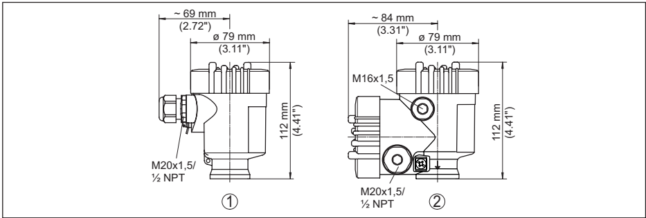
Fig. 48: Variantes de boîtier en protection IP66/IP67 (avec un module de réglage et d'affichage intégré, la hauteur du boîtier augmente de 9 mm/0.35 in)
