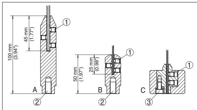
Fig. 37: Raccourcir le câble de la sonde
