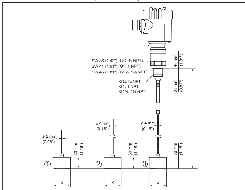
Fig. 54: VEGAFLEX 81, version filetée
