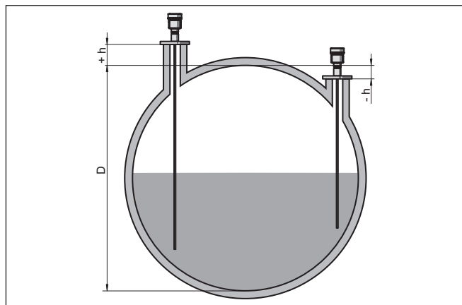
Fig. 27: Hauteur de la cuve et valeur de correction du manchon
