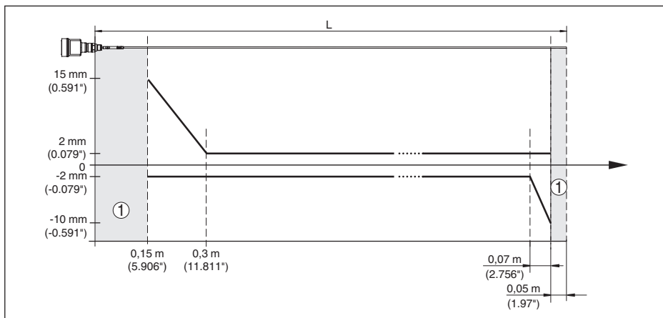
Fig. 40: Écart de mesure VEGAFLEX 81 en version tige dans l'huile
