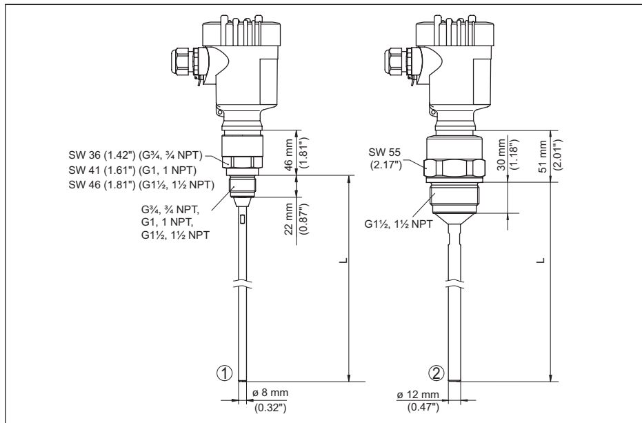
Fig. 55: VEGAFLEX 81, version fileté
