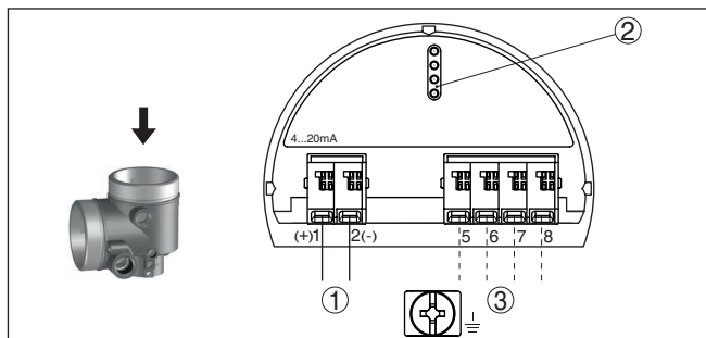
Fig. 17: Compartiment électronique - boîtier à deux chambres Ex d ia
