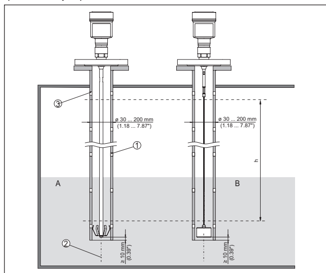
Fig. 9: Montage dans un tube tranquillisateur
