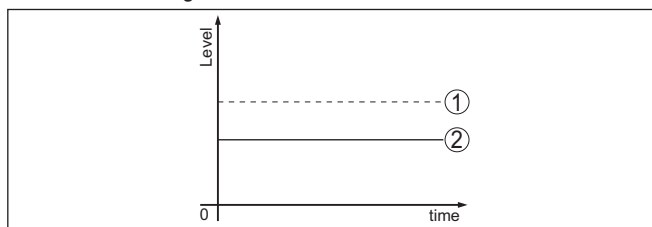
Fig. 35: La ligne en pointillés 1 montre le niveau réel, la ligne continue 2 montre le niveau indiqué par le capteur.
