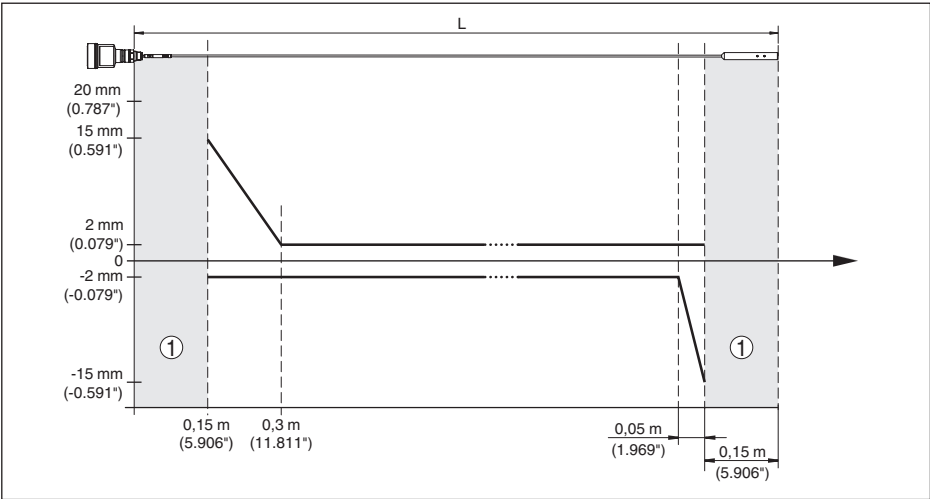
Fig. 43: Écart de mesure VEGAFLEX 81 en version câble (ø 4 mm/0.157 in), dans l'huile
