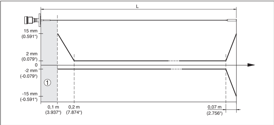
Fig. 44: Écart de mesure VEGAFLEX 81 en version câble (ø 4 mm/0.157 in, revêtu PFA) dans le produit Eau
