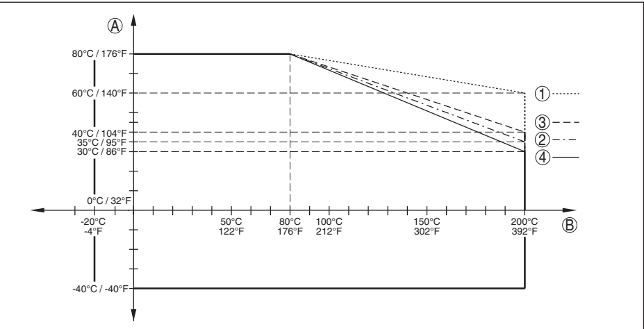
Fig. 47: Température ambiante - température process, version avec extension haute température
