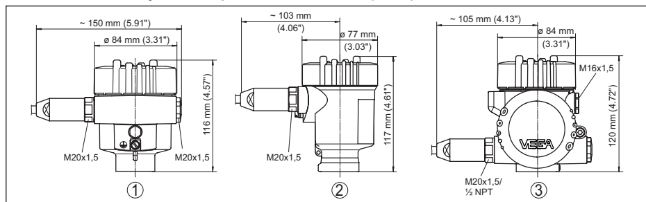
Fig. 52: Variantes de boîtier en protection IP66/IP68 (1 bar), (avec un module de réglage et d'affichage intégré, la hauteur du boîtier augmente de 9 mm/0.35 in)
