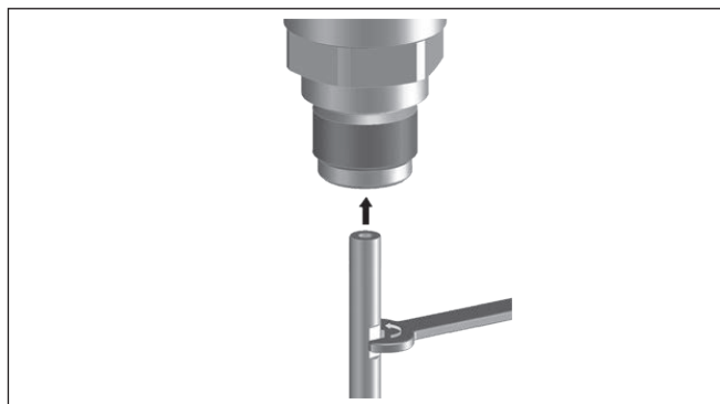
Fig. 36: Changer le câble de mesure ou la tige de mesure
