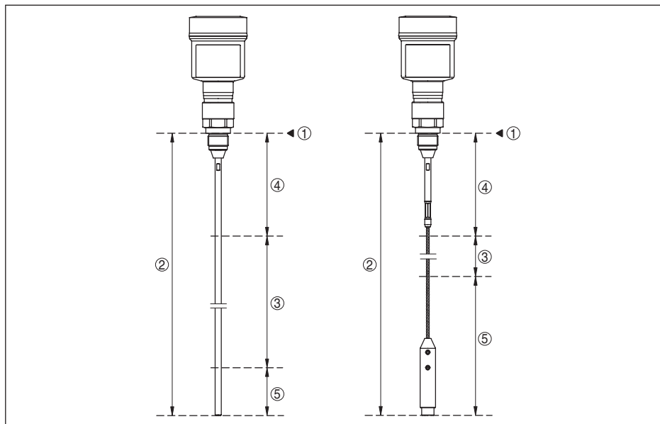
Fig. 38: Plages de mesure - VEGAFLEX 81
