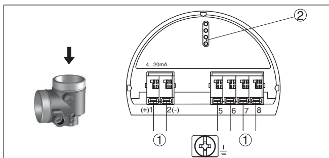
Fig. 14: Compartiment électronique - boîtier à deux chambres
