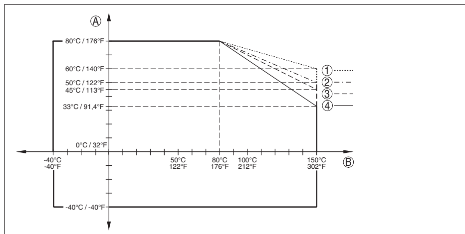
Fig. 46: Température ambiante - température process, version standard
