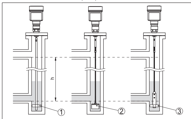
Fig. 8: Montage dans un tube bypass - Position de l'étoile de centrage ou du poids de centrage
