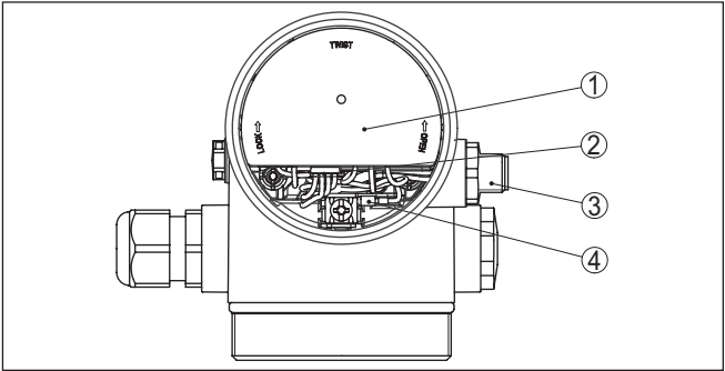
Abb. 17: Sicht auf den Elektronikraum mit VEGADIS-Adapter zum Anschluss der externen Anzeige- und Bedieneinheit
