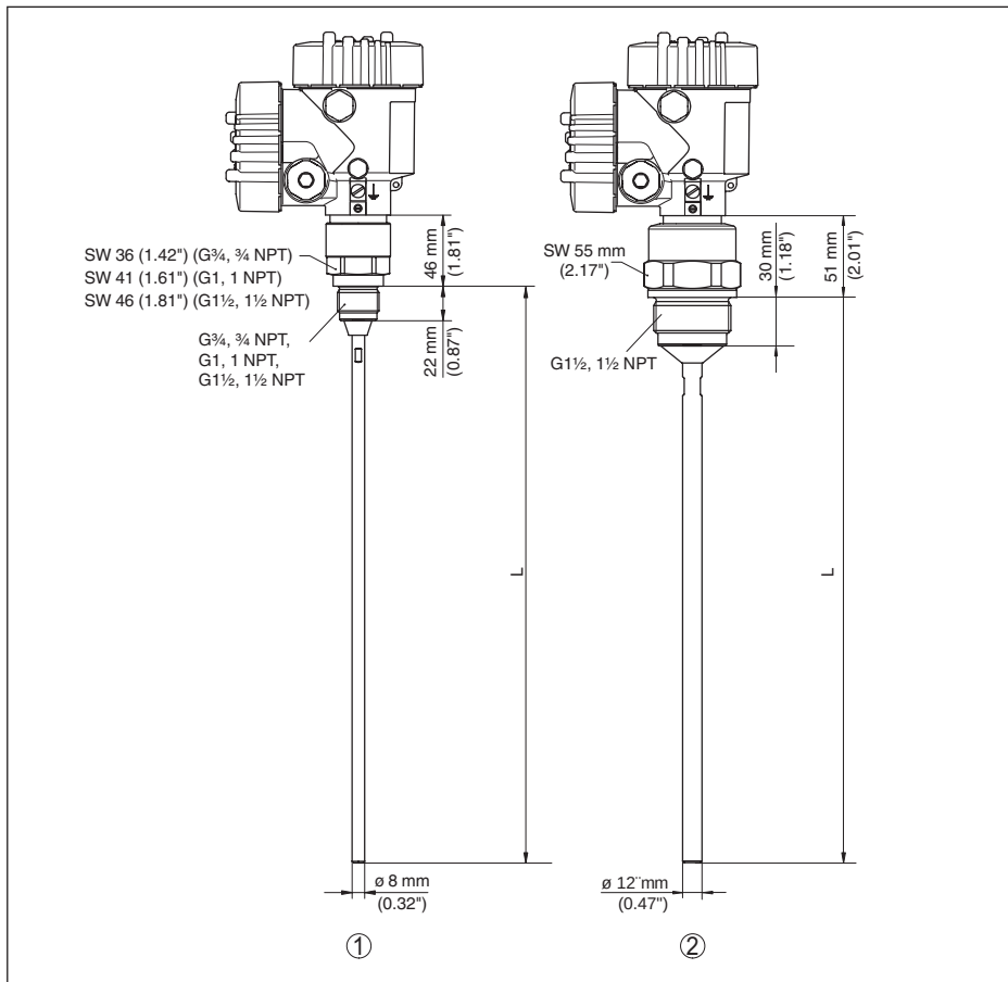
Abb. 43: VEGAFLEX 81, Gewindeausführung
