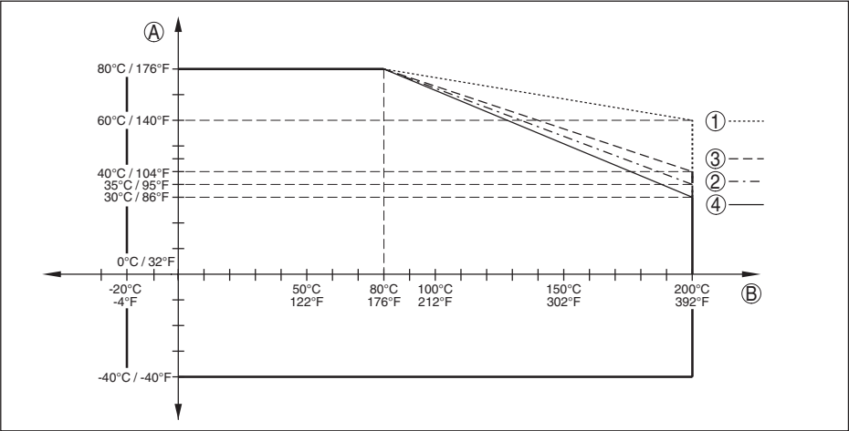
Abb. 39: Umgebungstemperatur - Prozesstemperatur, Ausführung mit Temperaturzwischenstück
