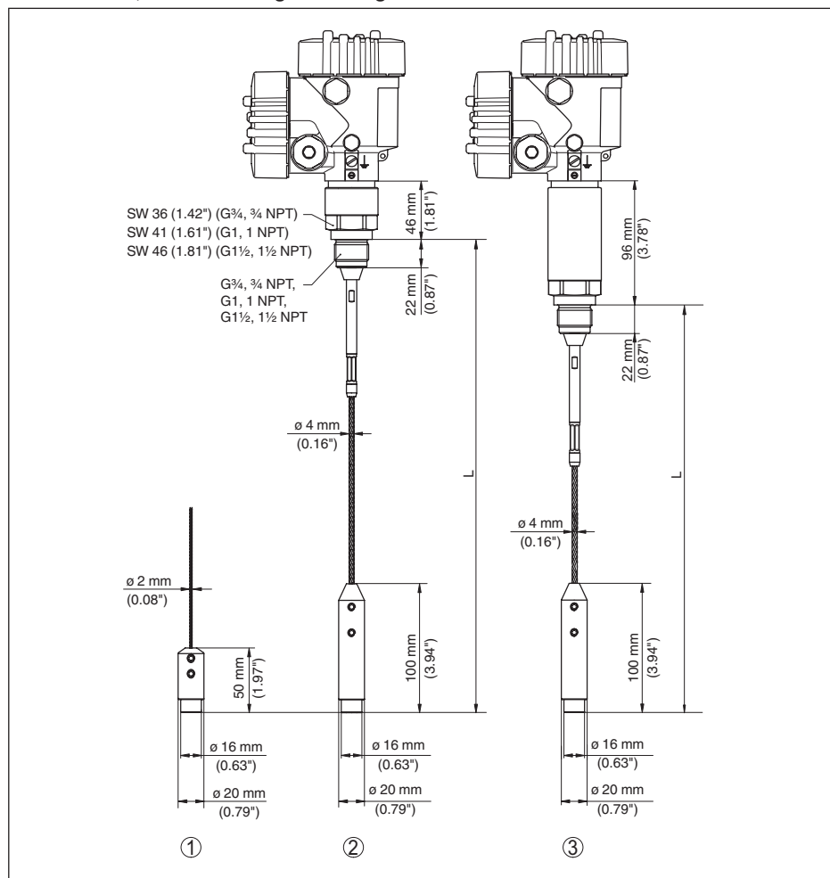
Abb. 41: VEGAFLEX 81, Gewindeausführung mit Straffgewicht (alle Straffgewichte mit Gewinde M8 für Ringschraube)
