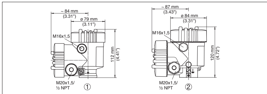
Abb. 40: Maße Gehäuse (mit eingebautem Anzeige- und Bedienmodul vergrößert sich die Gehäusehöhe um 9 mm/0.35 in)
