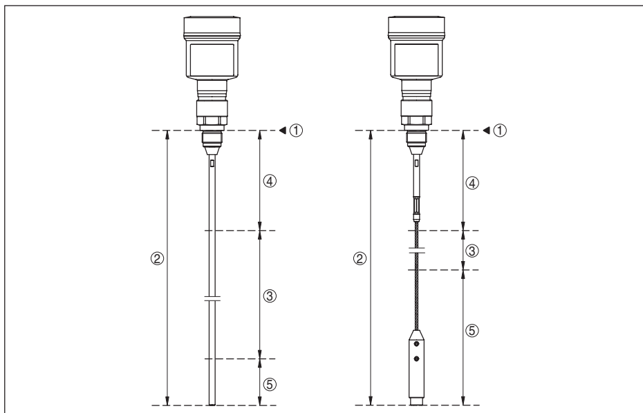
Abb. 30: Messbereiche - VEGAFLEX 81
