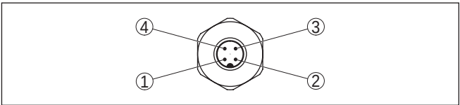
Abb. 18: Sicht auf den M12 x 1-Steckverbinder
