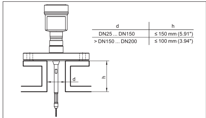
Abb. 6: Montagestutzen
