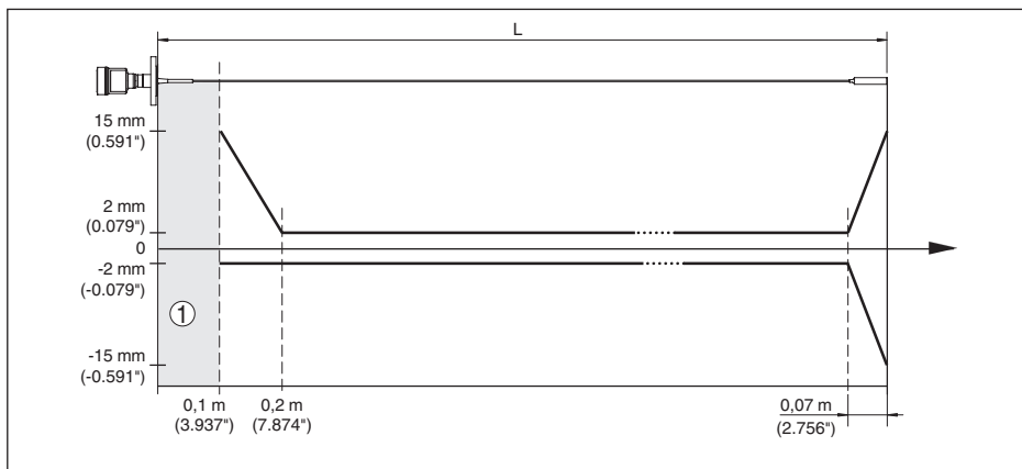
Abb. 36: Messabweichung VEGAFLEX 81 in Seilausführung (ø 4 mm/0.157 in, PFA-beschichtet) in Medium Wasser
