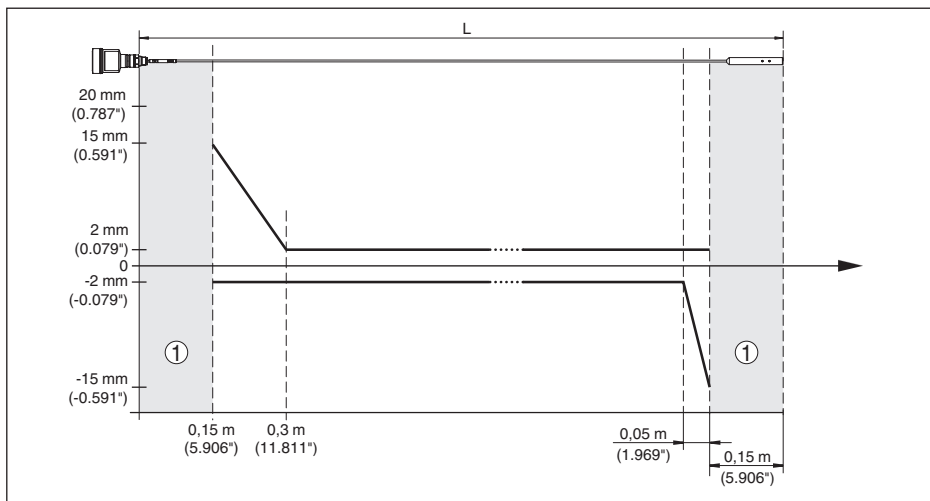
Abb. 35: Messabweichung VEGAFLEX 81 in Seilausführung (ø 4 mm/0.157 in), in Medium Öl
