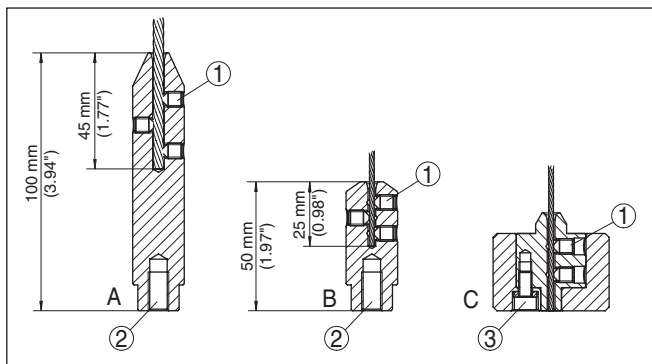
Abb. 29: Seilmesssonde kürzen
