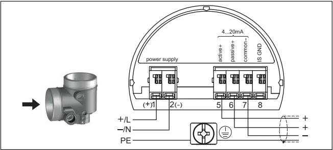
Abb. 15: Anschlussraum Zweikammergehäuse bei Netzspannung
