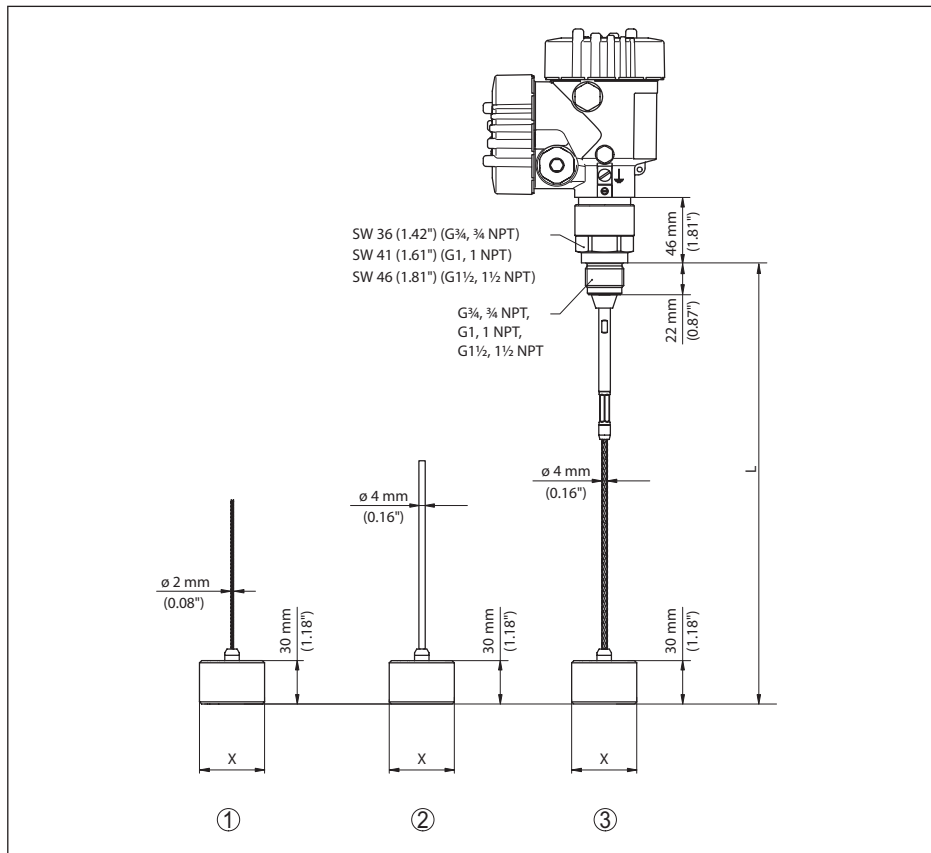
Abb. 42: VEGAFLEX 81, Gewindeausführung
