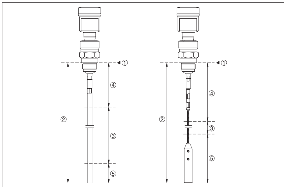
Fig. 32: Faixas de medição - VEGAFLEX 82
