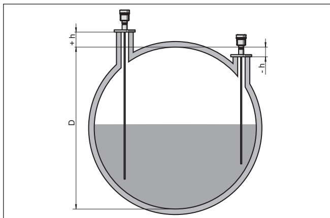
Fig. 17: Altura do reservatório e valor de correção da luva
