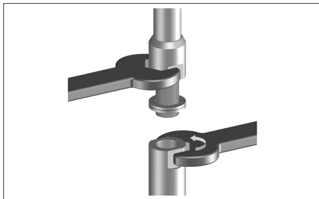
Fig. 26: Trocar o cabo ou a haste de medição
