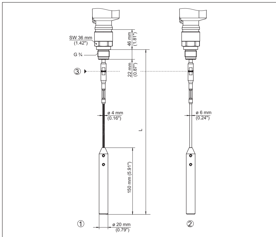
Fig. 38: VEGAFLEX 82, cabo de aço \varnothing 4 mm (0.157 in), \varnothing 6 mm (0.236 in) modelo com rosca com peso tensor (todos os pesos tensores com rosca M12 para olhal)
