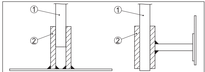
Fig. 7: Fixar a sonda de medição
