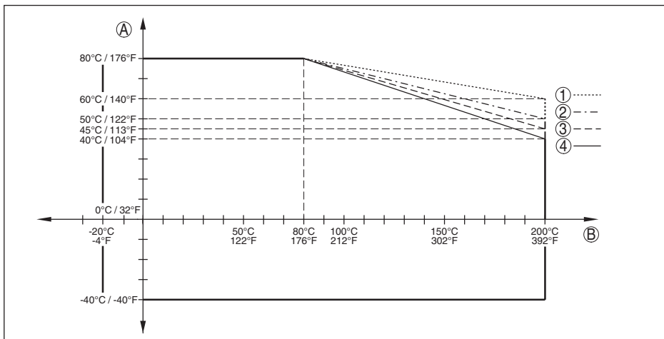
Fig. 36: Temperatura ambiente - Temperatura do processo, modelo com adaptador de temperatura
