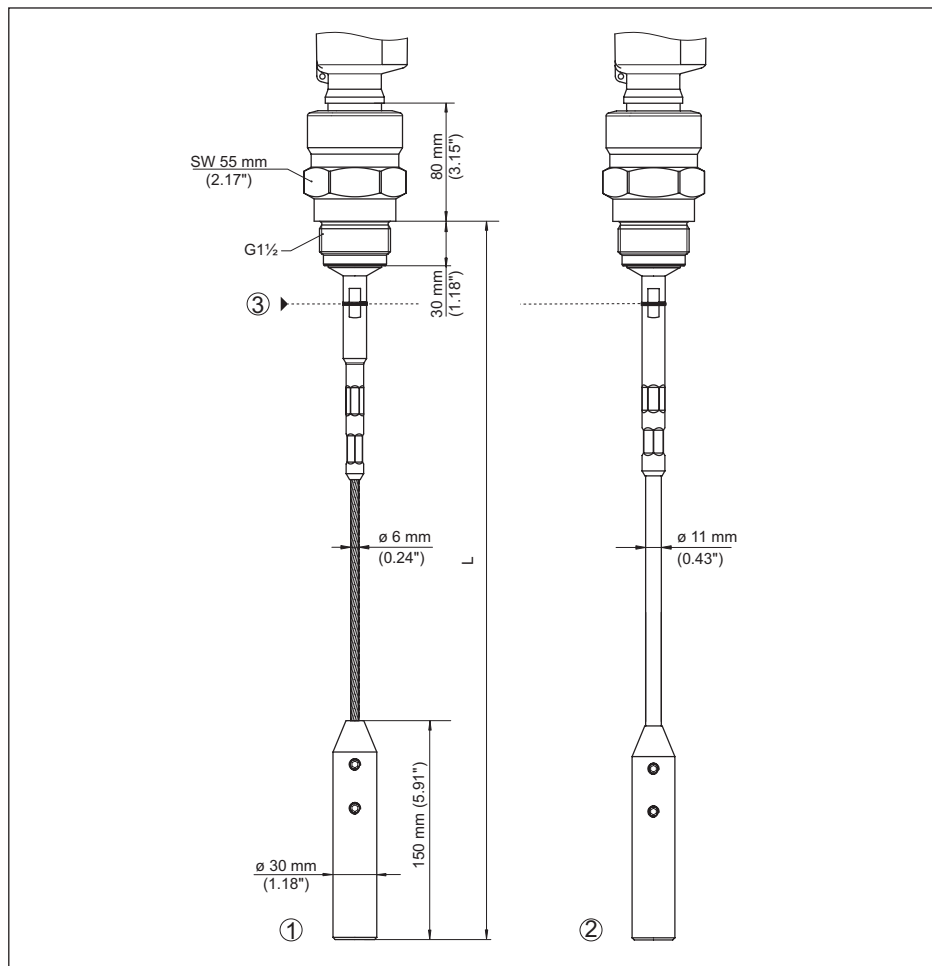
Fig. 39: VEGAFLEX 82, cabo de aço \varnothing 6 mm (0.236 in), \varnothing 11 mm (0.433 in) modelo com rosca com peso tensor (todos os pesos tensores com rosca M12 para olhal)
