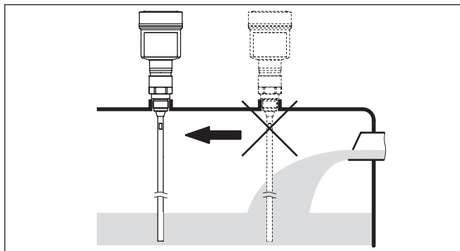
Fig. 6: Montagem do sensor no fluxo de entrada do produto
