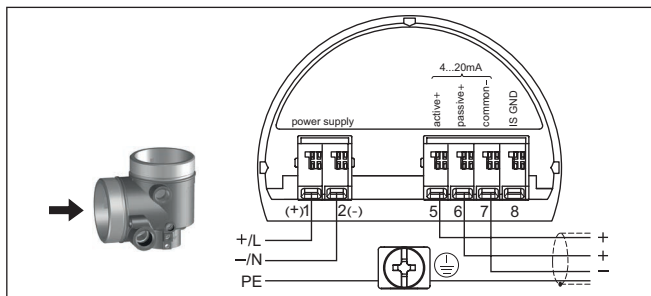
Fig. 10: Compartimento de conexão da caixa e duas câmaras para tensão da rede
