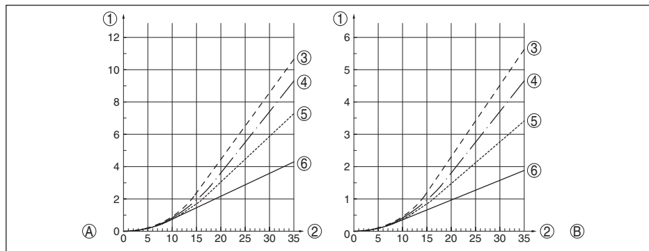
Fig. 28: Tração máxima no caso de cereais e granulado de plástico - Cabo de aço: \varnothing 4 mm (0.157 in)
