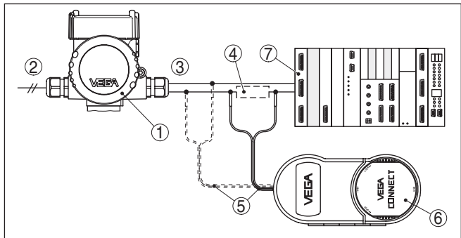
Fig. 21: Conexão do PC à linha de sinais via HART
