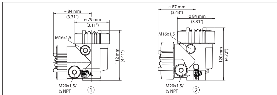
Fig. 37: VEGAFLEX 82 com o módulo de visualização e configuração, a altura da caixa é aumentada em 9 mm (0.35 in)
