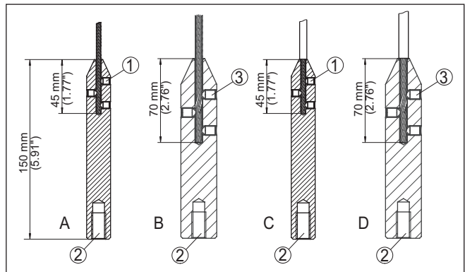
Fig. 27: Encurtar a sonda de medição com cabo
