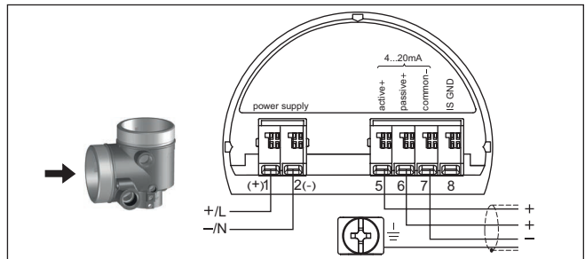
Fig. 11: Compartimento de conexão da caixa e duas câmaras para baixa tensão
