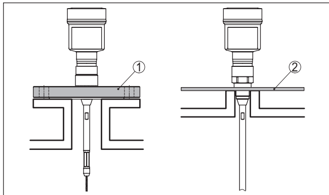
Fig. 2: Montagem em reservatório não metálico
