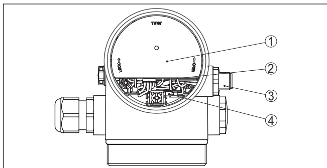
Fig. 12: Vista do compartimento do sistema eletrônico com adaptador do VEGADIS para a conexão da unidade externa de visualização e configuração
