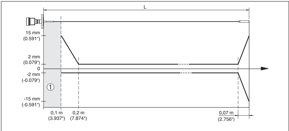
Abb. 36: Messabweichung VEGAFLEX 83 in Seilausführung (beschichtet) in Medium Wasser
