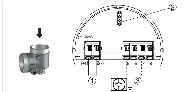
Abb. 14: Elektronikraum - Ex d ia-Zweikammergehäuse
