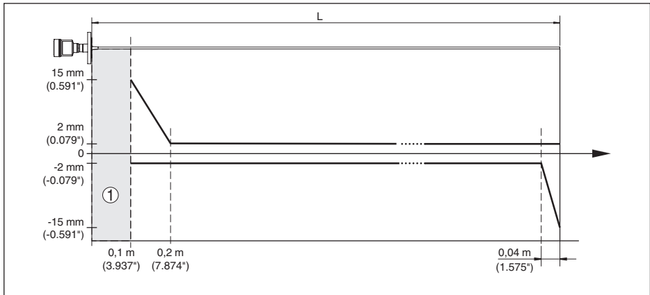
Abb. 34: Messabweichung VEGAFLEX 83 in Stabausführung (beschichtet) in Medium Wasser
