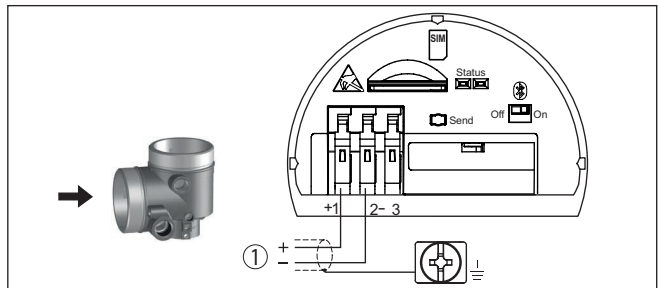
Abb. 13: Anschlussraum - Funkmodul PLICSMOBILE 81
