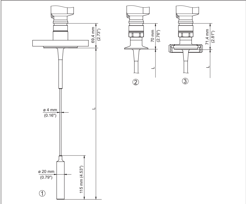
Abb. 44: VEGAFLEX 83, Seilausführung mit Straffgewicht
