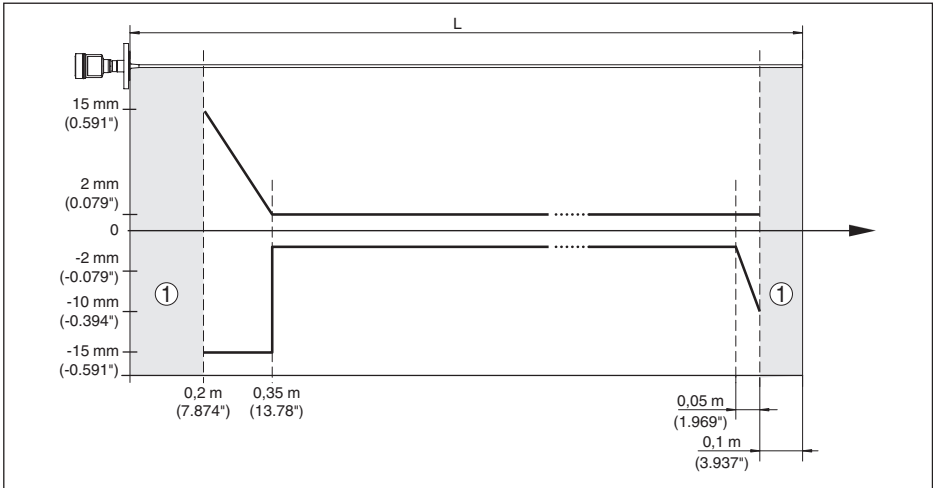
Abb. 35: Messabweichung VEGAFLEX 83 in Stabausführung (beschichtet) in Medium Öl
