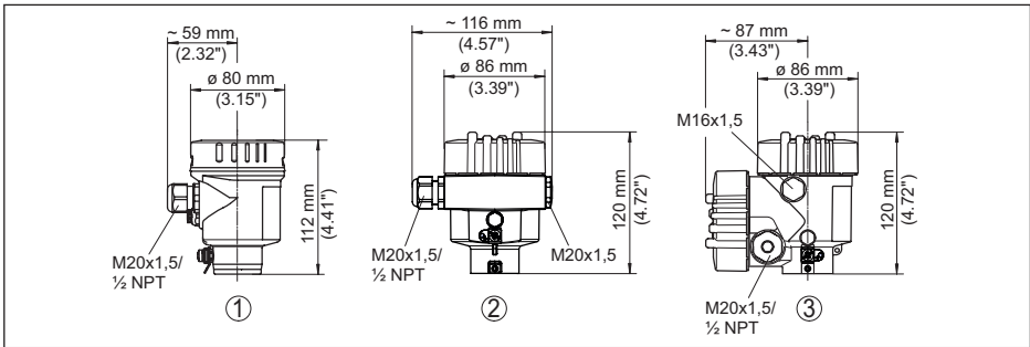
Abb. 42: Gehäuseausführungen in Schutzart IP66/IP68 (0,2 bar), (mit eingebautem Anzeige- und Bedienmodul vergrößert sich die Gehäusehöhe um 18 mm/0.71 in)
