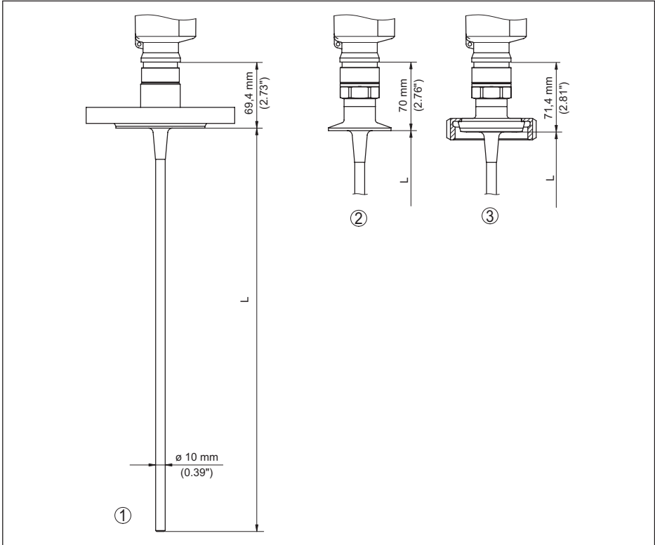
Abb. 45: VEGAFLEX 83, Stabausführung
