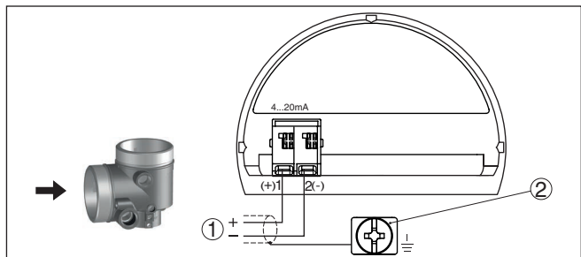
Abb. 15: Anschlussraum - Ex d ia-Zweikammergehäuse
