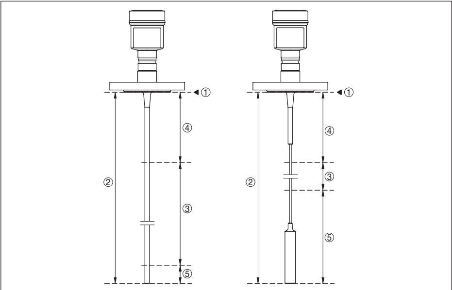
Abb. 33: Messbereiche - VEGAFLEX 83
