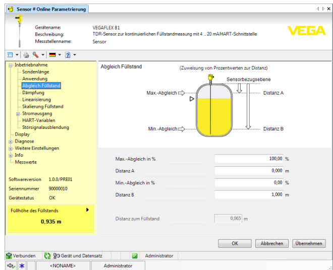
Abb. 27: Beispiel einer DTM-Ansicht
