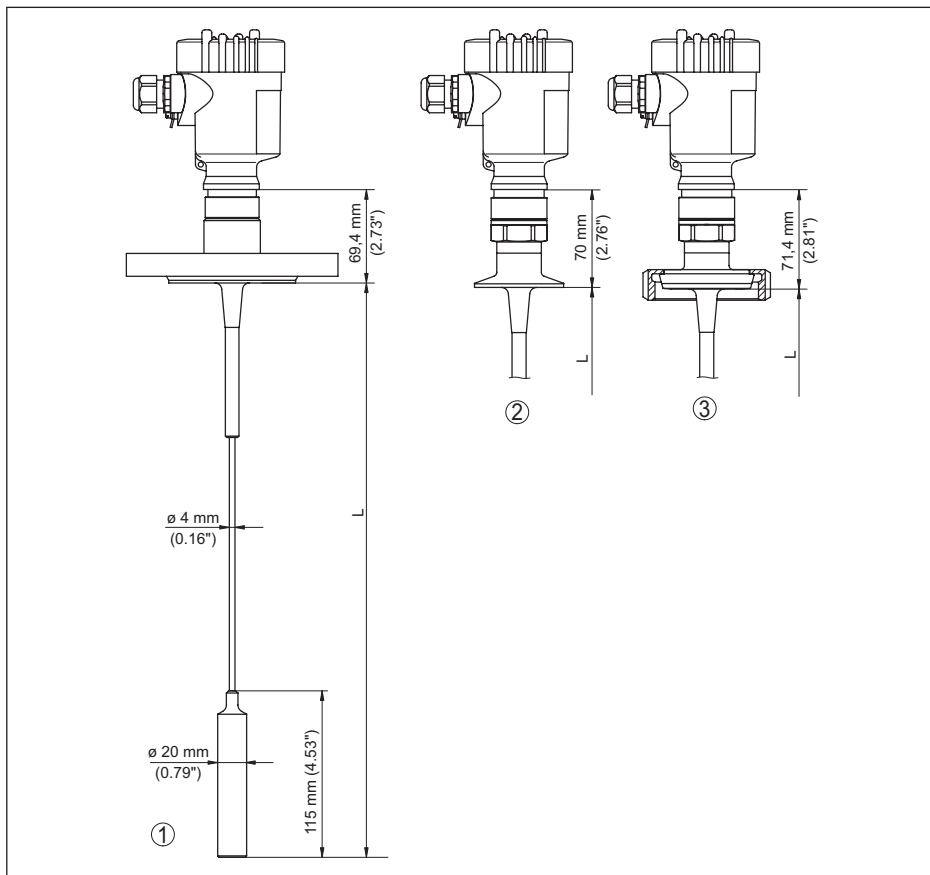
Abb. 42: VEGAFLEX 83, Seilausführung mit Straffgewicht
