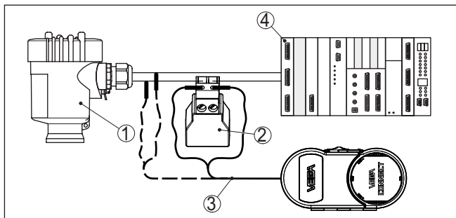
Abb. 26: Anschluss des PCs via HART an die Signalleitung
