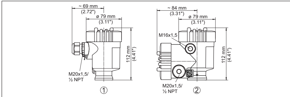
Abb. 37: Gehäuseausführungen in Schutzart IP66/IP67 (mit eingebautem Anzeige- und Bedienmodul vergrößert sich die Gehäusehöhe um 9 mm/0.35 in)
