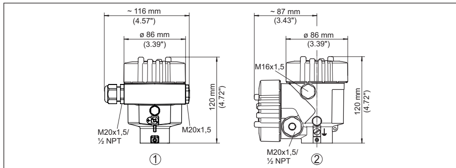
Abb. 38: Gehäuseausführungen in Schutzart IP66/IP68 (0,2 bar), (mit eingebautem Anzeige- und Bedienmodul vergrößert sich die Gehäusehöhe um 9 mm/0.35 in)
