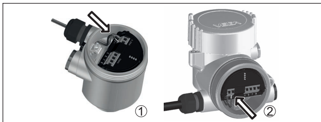
Abb. 10: Anschlusschritte 5 und 6
