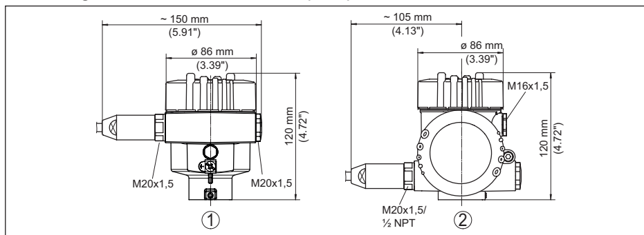
Abb. 39: Gehäuseausführungen in Schutzart IP66/IP68 (1 bar), (mit eingebautem Anzeige- und Bedienmodul vergrößert sich die Gehäusehöhe um 9 mm/0.35 in)
