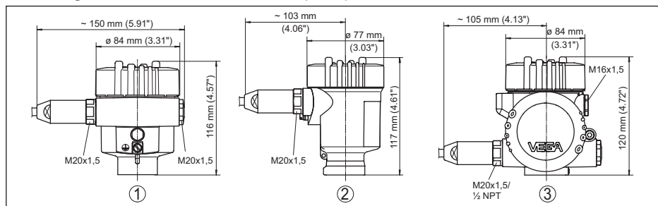
Abb. 41: Gehäuseausführungen in Schutzart IP66/IP68 (1 bar), (mit eingebautem Anzeige- und Bedienmodul vergrößert sich die Gehäusehöhe um 9 mm/0.35 in)
