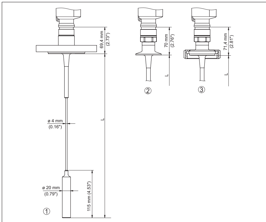
Fig. 44: VEGAFLEX 83, version câble avec poids tenseur
