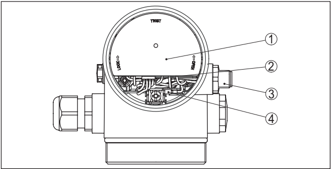
Fig. 16: Vue sur le compartiment de l'électronique avec l'adaptateur VEGADIS pour le raccordement de l'unité de réglage et d'affichage
