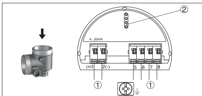
Fig. 11: Compartiment électronique - boîtier à deux chambres
