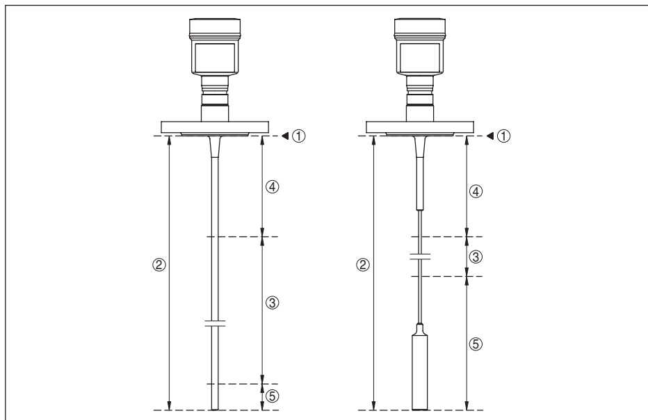
Fig. 33: Plages de mesure - VEGAFLEX 83
