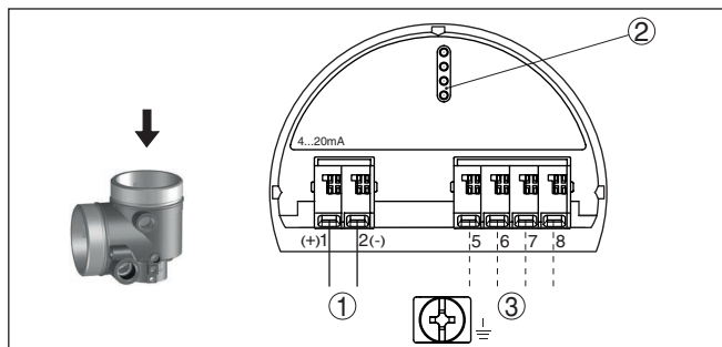
Fig. 14: Compartiment électronique - boîtier à deux chambres Ex d ia
