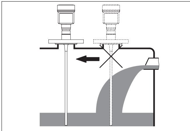
Fig. 7: Montage du capteur en présence d'un flux de produit
