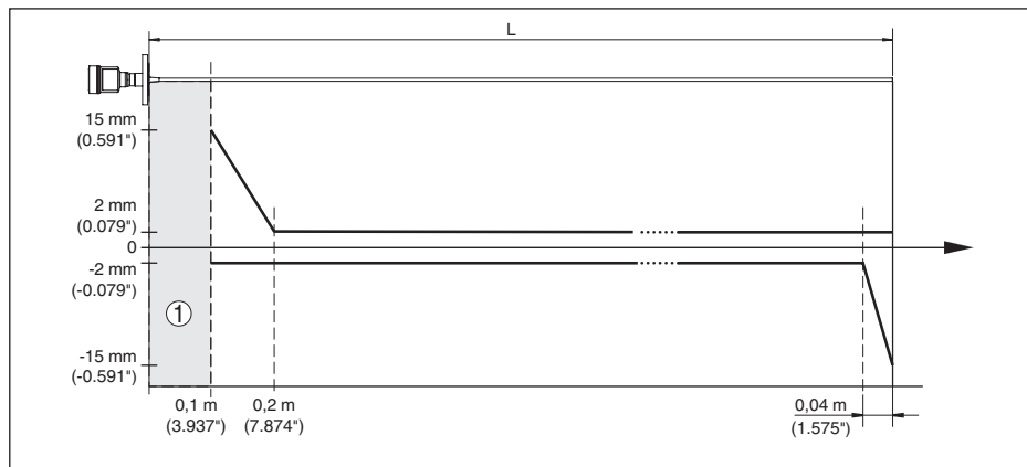
Fig. 34: Écart de mesure VEGAFLEX 83 en version tige (revêtue) dans l'eau
