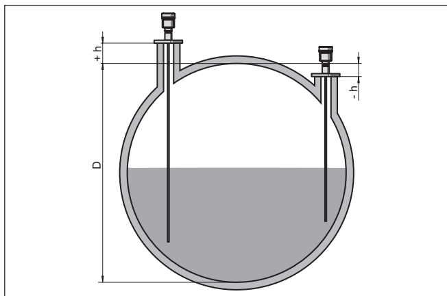
Fig. 24: Hauteur de la cuve et valeur de correction du manchon
