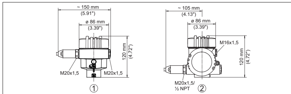
Fig. 41: Variantes de boîtier en protection IP66/IP68 (1 bar), (avec un module de réglage et d'affichage intégré, la hauteur du boîtier augmente de 18 mm/0.71 in)
