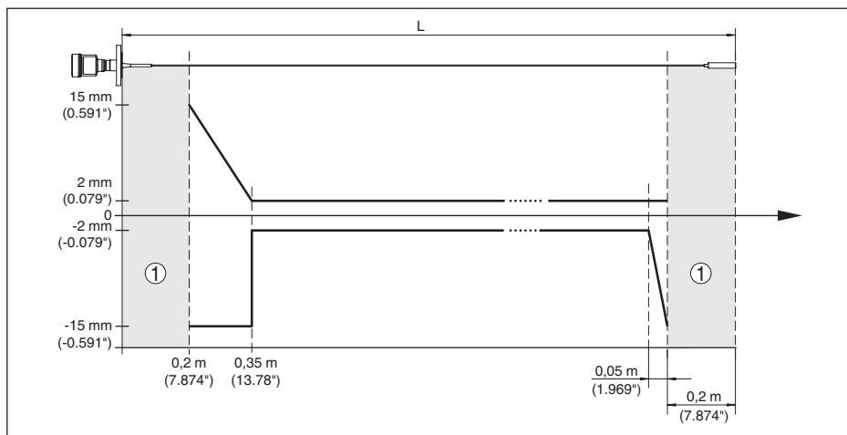
Fig. 37: Écart de mesure VEGAFLEX 83 en version câble (revêtu) dans l'huile
