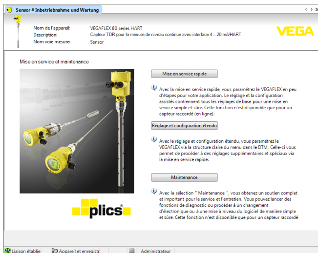
Fig. 30: Sélectionner la mise en marche rapide
