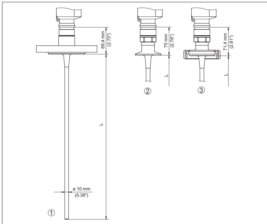
Fig. 45: VEGAFLEX 83, version tige
