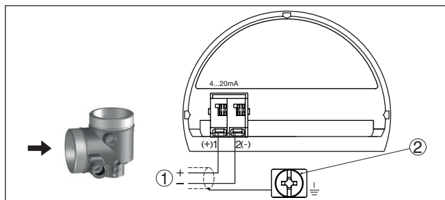
Fig. 15: Compartiment de raccordement - Boîtier à deux chambres Ex d ia
