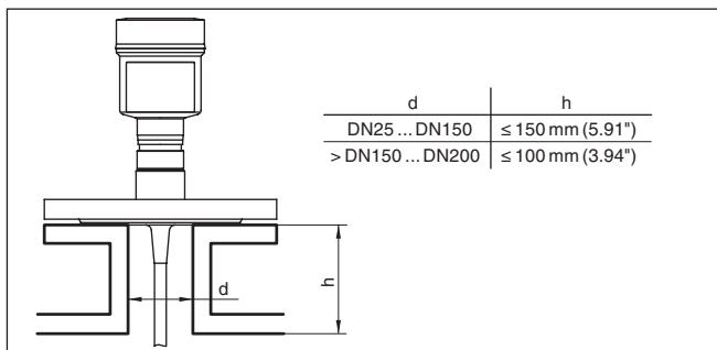
Fig. 5: Rehausse de montage
