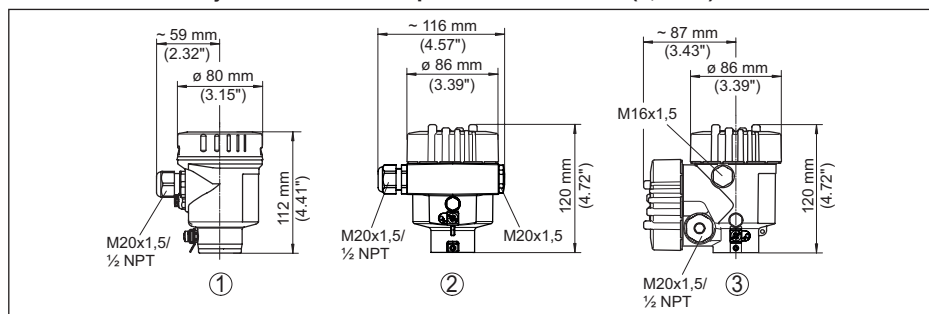
Fig. 42: Variantes de boîtier en protection IP66/IP68 (0,2 bar), (avec un module de réglage et d'affichage intégré, la hauteur du boîtier augmente de 18 mm/0.71 in)
