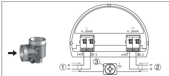
Fig. 19: Compartiment de raccordement boîtier à deux chambres, électronique supplémentaire "sortie courant supplémentaire"
