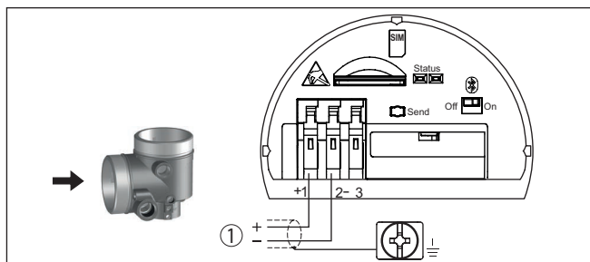
Fig. 13: Compartiment de raccordement - Module radio PLICSMOBILE 81
