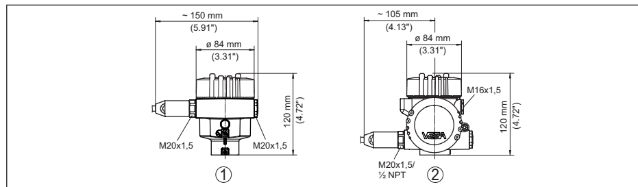
Fig. 43: Variantes de boîtier en protection IP66/IP68 (1 bar), (avec un module de réglage et d'affichage intégré, la hauteur du boîtier augmente de 18 mm/0.71 in)
