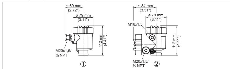
Fig. 39: Variantes de boîtier en protection IP66/IP67 (avec un module de réglage et d'affichage intégré, la hauteur du boîtier augmente de 9 mm/0.35 in)
