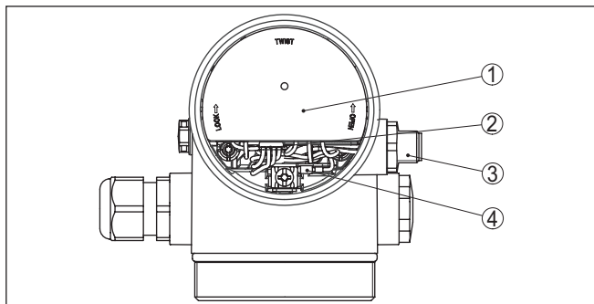
Fig. 17: Een blik op de elektronicarimte met VEGADIS-adapter voor aansluiting van de externe display- en bedieningseenheid
