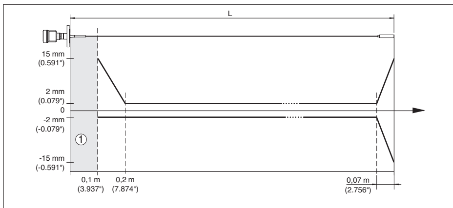
Fig. 37: Meetafwijking VEGAFLEX 83 in kabeluitvoering (bekleed) in product water
