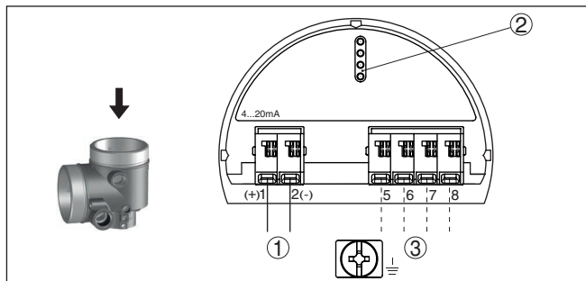
Fig. 15: Elektronicaruimte - Ex d ia-tweekamerbehuizing
