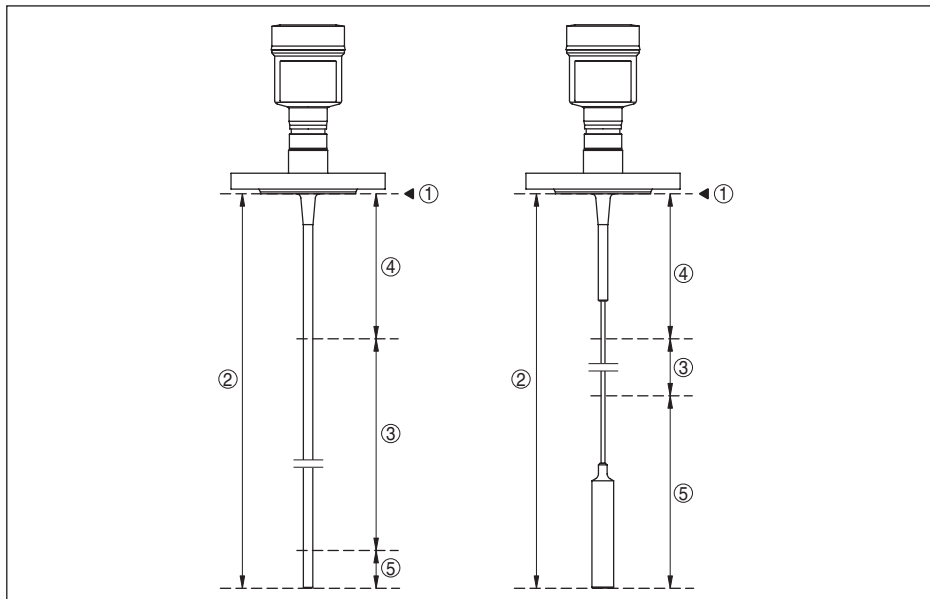
Fig. 34: Meetbereiken - VEGAFLEX 83
