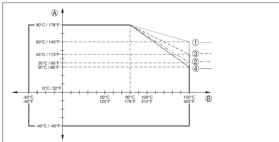
Fig. 39: Omgevingstemperatuur - procestemperatuur standaarduitvoering
