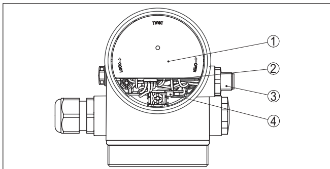
Fig. 17: Een blik op de elektronicaruimte met VEGADIS-adapter voor aansluiting van de externe display- en bedieningseenheid
