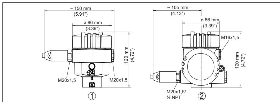
Fig. 39: Huisuitvoeringen in beschermingsklasse IP66/IP68 (1 bar), (met ingebouwde display- en bedieningsmodule wordt het huis 9 mm/0.35 in hoger)
