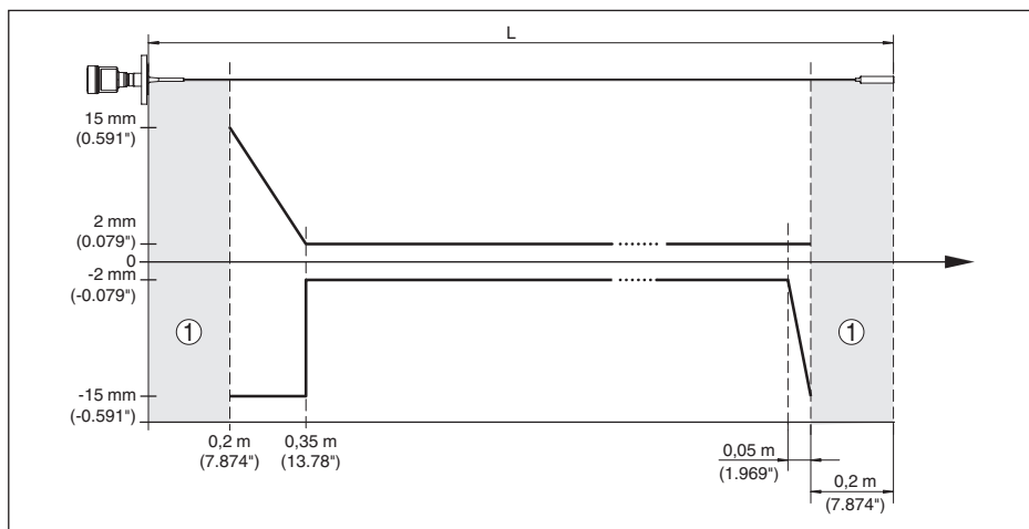
Fig. 35: Meetafwijking VEGAFLEX 83 in kabeluitvoering (bekleed) in product olie
