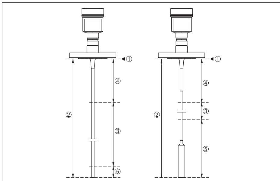
Fig. 31: Meetbereiken - VEGAFLEX 83
