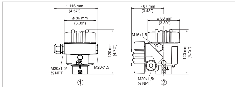
Fig. 38: Huisuitvoeringen in beschermingsklasse IP66/IP68 (0,2 bar), (met ingebouwde display- en bedieningsmodule wordt het huis 9 mm/0.35 in hoger)
