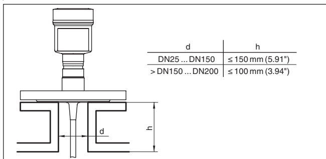
Fig. 6: Montagesok
