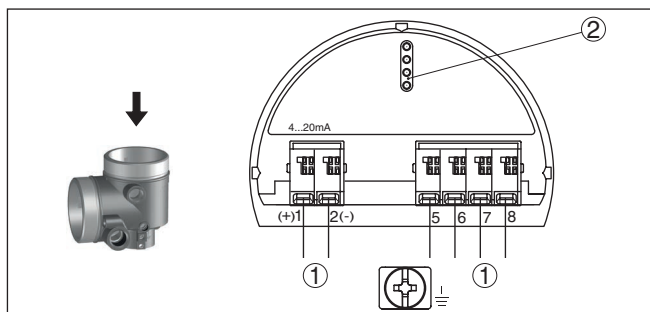
Fig. 12: Elektronicaruimte - tweekamerbehuizing
