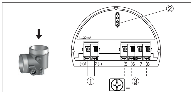
Fig. 15: Elektronicaruimte - Ex-ia-tweekamerbehuizing
