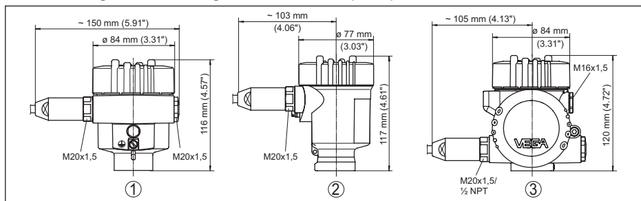
Fig. 41: Huisuitvoeringen in beschermingsklasse IP66/IP68 (1 bar), (met ingebouwde display- en bedieningsmodule wordt het huis 9 mm/0.35 in hoger)
