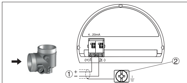
Fig. 16: Aansluitruimte - Ex-d-ia-tweekamerbehuizing
