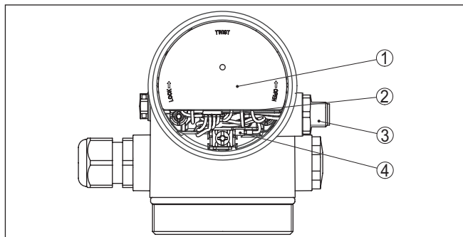
Fig. 14: Een blik op de elektronicarimte met VEGADIS-adapter voor aansluiting van de externe display- en bedieningseenheid
