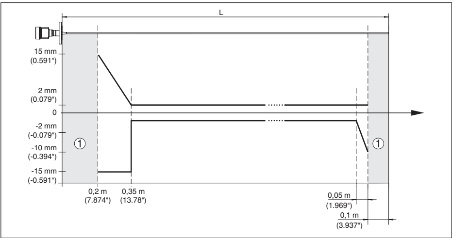
Fig. 30: Meetafwijking VEGAFLEX 83 in staafuitvoering (bekleed) in product olie
