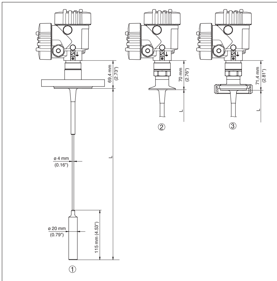
Fig. 35: VEGAFLEX 83, kabeluitvoering met spangewicht
