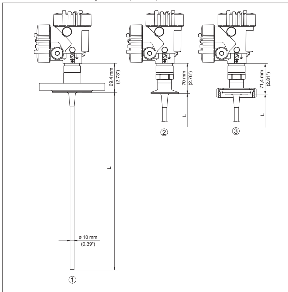
Fig. 36: VEGAFLEX 83, staafuitvoering
