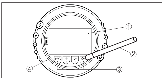
Fig. 18: Display- en bedieningselement - met bediening via magneetpen
