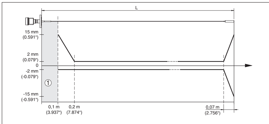
Fig. 31: Meetafwijking VEGAFLEX 83 in kabeluitvoering (bekleed) in product water
