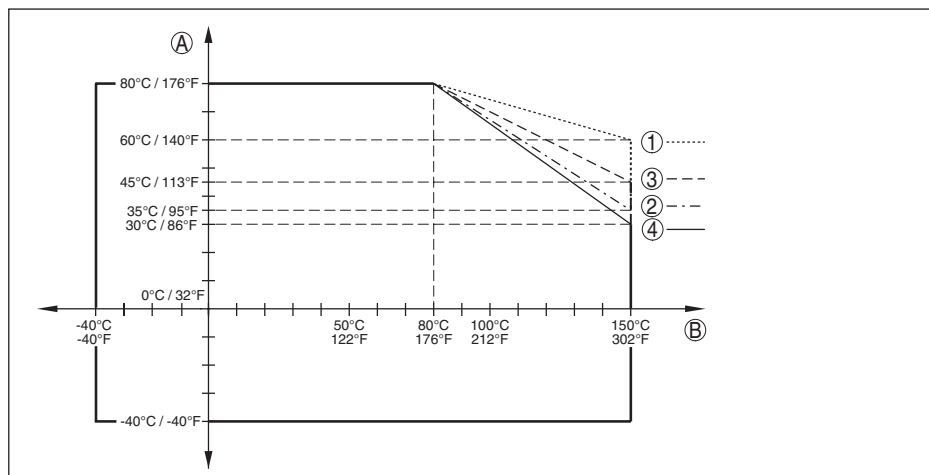
Fig. 33: Omgevingstemperatuur - procestemperatuur standaarduitvoering
