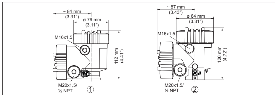
Fig. 34: Afmeting behuizing (met ingebouwde display- en bedieningsmodule wordt de hoogte van de behuizing 9 mm groter)
