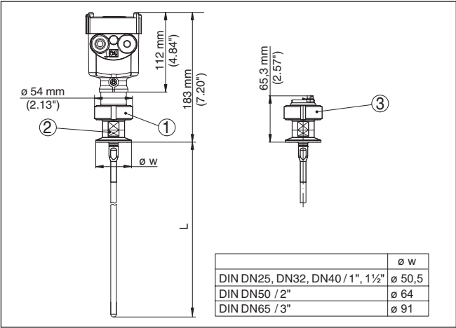
Fig. 10: Autoclaveerbare uitvoering
