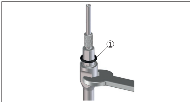
Fig. 30: Meetstaaf vervangen
