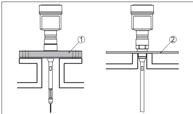
Fig. 6: Montage in niet-metalen tank
