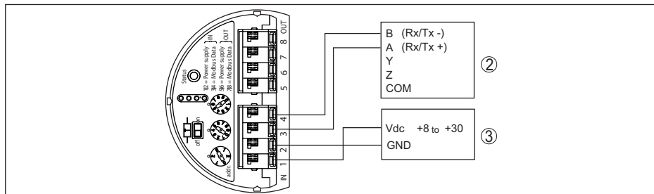
Fig. 37: Aansluiting van de VEGAFLEX 83 op RTU Fisher ROC 809
