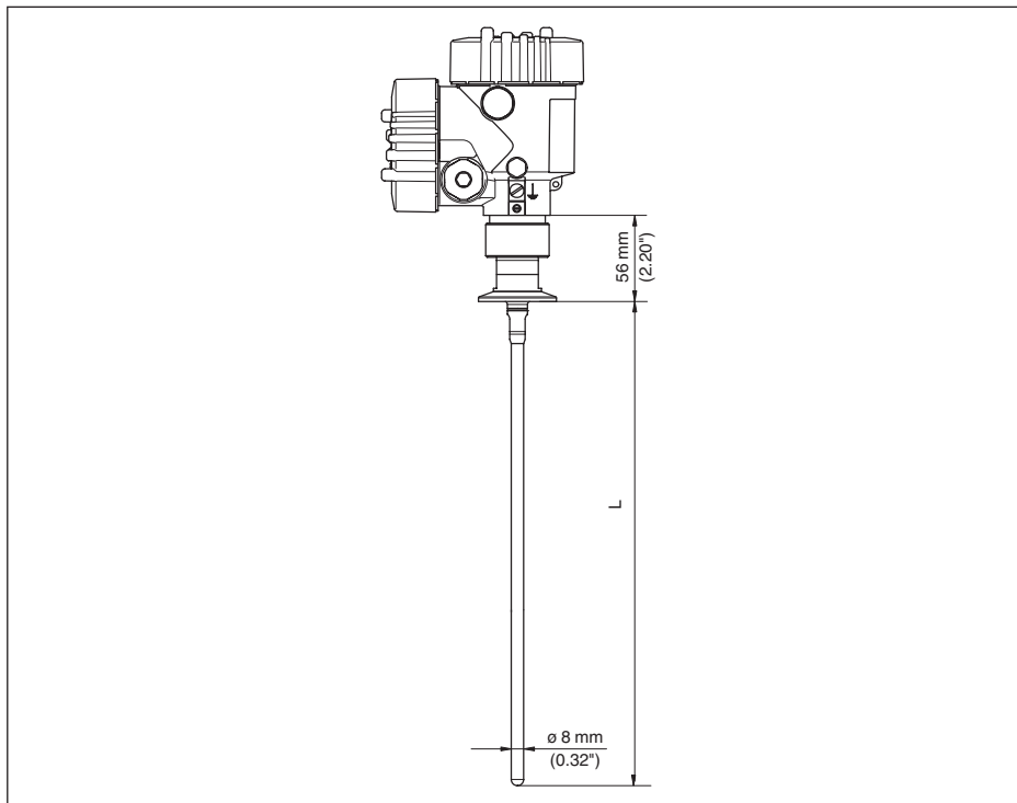
Fig. 39: VEGAFLEX 83, staafuitvoering ø 8 mm (0.315 in), gepolijst
