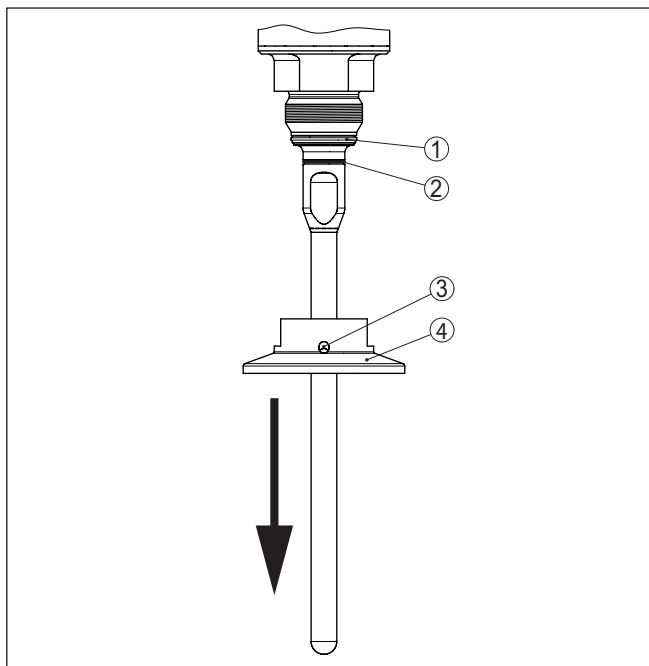
Fig. 32: Afdichting - procesaansluiting
