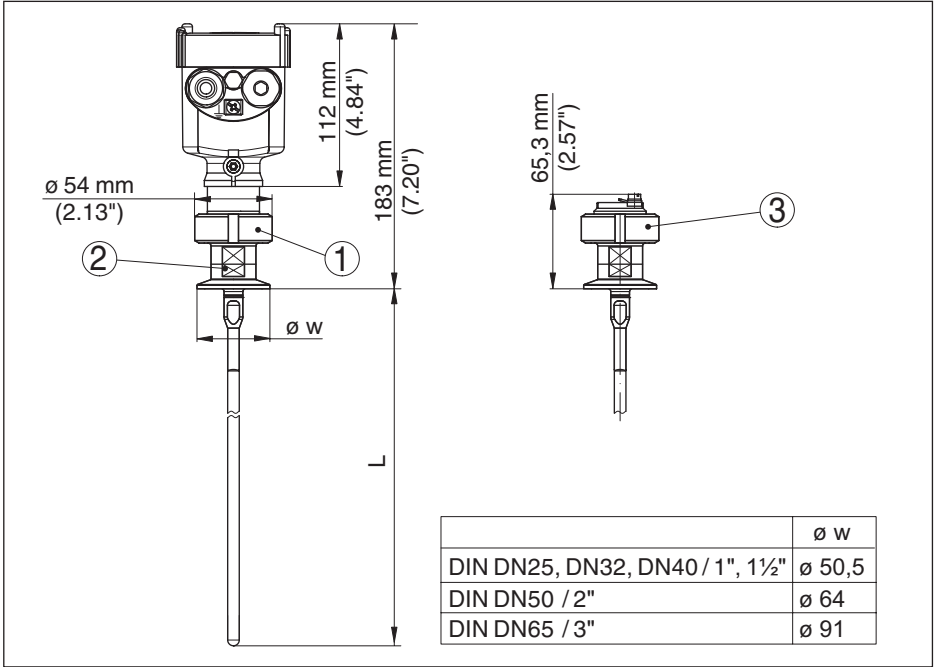
Fig. 40: VEGAFLEX 83, staafruitvoering ø 8 mm (0.315 in), gepolijst - autoclaveerbare uitvoering
