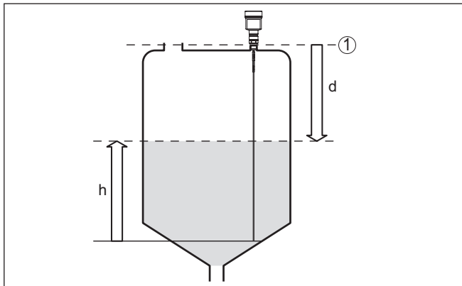
Fig. 3: Niveaumeting
