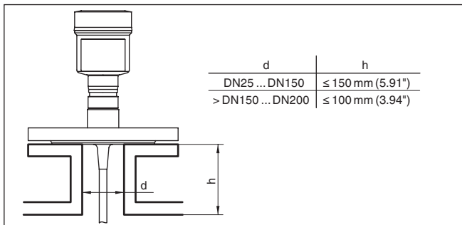
Fig. 7: Montagesok
