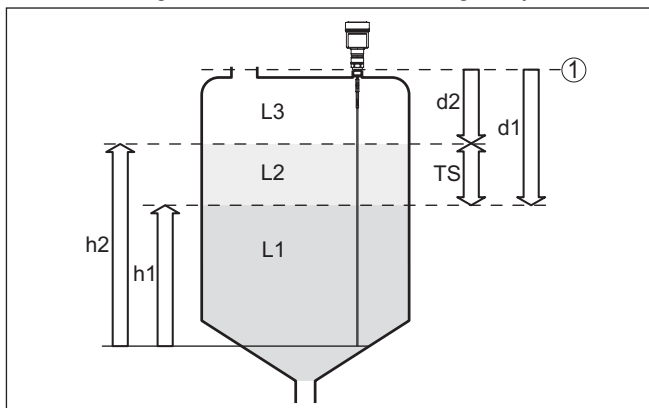
Fig. 4: Scheidingslaagmeting
