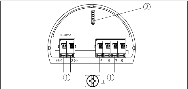
Fig. 13: Elektronicaruimte - tweekamerbehuizing
