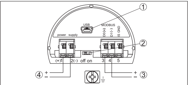
Fig. 14: Aansluitruimte
