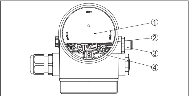
Fig. 15: Een blik op de elektronicarimte met VEGADIS-adapter voor aansluiting van de externe display- en bedieningseenheid
