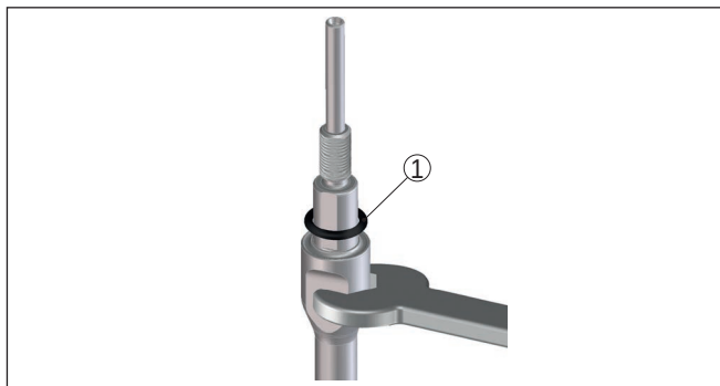
Fig. 31: Meetstaaf demonteren
