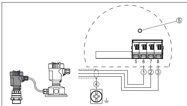
Fig. 24: Aansluiting van de kabel in de sensorbehuizing
