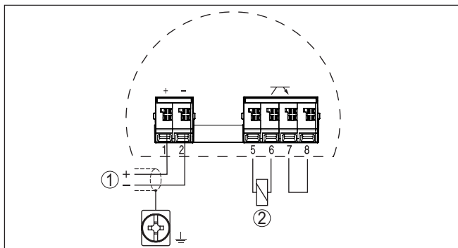
Fig. 27: Aansluitschema meetversterker - VEGAMIP 62 (receiver) - NPN-gedrag
