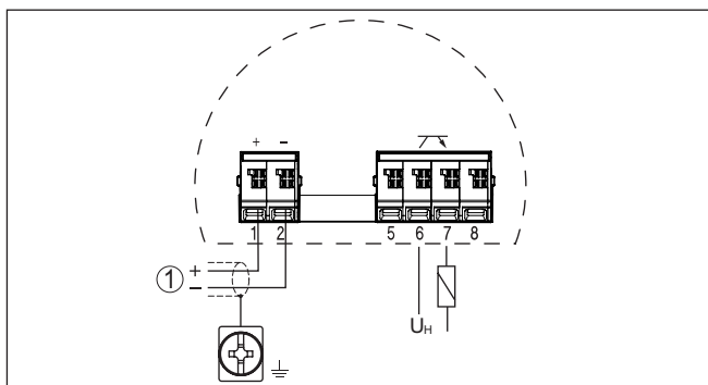
Fig. 28: Aansluitschema meetversterker - VEGAMIP 62 (receiver) - potentiaalvrij
