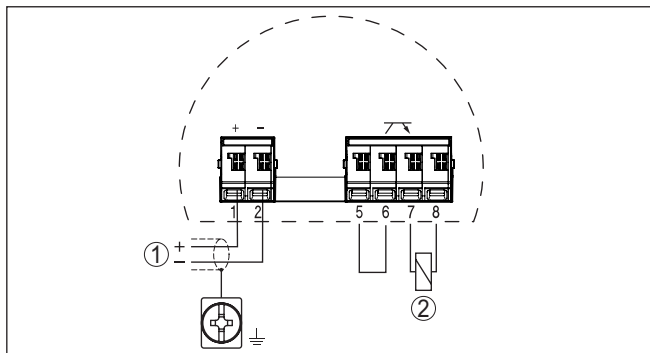
Fig. 26: Aansluitschema meetversterker - VEGAMIP 62 (receiver) - PNP-gedrag
