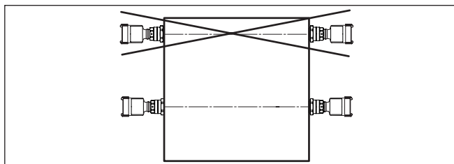
Fig. 6: Inbouwpositie (bovenaanzicht)
