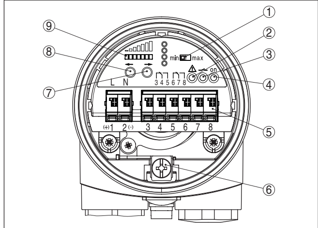
Fig. 27: Módulo eletrônico MP6X R (unidade receptora) - Saída de relé
