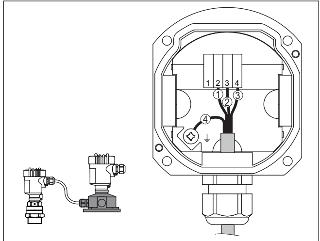
Fig. 23: Conexão do sensor na base da caixa (caixa externa)
