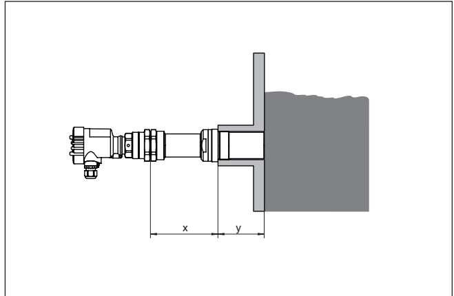
Fig. 15: Adaptador de montagem "alta temperatura com tubo" -40 ... +450 °C (-40 ... +842 °F) para montagem frontal embutida
