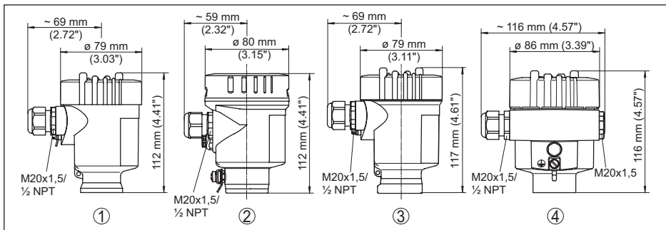
Fig. 32: Modelos da caixa, para caixa do aparelho e caixa externa
