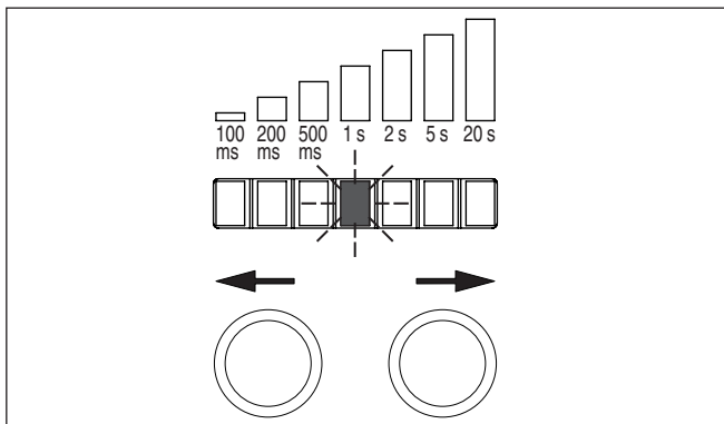
Fig. 31: Ajustar o retardamento de comutação - O LED pisca
