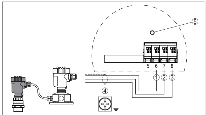
Fig. 24: Conexão do cabo para a caixa externa (unidade de avaliação)
