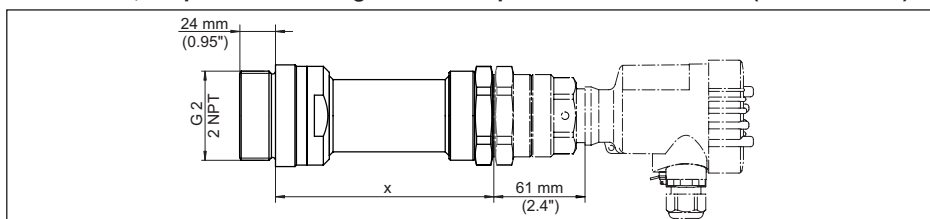
Fig. 38: Adaptador de montagem com cobertura de cerâmica (opcional) para VEGAMIP 62 com antena interna tipo corneta, modelo com rosca G1½ com cobertura de PTFE (também com rosca 1½ NPT)
