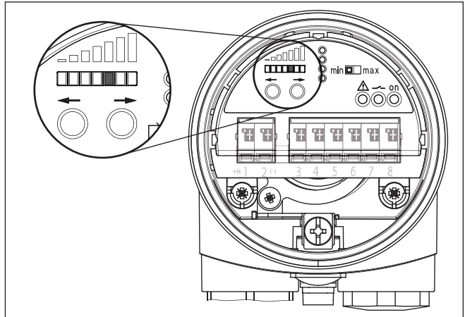
Fig. 30: Barra de LEDs - Ajuste para produtos com baixa capacidade de atenuação do sinal
