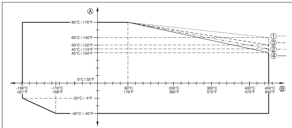
Fig. 36: Omgevingstemperatuur - procestemperatuur standaarduitvoering
