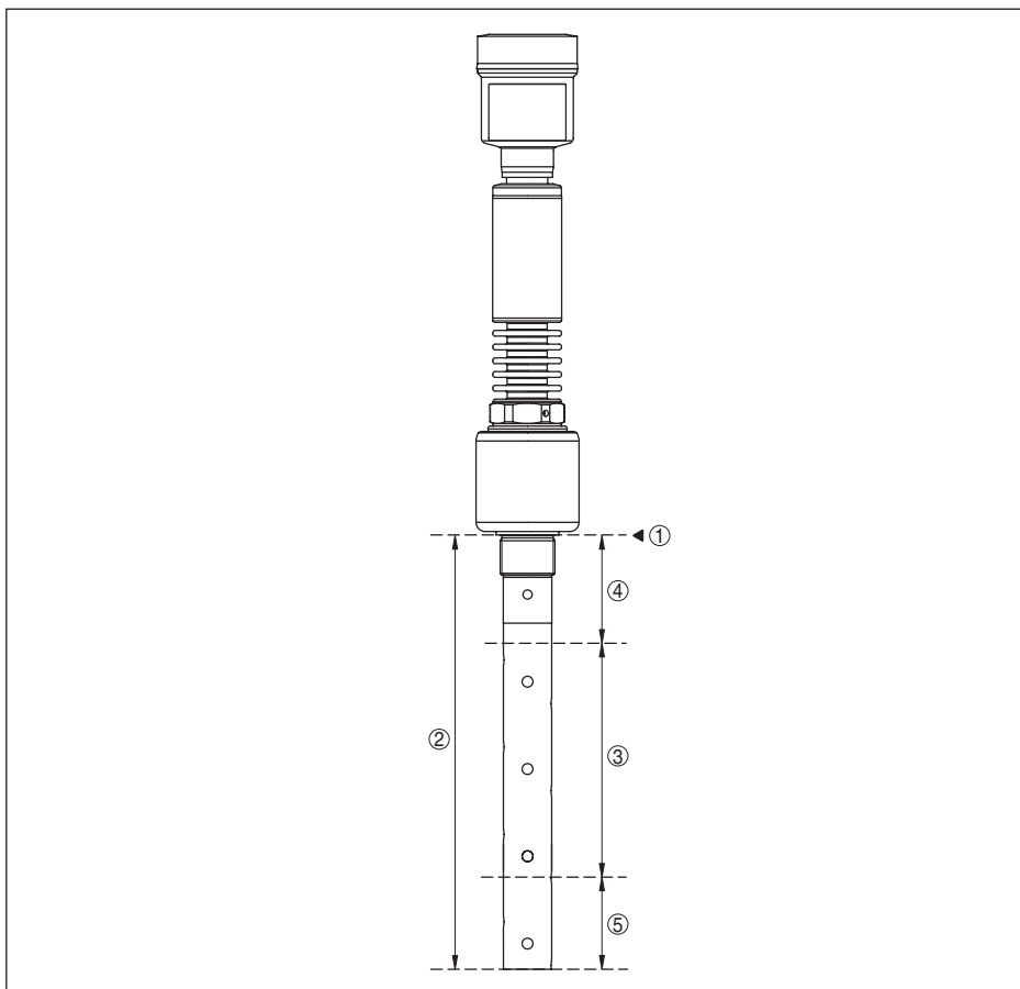
Fig. 30: Meetbereiken - VEGAFLEX 86
