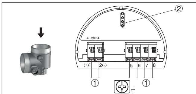
Fig. 11: Elektronicaruimte - tweekamerbehuizing
