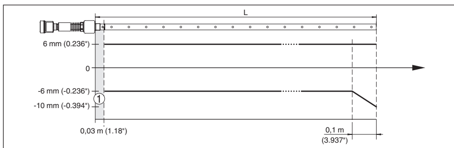
Fig. 32: Meetafwijking VEGAFLEX 86 in coaxuitvoering in product water (meetlengte tot 6 m/19.69 ft)
