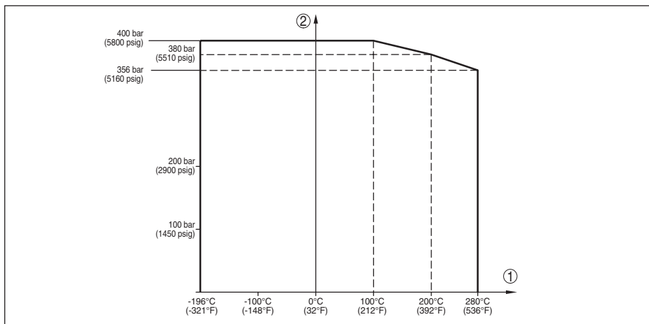
Fig. 37: Procesdruk - procestemperatuur (uitvoering -196 ... +280 °C/-321 ... +536 °F)
