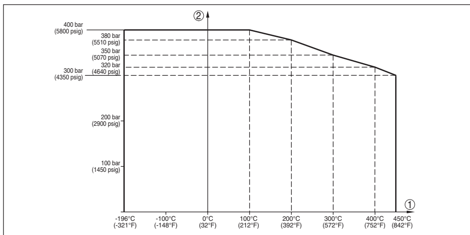
Fig. 38: Procesdruk - procestemperatuur (uitvoering -196 ... +450 °C/-321 ... +842 °F)
