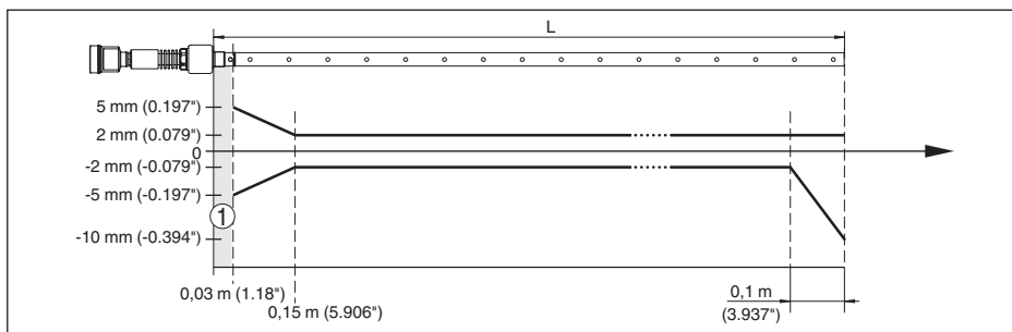
Fig. 31: Meetafwijking VEGAFLEX 86 in coaxuitvoering in product water (meetlengte tot 1,5 m/4.92 ft)
