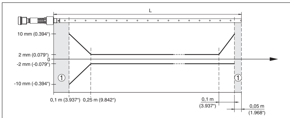
Fig. 33: Meetafwijking VEGAFLEX 86 in coaxuitvoering in product olie (meetlengte tot 1,5 m/4.92 ft)
