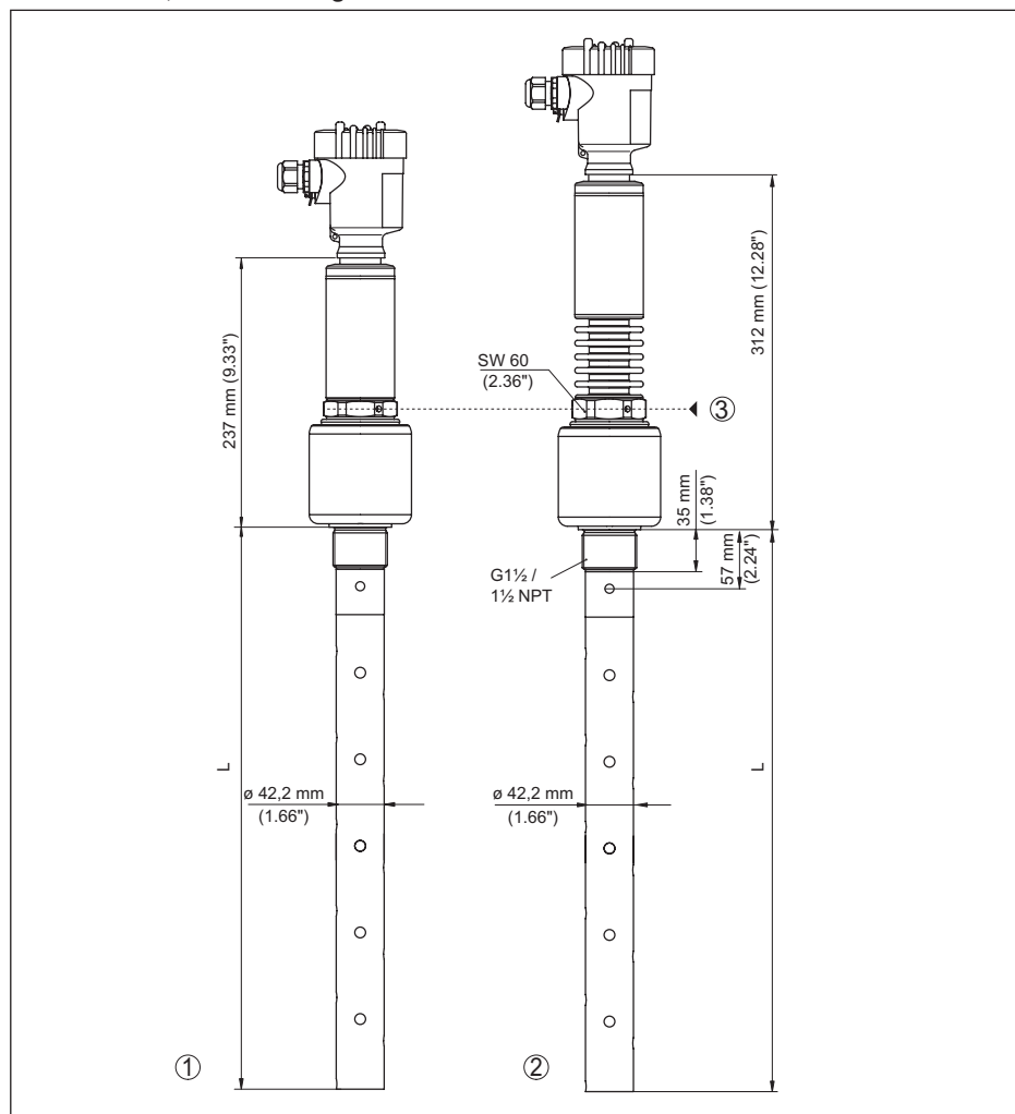
Fig. 44: VEGAFLEX 86, schroefdraaduitvoering
