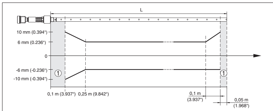
Fig. 34: Meetafwijking VEGAFLEX 86 in coaxuitvoering in medium olie (meetlengte tot 6 m/19.69 ft)
