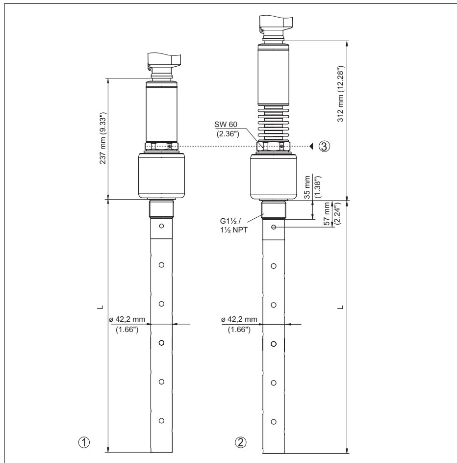
Fig. 37: VEGAFLEX 86, version fileté
