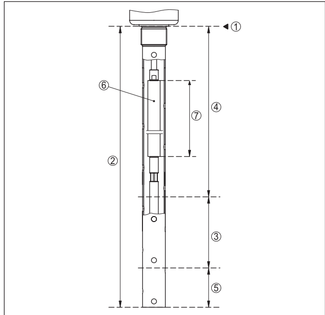
Fig. 31: Plages de mesure - VEGAFLEX 86 avec compensation de la vapeur
