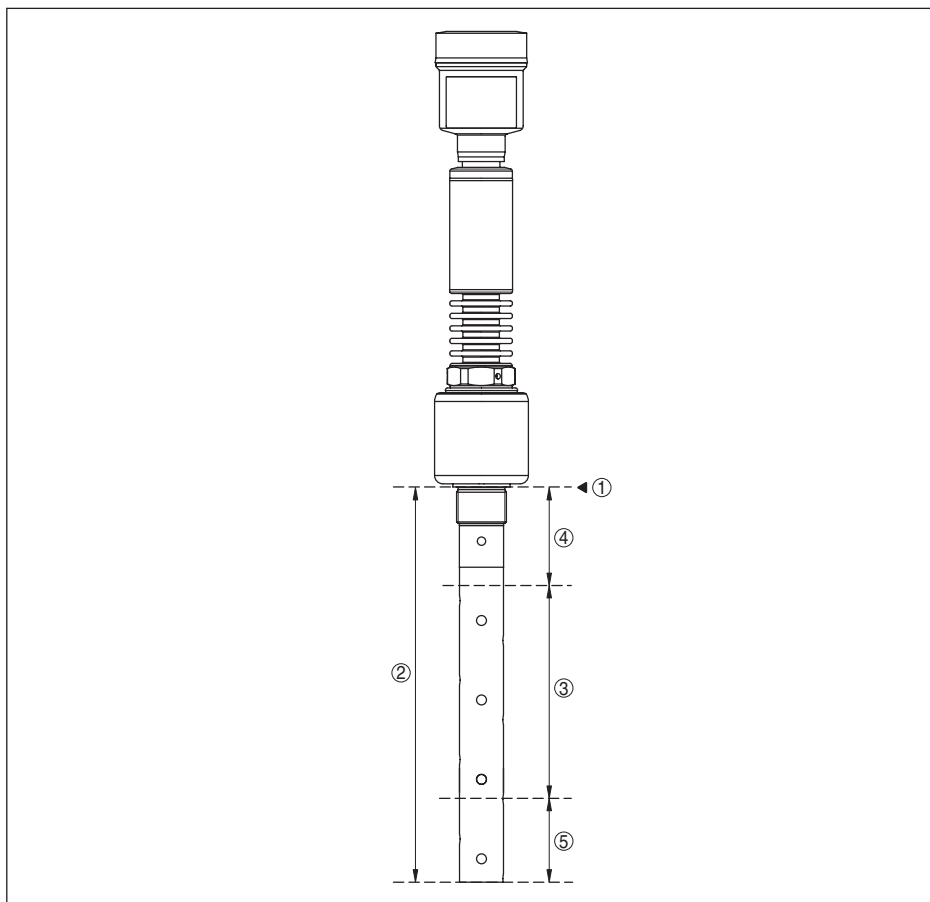
Fig. 26: Plages de mesure - VEGAFLEX 86
