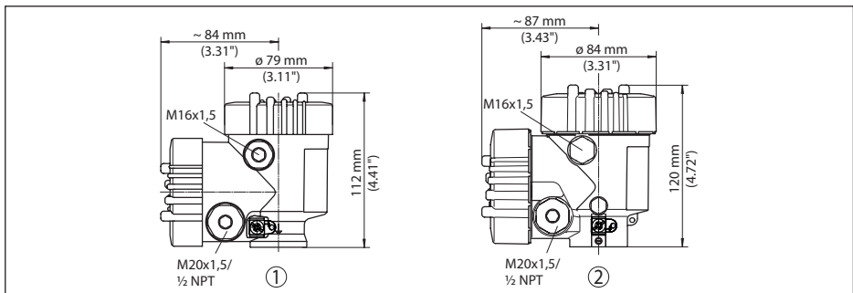
Fig. 36: VEGAFLEX 86 avec module de réglage et d'affichage intégré, la hauteur du boîtier augmente de 9 mm (0.35 in)
