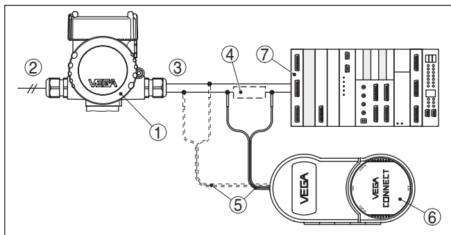
Fig. 21: Raccordement du PC à la ligne signal via HART
