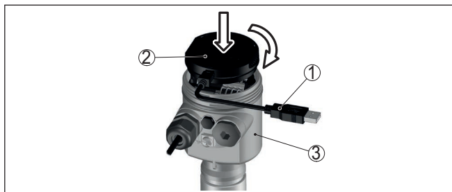
Fig. 20: Raccordement du PC directement au capteur via l'adaptateur d'interfaces
