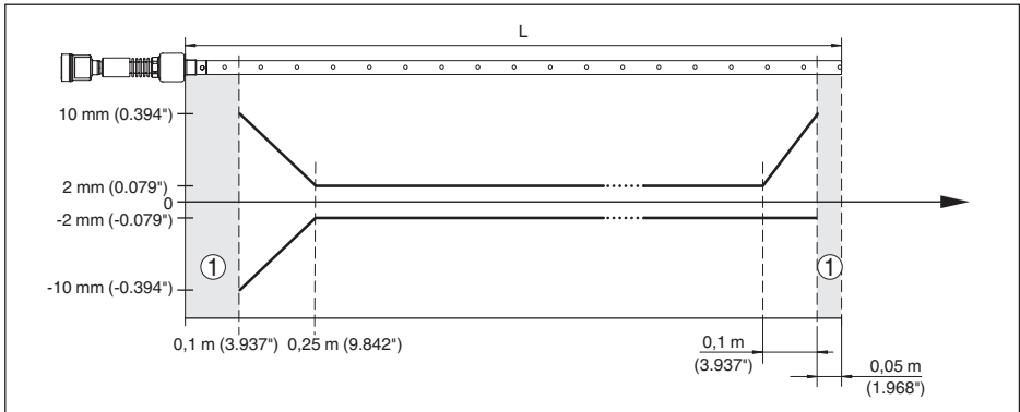
Fig. 29: Écart de mesure VEGAFLEX 86 en version coaxiale dans l'huile (longueur de mesure jusqu'à 1,5 m/4.92 ft)
