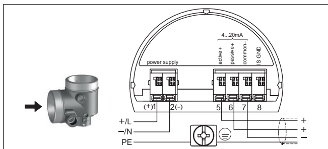
Fig. 10: Compartiment de raccordement boîtier deux chambres pour tension de réseau
