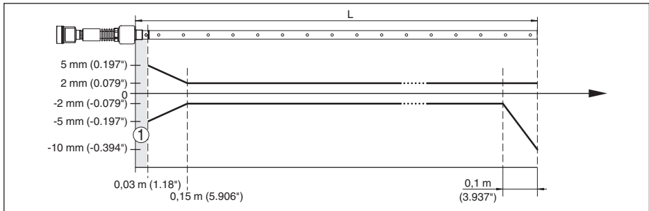
Fig. 27: Écart de mesure VEGAFLEX 86 en version coaxiale dans l'eau (longueur de mesure jusqu'à 1,5 m/4.92 ft)
