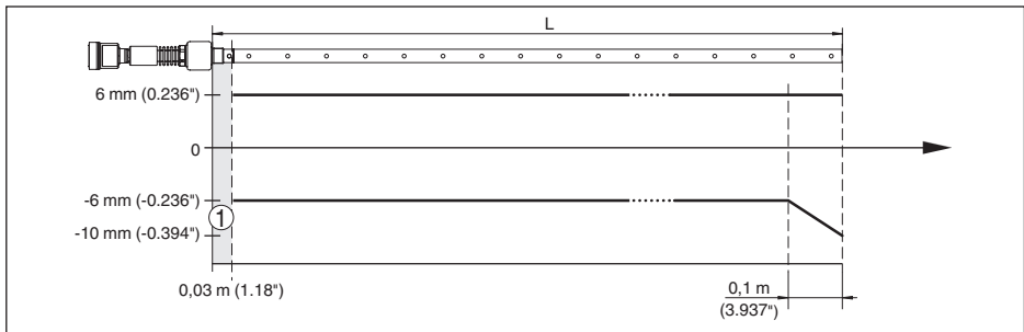
Fig. 28: Écart de mesure VEGAFLEX 86 en version coaxiale dans l'eau (longueur de mesure jusqu'à 6 m/19.69 ft)
