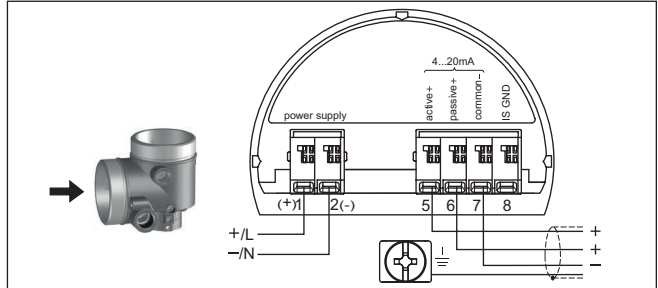
Fig. 11: Compartiment de raccordement boîtier deux chambres pour très basse tension
