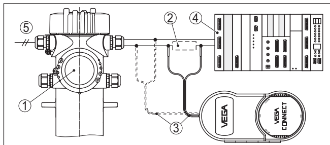
Fig. 21: Aansluiting van de PC via HART op de signaalkabel
