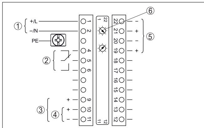
Fig. 8: Elektronica- en aansluitruimte bij niet-Ex instrumenten en instrumenten met niet-intrinsiekveilige stroomuitgang
