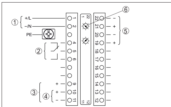
Fig. 12: Elektronica- en aansluitruimte bij niet-Ex instrumenten en instrumenten met niet-intrinsiekveilige stroomuitgang
