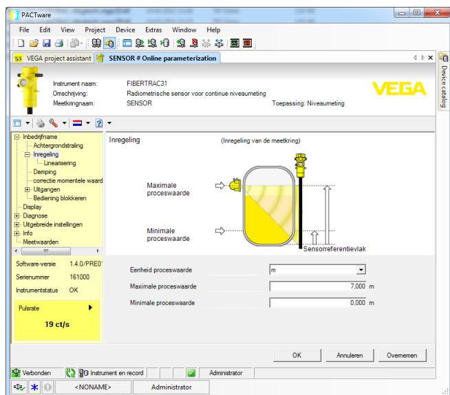
Fig. 22: Voorbeeld van een DTM-aanzicht
