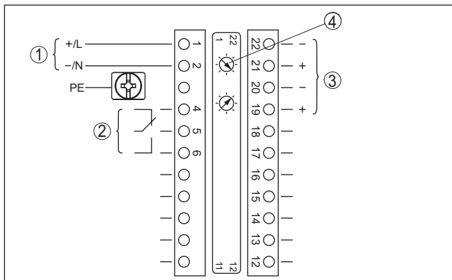
Fig. 10: Elektronica- en aansluitruimte (Ex-d) bij instrumenten met intrinsiekveilige stroomuitgang
